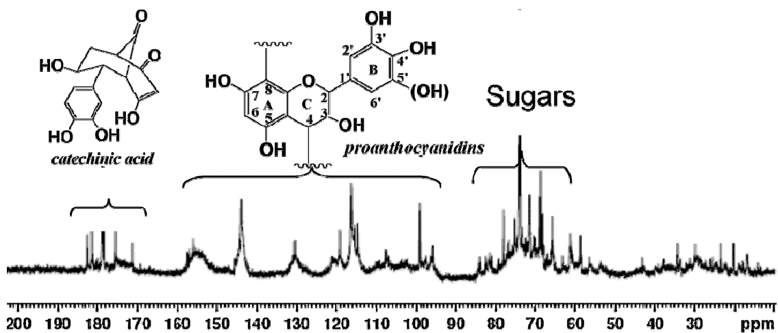
Figure 6. Spectre RMN 13 C d'un extrait de tannin dans D 2 O.
