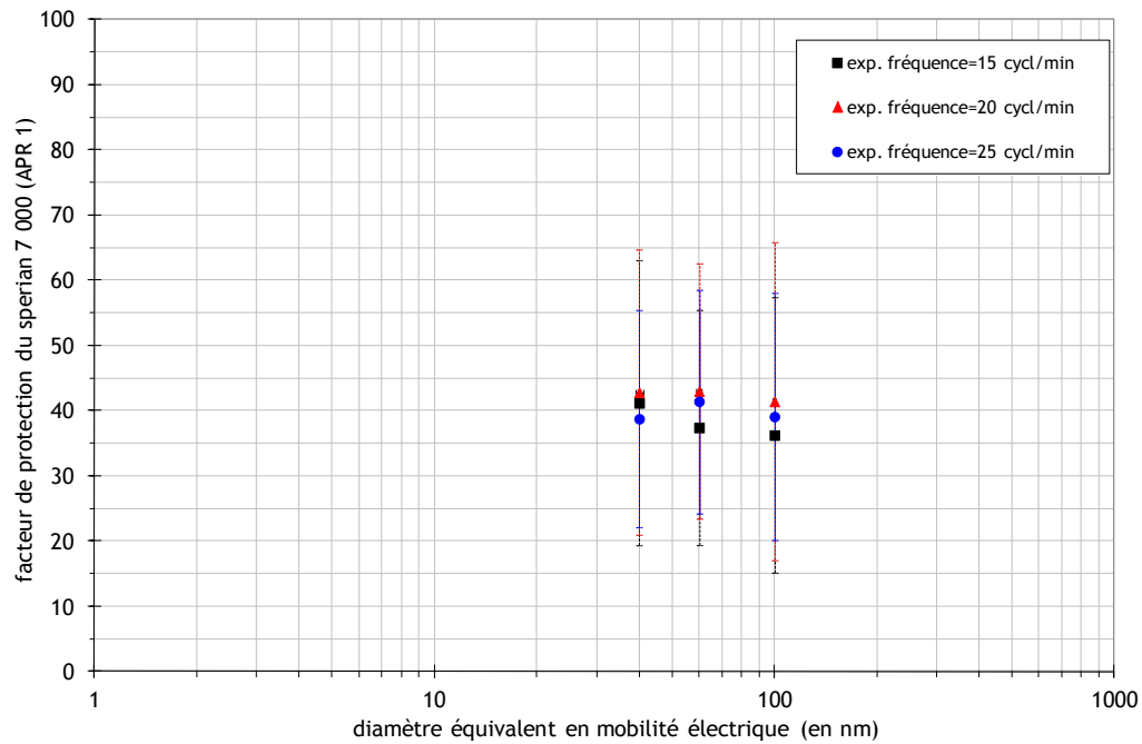
Figure 5-10. Facteurs de protection expérimentaux en présence du tube 3 (de 2,8 mm de diamètre) et pour des débits cycliques d'intensités différentes
