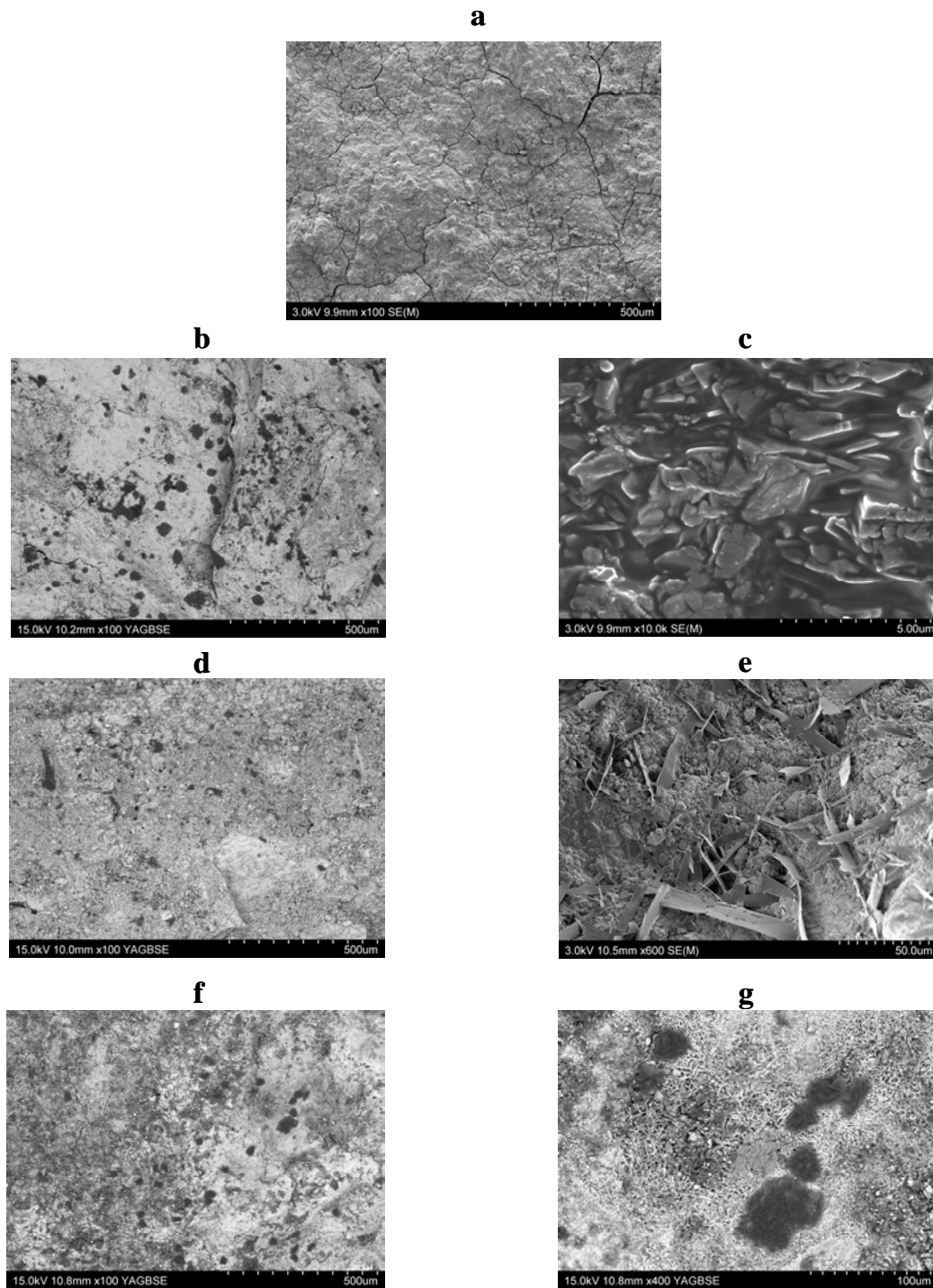
Figure 4.83 : Photographies MEB-mode SE et BSE, sur le faciès de corrosion « maghémite-magnétite », a. non traité, b et c. traité 5 jours dans HC_{10} d et e. traité 5 jours dans NaC_{10} , f et g. traité 5 jours dans la catéchine
