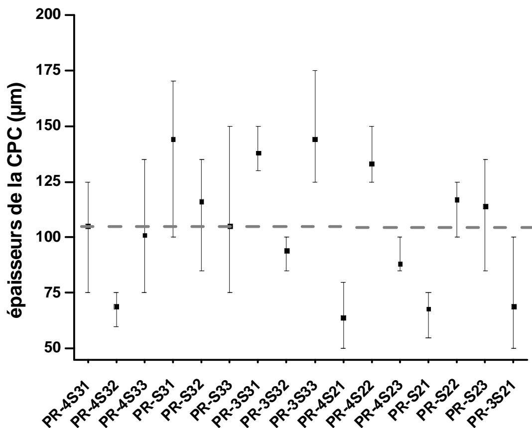
Figure 3.35 : Epaisseurs moyennes de couches de produits de corrosion en microscopie optique. Le trait en pointillés correspond à la valeur moyenne sur l'ensemble des échantillons
