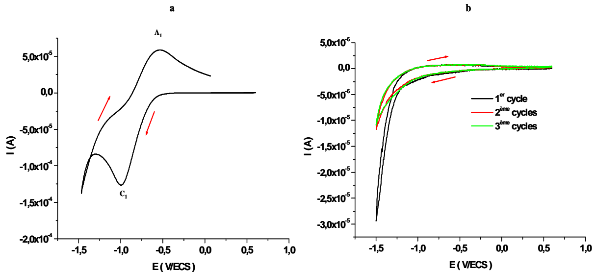
Figure 96 : Voltampérogrammes (1 er cycle) obtenus avec une électrode à pâte de carbone de : a. ferrihydrite deux raies, b. blanc, dans une solution de Na 2 CO 3 0,04 M à pH=11
