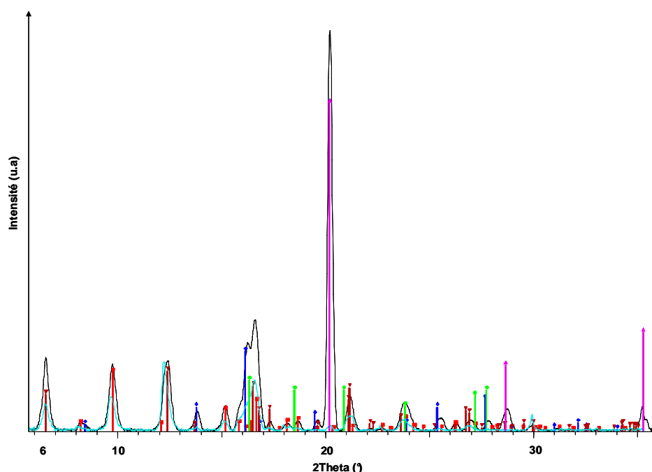
Figure 3.48 : Diagrammes des diffractions des rayons X enregistrés sur des produits de corrosion grattés du système « ferrihydrite », sur deux semelles S_1 (noir) et S_3 (bleu ciel). Identification de la goéthite (carrés rouges, JCPDF n°081-0464), de la lépidocrocite (triangles marrons, JCPDF n°44-1415), de la maghémite (carrés bleus, JCPDF n°39-1346), de la magnétite (carrés bleus, JCPDF n°19-0629) et du métal (triangles roses, JCPDF n°06-0696).
