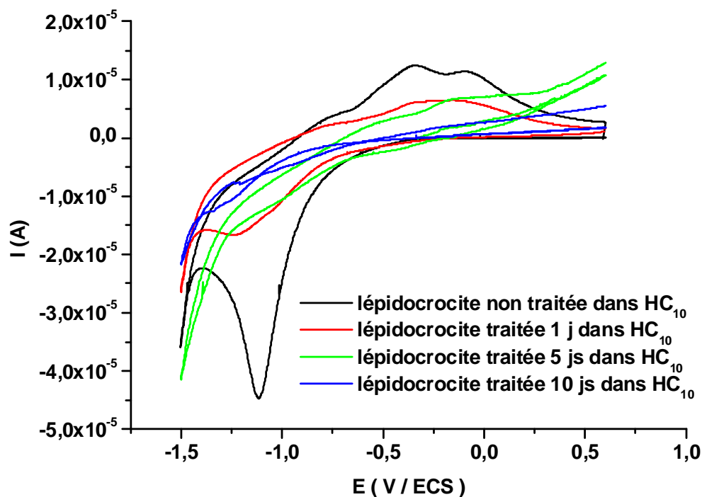
Figure 4.71 : Voltampérogrammes (1er cycle) obtenus avec une électrode à pâte de carbone de poudre de la lépidocrocite non traitée, et traitée à différents temps d’immersions dans HC_{10} , dans une solution de Na_2SO_4 10^{-1}M à pH=7
