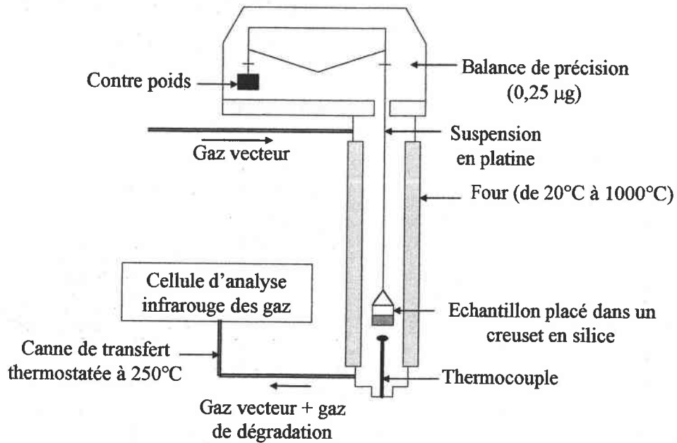
Figure 21 : Schéma de l'appareil d'analyse thermogravimétrique
