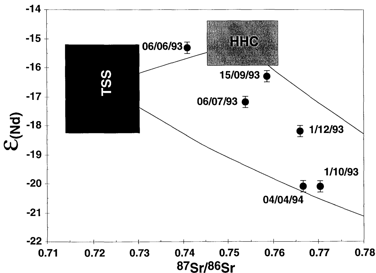
Figure V-26 : Composition isotopique du Nd en fonction de celle du Sr pour la fraction silicatée des sédiments de la Trisuli à Betrawati. La date de prélèvement est indiquée à proximité de chaque point. Les échantillons des périodes sèches contiennent plus de matériel dérivée du LH.
