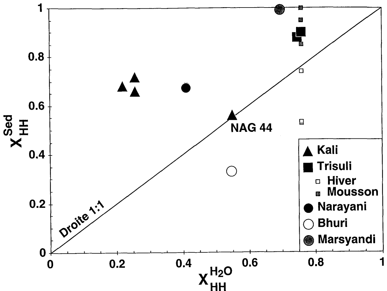
Figure V-29 : Proportion de sédiment de rivière provenant du Haut Himalaya en fonction de la proportion annuelle d'eau provenant du même endroit. La présence de blocs et galets dans NAG 44 entraîne une sous-estimation de la proportion de HH. L'écart à la droite de pente 1 indique que les précipitations orographiques, n'est pas le seul facteur augmentant l'érosion du HH par rapport à celle du LH.
