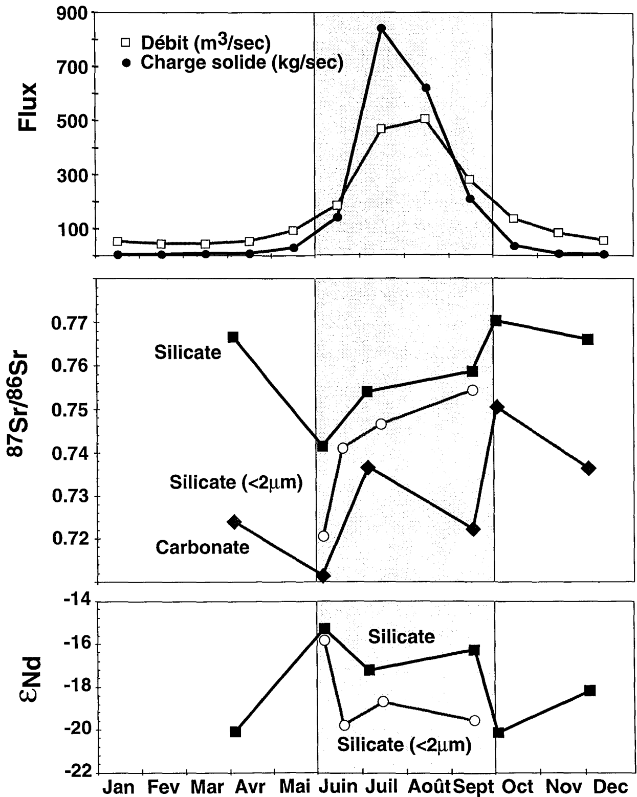
Figure V-25 : Variation de la composition isotopique en Sr et Nd des différentes fractions (silicatée, carbonatée et argileuse) des sédiments de la Trisuli à Betrawati en fonction de la saison d'échantillonnage.
