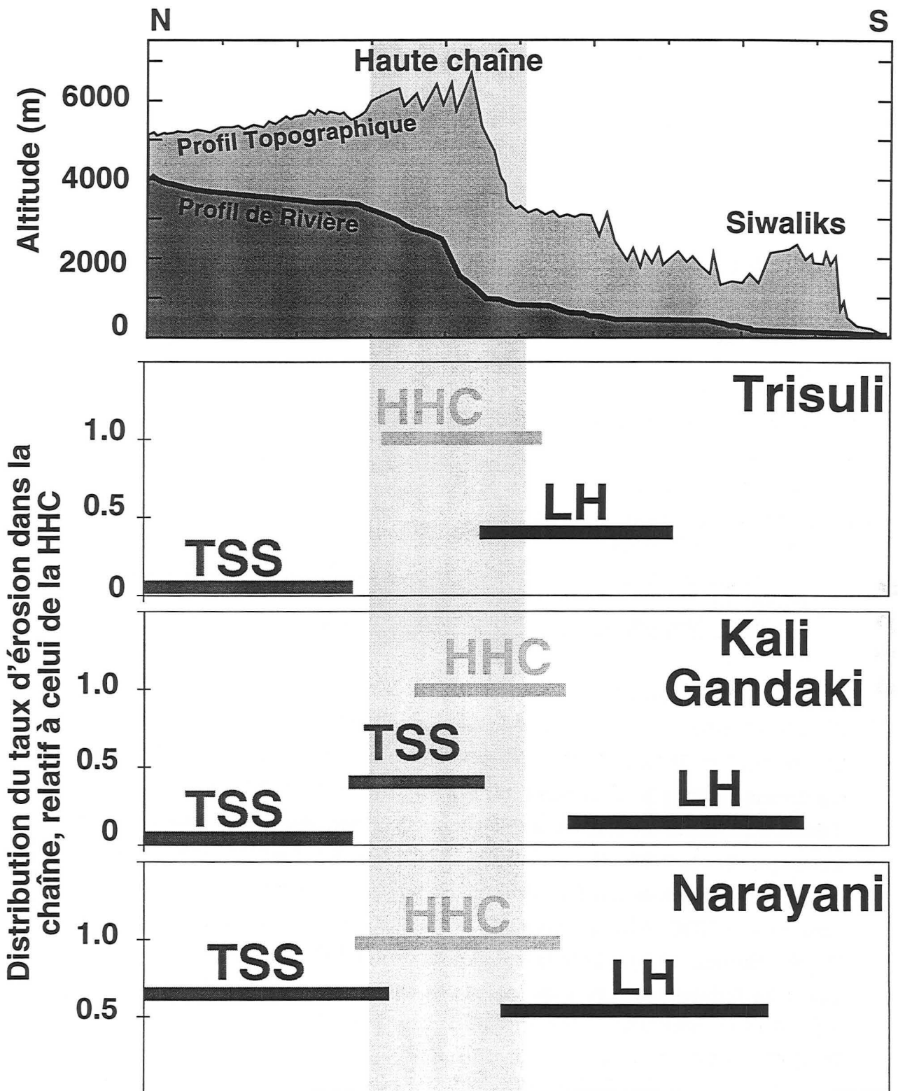
Figure V-28 : Comparaison de la répartition spatiale des taux d'érosion entre le bassin de la Trisuli et celui de la Kali Gandaki au Népal Central. Les surfaces au Nord de la haute chaîne sont plus faiblement érodées que le flanc Sud. La différence d'érosion du LH par rapport à la HHC est contrôlée par la position plus ou moins élevée du MCT.
