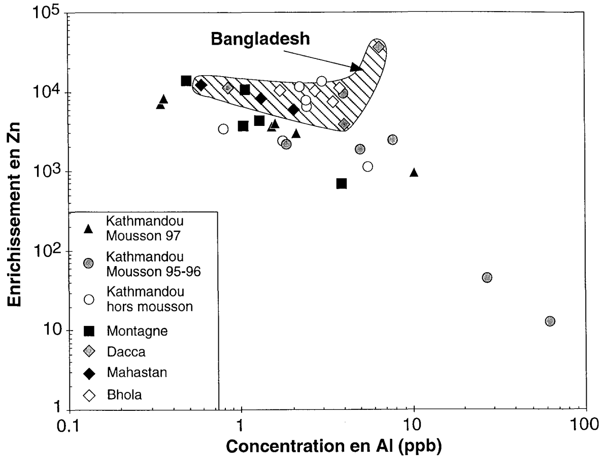
Figure III-32 : Facteur d'enrichissement du Zn en fonction de la teneur en Al.
