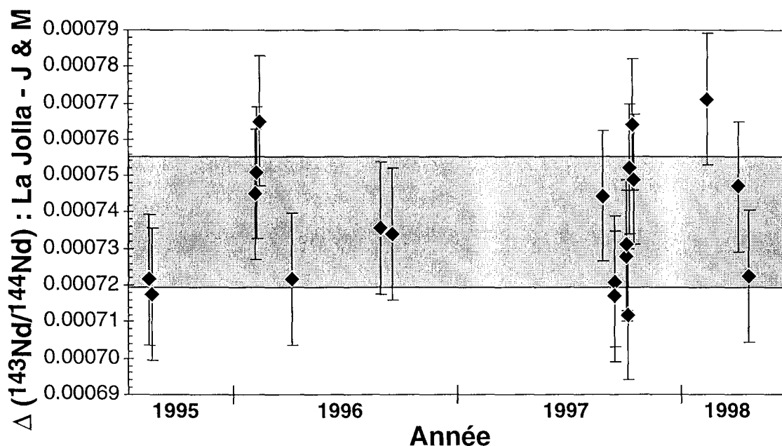
Figure II-4 : Variation temporelle de l'écart de composition isotopique du Nd pour les deux standards utilisés (La Jolla et J & M). Les barres d'erreurs sont en 2\sigma .
