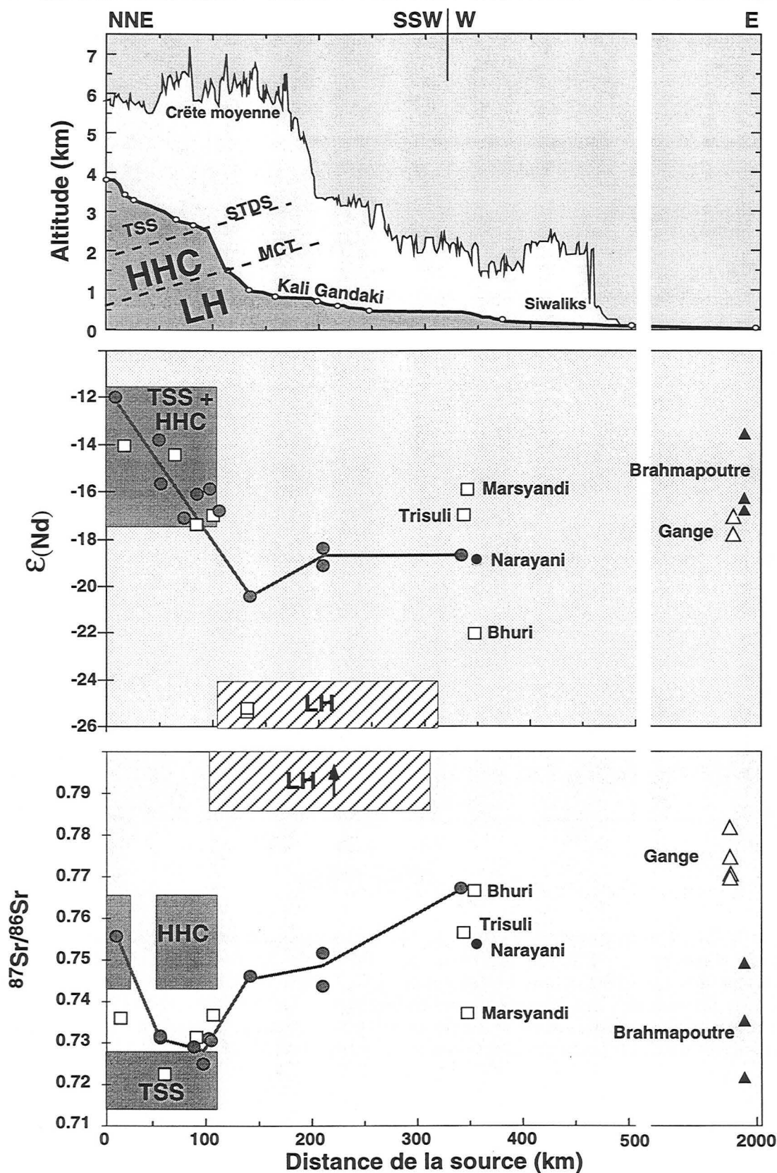
Figure V-22 : Variation de la composition isotopique du Sr et du Nd de la fraction silicatée des sédiments de rivières le long du profil de la Kali Gandaki, depuis sa source en flanc nord de la chaîne, jusqu'à son entrée dans la plaine du Gange. Les carrés sont les affluents, alors que les ronds indiquent le drain principal. Le profil topographique est d'après Hurtrez (1998).
