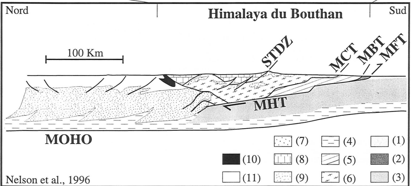
Figure III-3 : Coupe synthétique de la chaîne himalayenne, d'après la cartographie (France-Lanord et Le Fort, 1988) et les profils sismiques (Nelson et al. , 1996). THB : batholite du Trans-Himalaya; ITS : Ophiolite de la zone de Indus-Tsangpo; TSS : Séries Sédimentaires Téthysiennes; HHC : formations du Haut Himalaya Cristallin. LH : formations du Moyen Pays. Siwaliks : Sédiments Néogène du bassin d'avant chaîne. STDZ : détachement sud tibétain; MHT : chevauchement principal himalayen; MCT : chevauchement central himalayen; MBT : chevauchement basal himalayen et MFT : chevauchement frontal himalayen. (1) : Sédiments Holocène de la plaine du Gange. (2) : Siwaliks. (3) : Croûte indienne. (4) Croûte inférieure litée. (5) : LH. (6) : HHC. (7) : Leucogranite himalayen. (8) : TSS. (9) : zone de la croûte partiellement fondue. (10) THB+ITS. (11) : Croûte du bloc de Lhassa.
