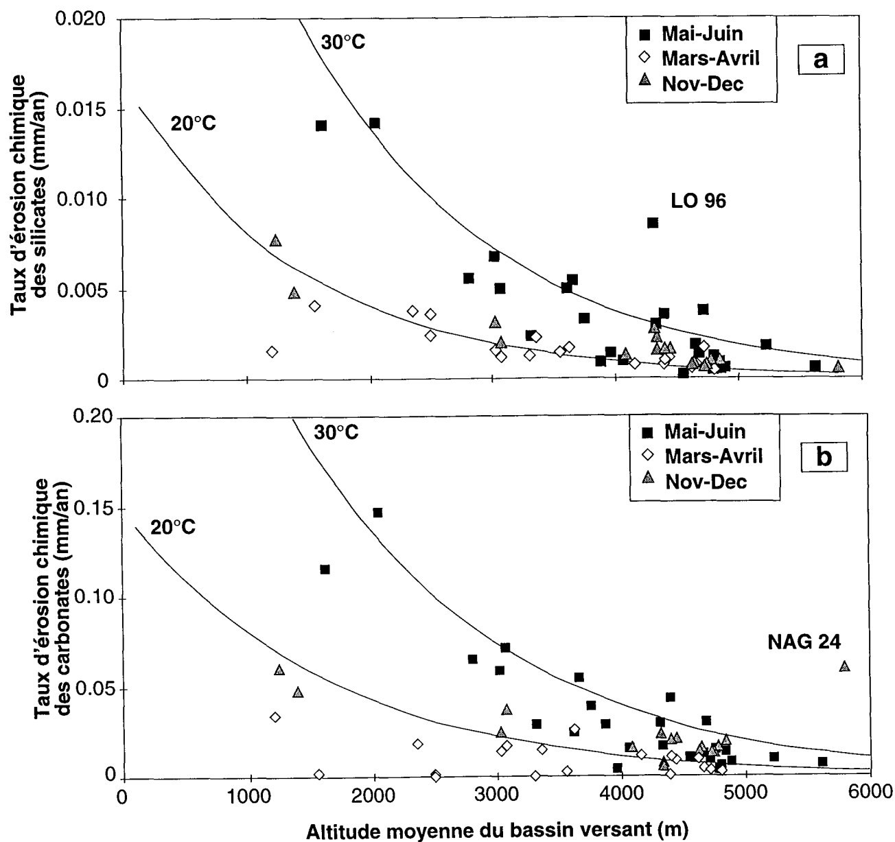
Figure IV-27 : Variation du taux de dénudation des silicates (a) et des carbonates (b) en fonction de l'altitude moyenne des bassins versants et de la saison. Les courbes modélisent une relation de type Arrhenius couplé à un gradient de température linéaire avec l'altitude.
