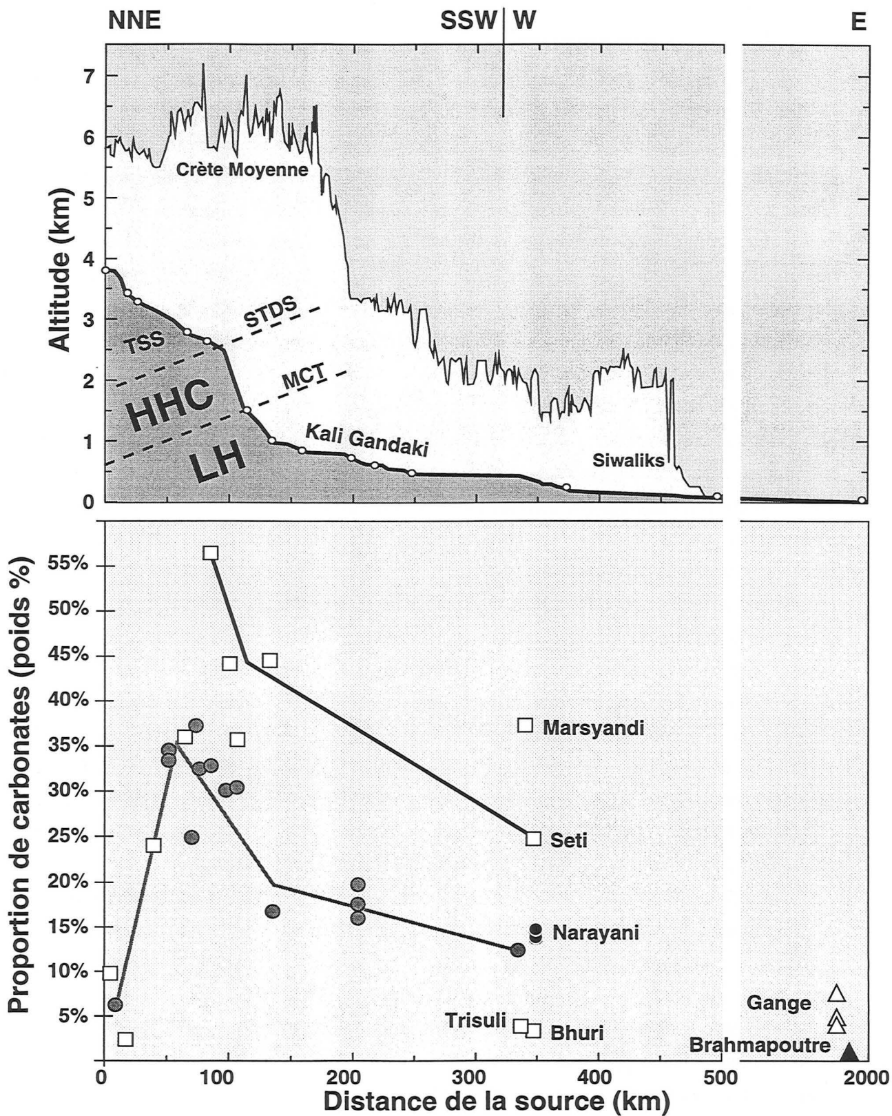
Figure V-16 : Variation de la teneur en carbonate des sédiments de rivières le long du profil de la Kali Gandaki, depuis sa source en flanc nord de la chaîne, jusqu'à son entrée dans la plaine du Gange. Le profil topographique est d'après Hurtrez (1998).
