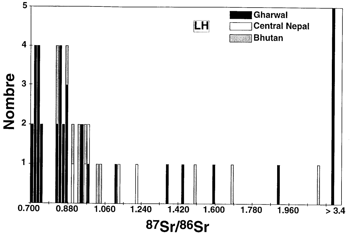
Figure III-11 : Composition isotopique du Sr des roches du LH.
