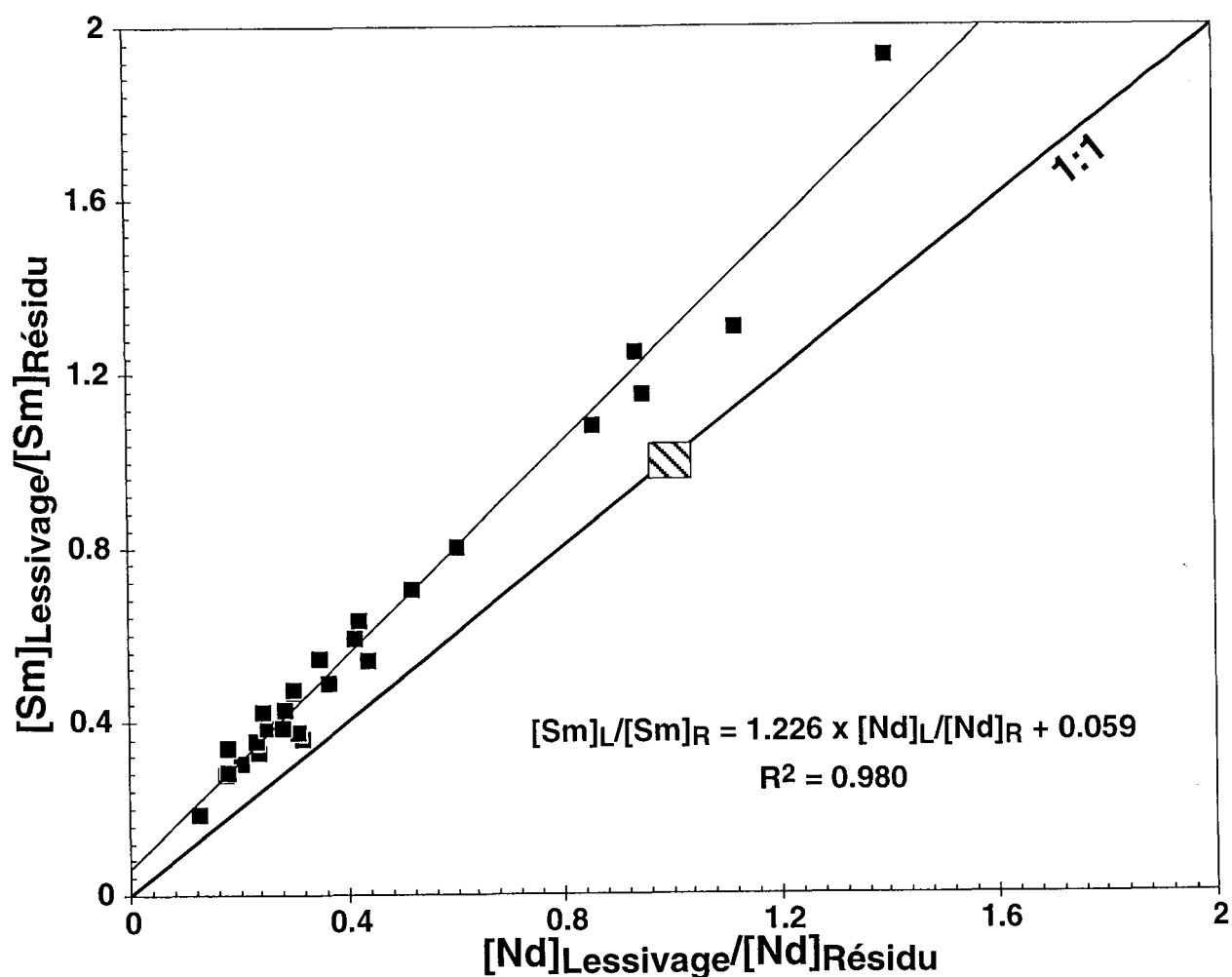
Figure II-18 : Enrichissement relatif en Nd et Sm dans les phases solubles lors de l'attaque ménagée par rapport aux phases insolubles. Le carré hachuré indique une teneur similaire entre la phase soluble et les phases insolubles pour les deux éléments.
