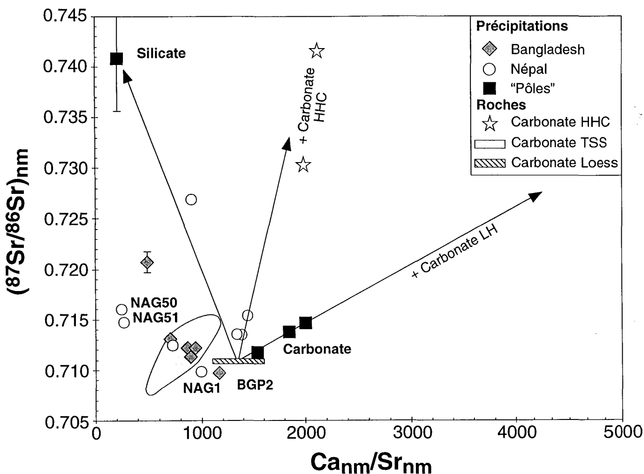
Figure III-29 : Composition isotopique du Sr dissous d'origine non marine en fonction du rapport molaire entre le Ca et le Sr d'origines non marine (corrigés sur la base du Cl). Le pôle silicaté correspond à GK 4 et le pôle carbonaté à NAG 53, 54 et GK 8. Les compositions des carbonates des TSS sont dans la Table III-8. Les carbonates de la HHC sont similaires aux carbonates disséminés décrits par Blum et al. (1998), mais proviennent des environs de Kathmandou (voir chapitre IV). Les carbonates du LH ont des rapports \text{Ca}/\text{Sr} > 5000 . Les carbonates des loess sont d'après Gallet et al. (1996), en supposant une minéralogie de calcite pour le Ca.
