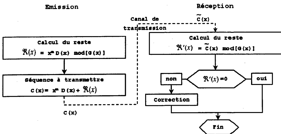
FIG. 2.8 – Détection d'erreurs par CRC.
