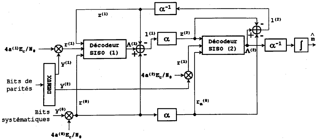
FIG. 3.2 – Exemple d'un turbo-décodeur.
