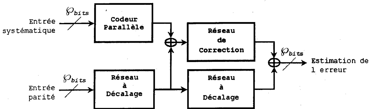
FIG. 6.3 – Schéma fonctionnel du décodeur parallèle.
