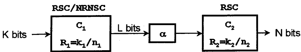
FIG. 2.19 – Turbo-code série.
