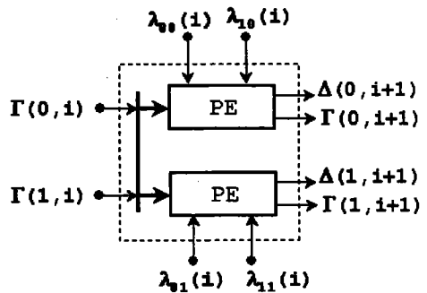
FIG. 3.6 – ACS Radix-2.
