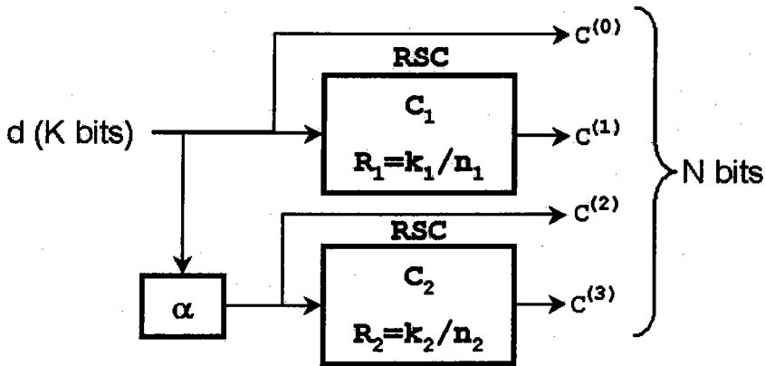
FIG. 2.20 – Turbo-code parallèle.
