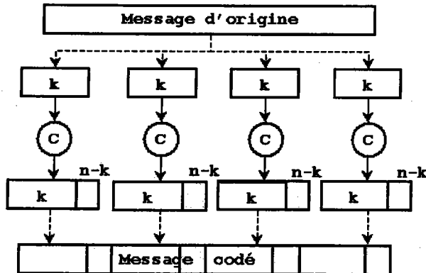
FIG. 2.7 – Codage systématique.
