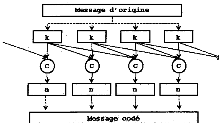
FIG. 2.10 – Codage convolutif.
