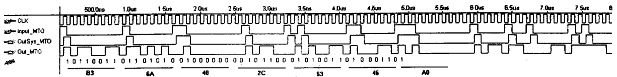
FIG. 5.38 – Simulation du codeur RSC série Many To One ( CS_{mto} ).
