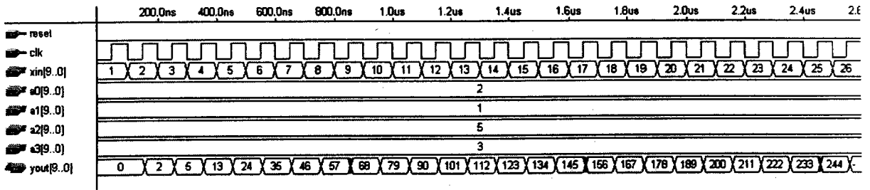
FIG. 4.22 – Simulation du réseau de convolution non récursive DR.
