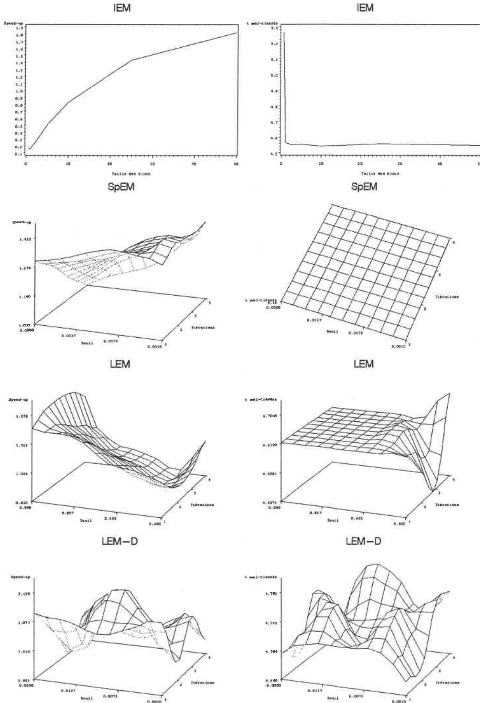
FIG. 4.6 – Degré de mélange (+) : IEM, SpEM, LEM et LEM-D (Coefficient d'accélération à gauche et pourcentage de mal-classés à droite). Ici, SpEM trouve toujours le même pourcentage de mal-classés, c'est pourquoi le graphique est ainsi.
