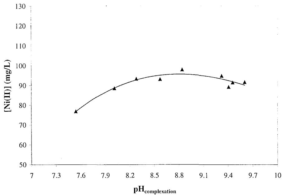
Figure 3.2 Concentration de Ni(II) mesurée dans la solution en fonction du pH de complexation. 0.5 M NH 4 Cl, T= 25°C, V f-liq = 100 ml, W b = 1.5 g.
