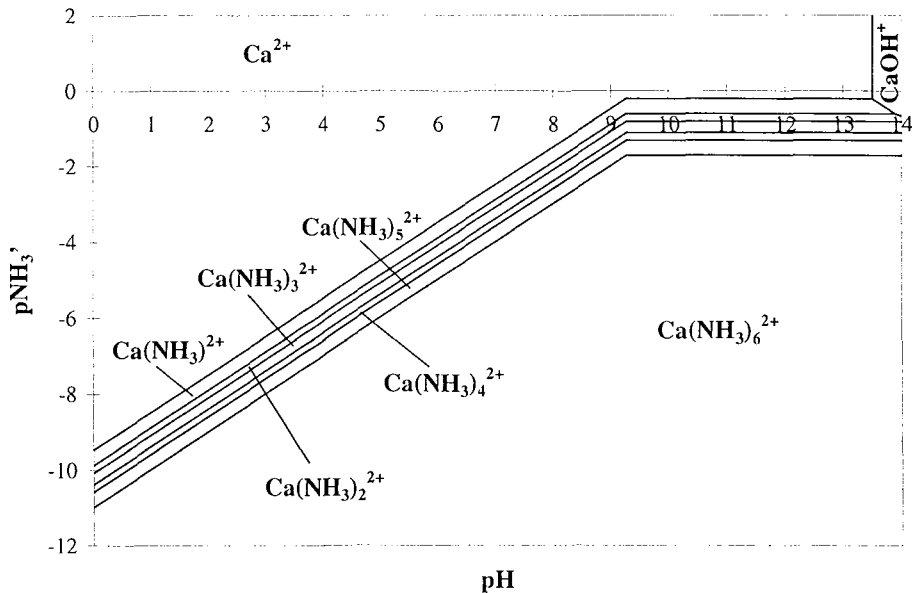
Figure 3.4 Diagramme de zones de prédominance pour le système \text{Ca(II)}-\text{NH}_3-\text{H}_2\text{O} .
