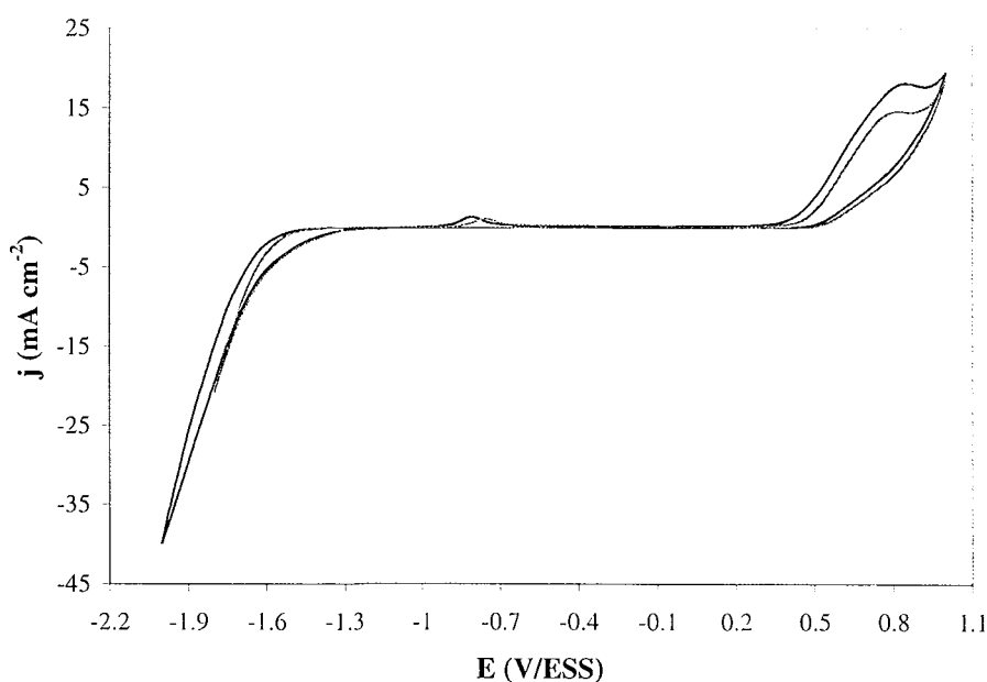
Figure 7.9 Voltammogramme de \text{NiSO}_4 \cdot 7\text{H}_2\text{O} 0.12 M, Glycine 2 M, \nu = 50 \text{ mVs}^{-1} , \text{pH} = 8 , T = 25^\circ\text{C} . à différentes limites de potentiel, (---) -1.8 et (—) -2 V/ESS.
