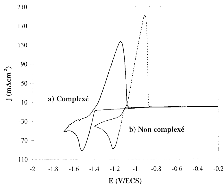
Figure 5.5 Comparaison des courbes courant - potentiel du zinc complexé et non complexé. a) Voltammogramme du système \text{ZnCl}_2 0.22 M et \text{NH}_3 4 M, \nu = 50 \text{ mVs}^{-1} , pH= 10, T= 25°C. b) Zn non complexé.
