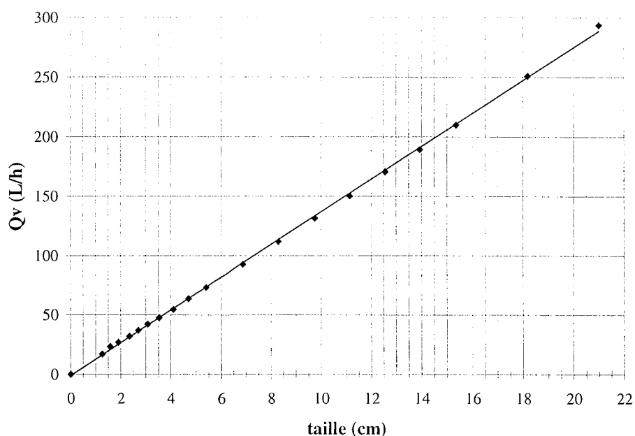
Figure D.1 Courbe d'étalonnage pour les deux débitmètres.
