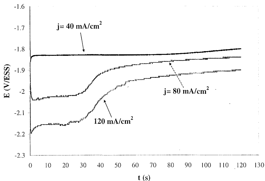
Figure 7.15 Variations transitoires du potentiel à différentes densités de courant sur une électrode à disque tournante à 1000 tours/min à partir de la solution de lixiviation française avec la glycine. T=25^{\circ}\text{C} .
