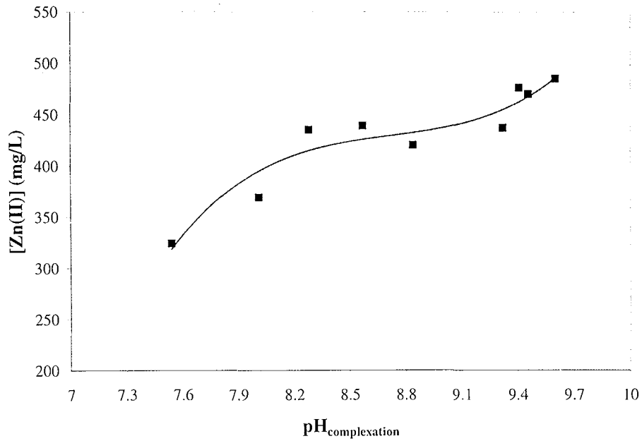
Figure 3.1 Concentration de Zn(II) mesurée dans la solution en fonction du pH de complexation. 0.5 M NH 4 Cl, T= 25°C, V f-liq = 100 ml, W b = 1.5 g.
