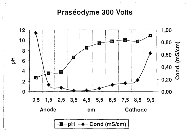
Figure VII-12 . Profils de pH et de conductivité des solutions préparées à partir des fractions de lit imprégné avec une solution \text{PrCl}_3 , \text{K}_2\text{H}_2\text{Y} à 0.0025 M, après 30 minutes sous une tension appliquée de 300 Volts.
