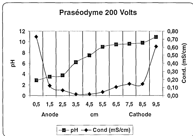
Figure VII-11 Profils de pH et de conductivité des solutions préparées à partir des fractions de lit imprégné avec une solution \text{PrCl}_3 , \text{K}_2\text{H}_2\text{Y} à 0.0025 M, après 30 minutes sous une tension appliquée de 200 Volts.
