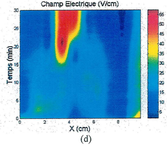
Figure VII-15 Distributions du potentiel à 100 Volts et du champ électrique pour le complexe PrY^1 en 3D (a) et (c) et 2D (b) et (d).
