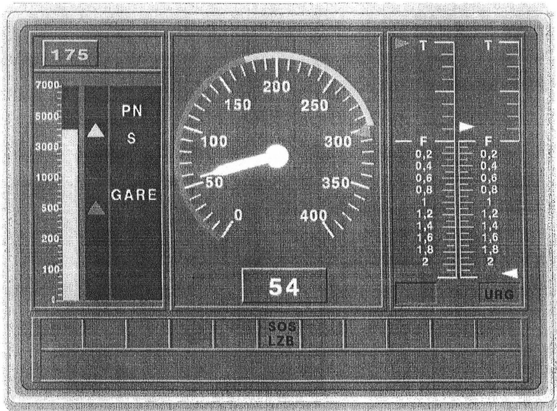
Figure 36 : Préconception d'interface avec barregraphes pour les niveaux de traction et de freinage.
