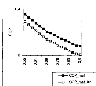
Figure 4.14 : Evolution du COP en fonction de T_{SI}^H pour les machines à froid
