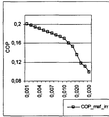
Figure 4.12 : Evolution du COP en fonction de \bar{S}^H pour les machines à froid
