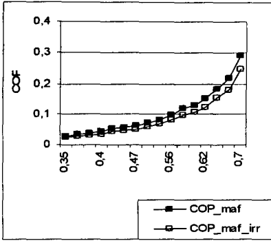
Figure 4.13 : Evolution du COP en fonction de T_{SF}^H pour les machines à froid
