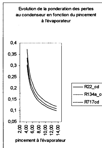
Figure 2.16 : Evolution des pondérations des pertes au condenseur en fonction du pincement à l'évaporateur
