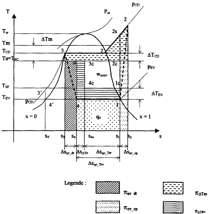
Figure 2.10 : Représentation graphique des pertes énergétiques internes et externes pour la machine à froid ditherme
