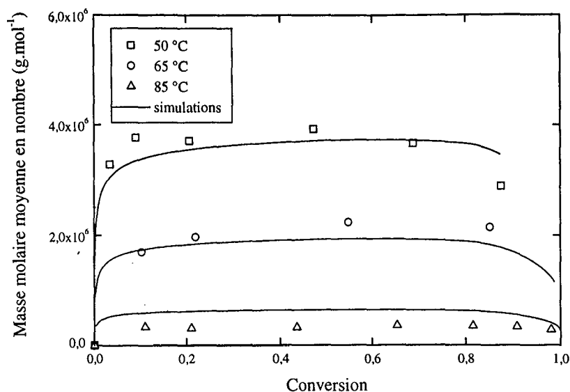
Figure 4.3 : comparaison de l'évolution des masses molaires moyennes en nombre expérimentales et simulées en fonction de la conversion pour différentes températures
