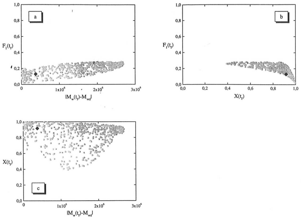
Figure 6.14 : meilleure (♦) et 600 premières solutions du front de Pareto obtenues par bilans de flux pour le système de copolymérisation pour les trois critères f_1 , f_2 et f_3
