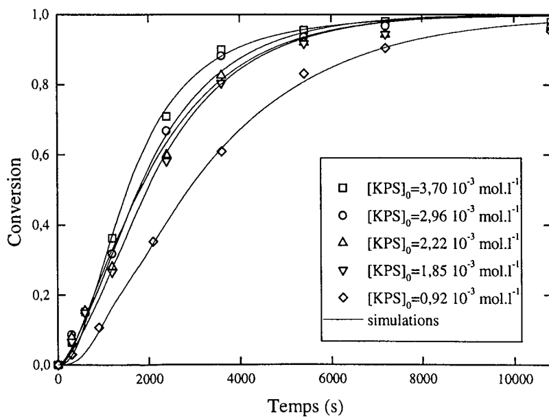
Figure 3.4 : comparaison de l'évolution des conversions expérimentales et simulées en fonction du temps pour une concentration initiale en tensioactif fixée à [SDS]_0 = 2,13 \text{ cmc}
