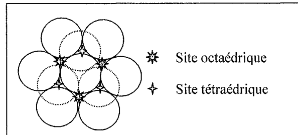
Figure III.27 : Représentation schématique du mécanisme de pseudo-maclage ; schéma d'un empilement dense CFC avec localisation des sites octaédriques et tétraédriques.
