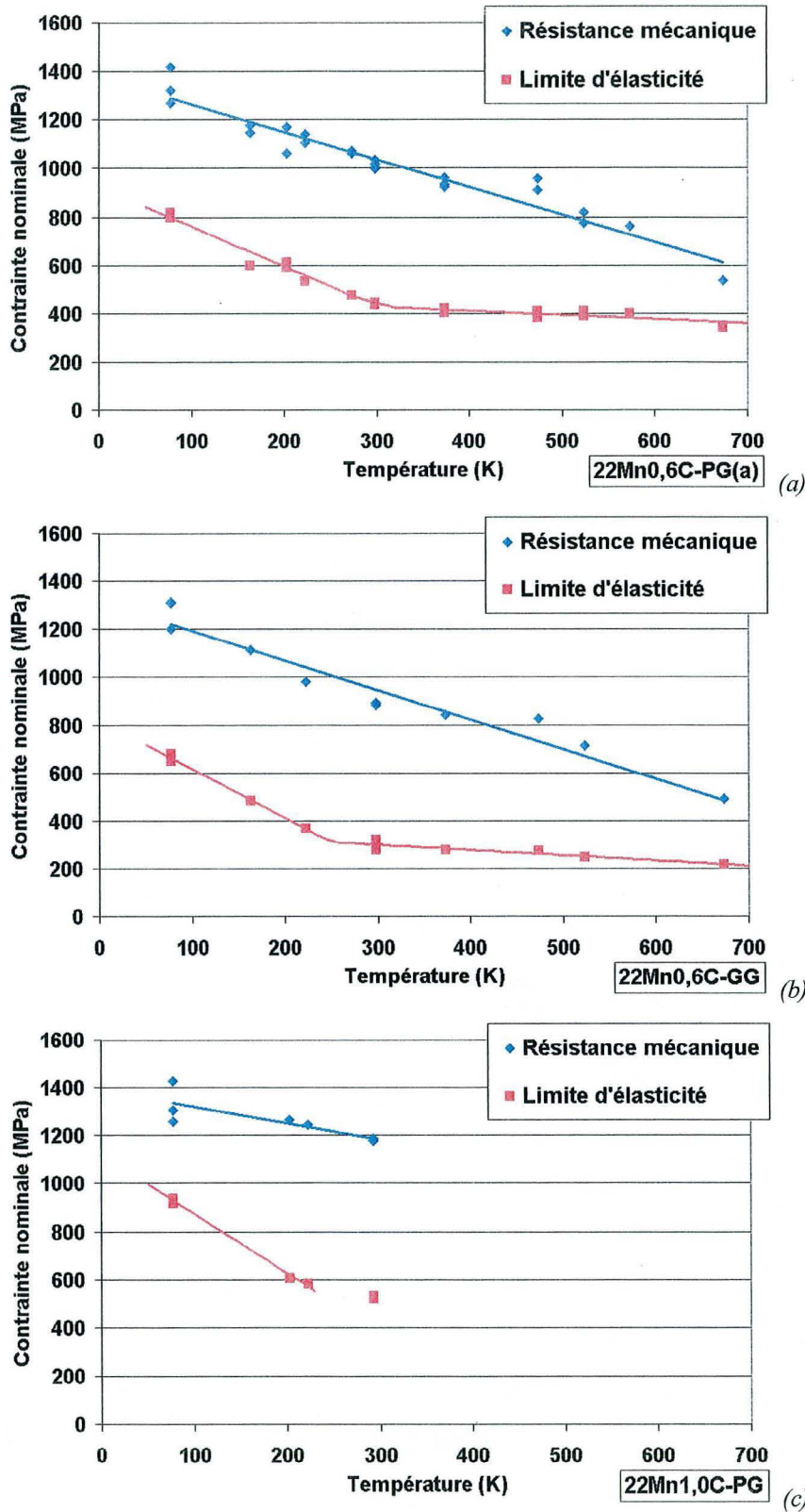
Figure III.4 : (a), (b) et (c) Résistances mécaniques et limite d'élasticité des alliages 22Mn0,6C-PG(a), 22Mn0,6C-GG et 22Mn1,0C-PG respectivement à différentes températures. Les résistances mécaniques décroissent linéairement avec la température et les limites d'élasticité atteignent un palier quasiment athermique au-dessus de 300 K et 250 K pour les nuances 22Mn0,6C-PG(a), 22Mn0,6C-GG respectivement.
