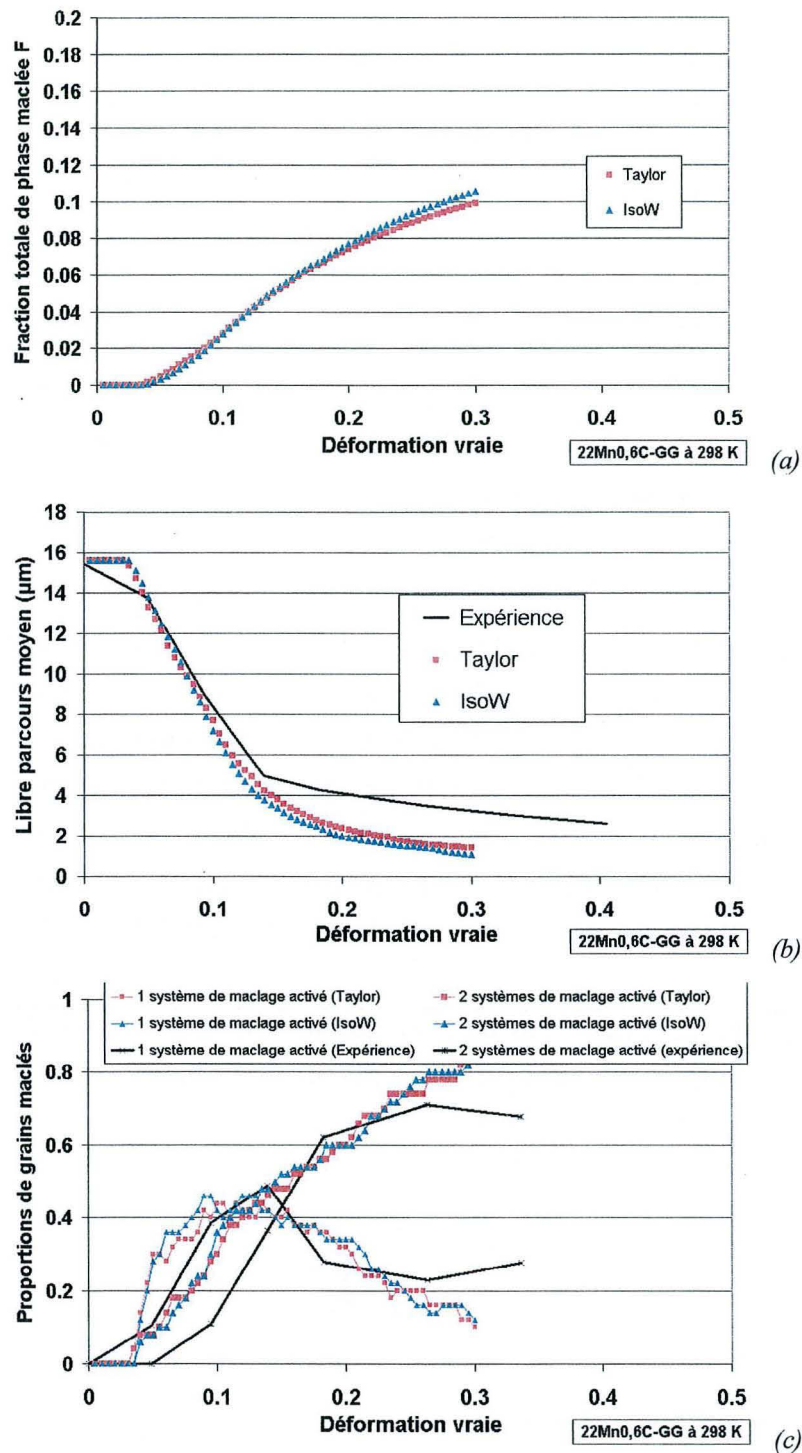
Figure V.8 : Résultats expérimentaux et de simulation selon le modèle de Taylor et IsoW concernant l'évolution de la microstructure de maillage de la nuance 22Mn0,6C-GG à 298 K : (a) cinétique de maillage F, (b) évolution du libre parcours moyen L et (c) évolution de la fraction de grains maclés par un et deux systèmes de maillage respectivement.
