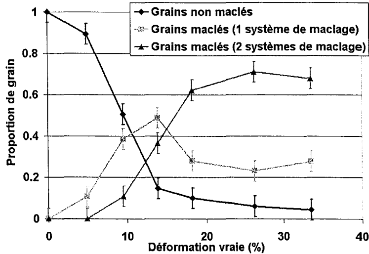
Figure IV.13 : Évolution de la proportion de grains non maclés, ou maclés avec 1 ou 2 systèmes de maclage activés. Cette mesure a été réalisée en microscopie optique sur la nuance 22Mn0,6C-GG après attaque.
