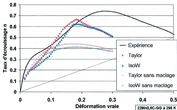
Figure V.9 : Taux d'écroutissage des courbes de traction expérimentale et simulées selon Taylor et IsoW de la nuance 22Mn0,6C-GG à 298 K. Les courbes sans maclage sont obtenues à partir des courbes de traction de la figure V.3(a).
