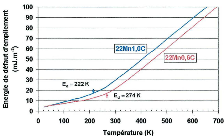
Figure III.17 : Évolution de l'EDE calculée en fonction de la température pour les nuances étudiées. Les températures théoriques de transition E_d ont été repérées par des flèches pour les deux nuances.
