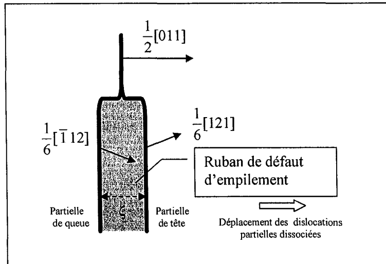
Figure I.8 : Représentation schématique de la dissociation d'une dislocation parfaite de type coin en deux dislocations partielles bordant un défaut d'empilement. Définition de la partie de tête et de queue.
