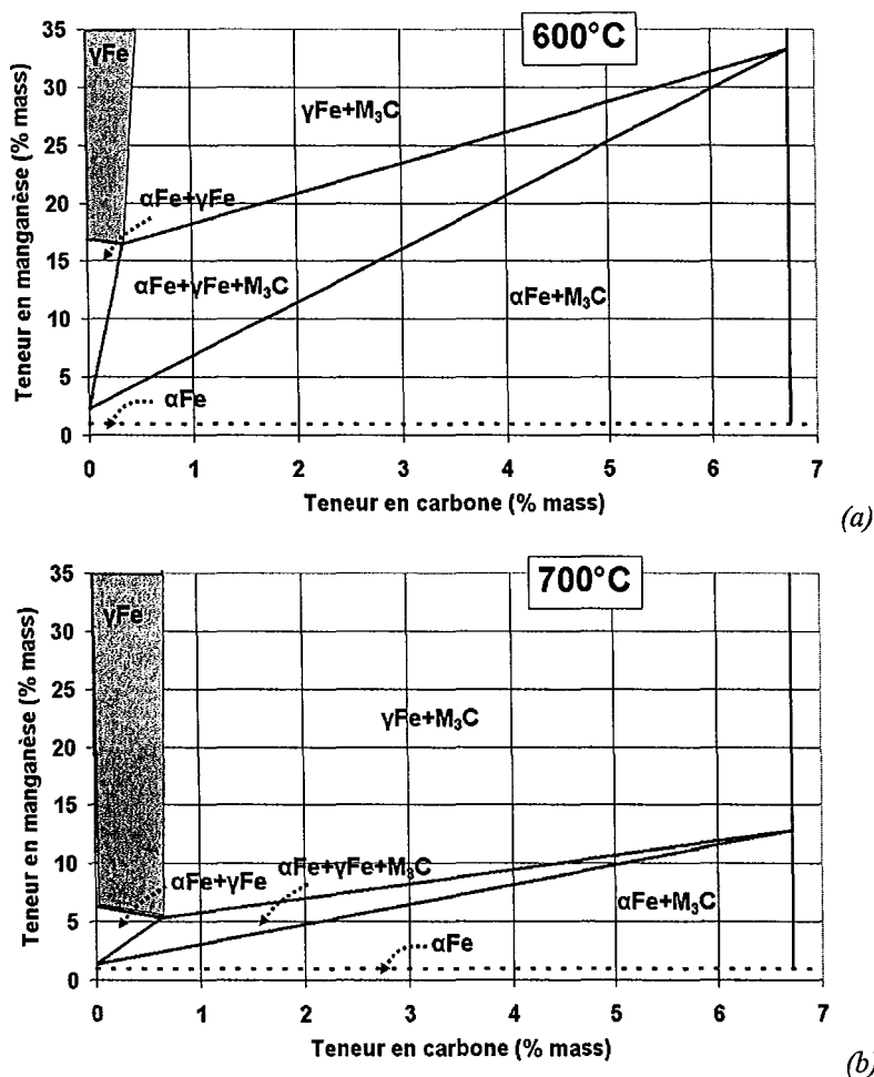
Figure 1.4 : Coupes du diagramme de phases stables des alliages ternaires Fe-Mn-C riches en fer à 600°C et 700°C d'après [Raynor & Rivlin 88]. Les composés \text{M}_3\text{C} sont des carbures \text{Fe}_3\text{C} ou \text{Mn}_3\text{C} .
