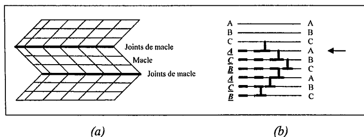
Figure I.10 : (a) représentation schématique d'une macle dans un arrangement périodique. Les joints de macles sont des plans de symétrie. (b) Représentation schématique du réarrangement des plans compacts autour d'une macle mécanique créée par le déplacement de dislocations partielles intrinsèques tous les plans atomiques. La flèche indique la position du joint de macle plan miroir pour le réseau CFC.
