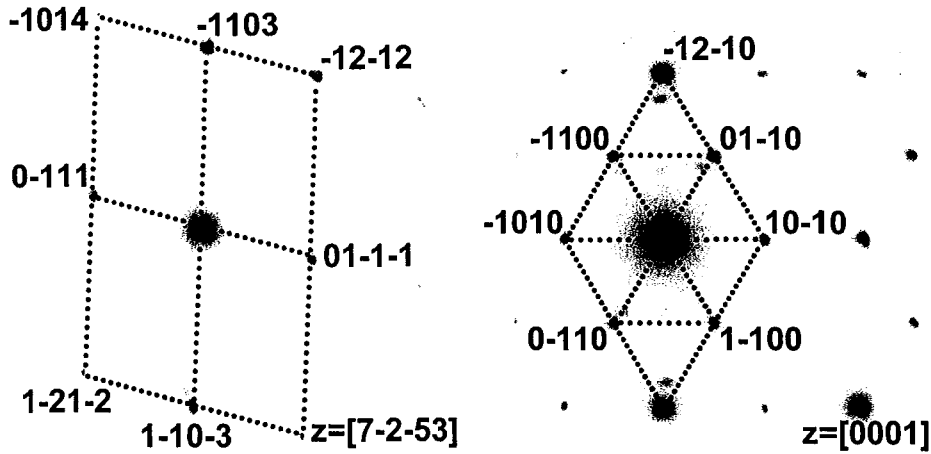
Figure III.10 : Clichés de diffraction obtenus sur des structures lamellaires observées à l'intérieur des grains. Les symétries et les distances réticulaires sont spécifiques à la martensite \epsilon . (a) axe de zone [7-2-53] et (b) axe de zone de symétrie 6 [0001] .
