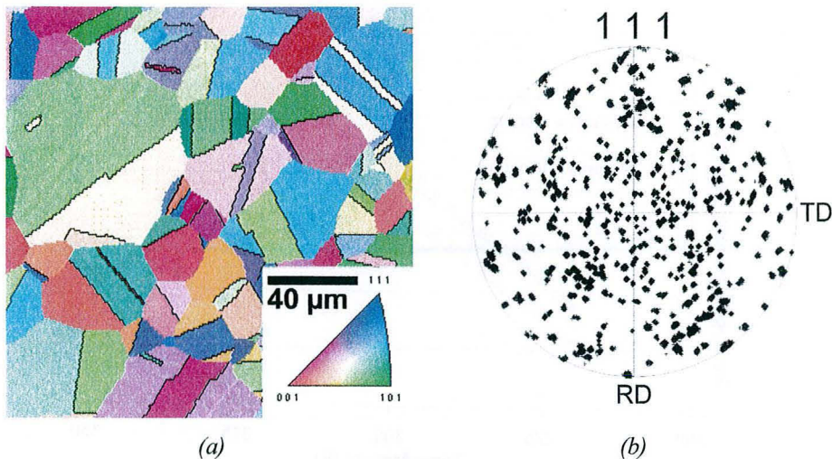
Figure II.6 : (a) Cartographie en orientation de la nuance 22Mn0,6C-GG avant déformation. Les joints de grain tracé en noir indiquent une désorientation de type \Sigma 3 . La correspondance entre les nuances de couleur et les orientations est donnée en insert. (b) Localisation des axes \langle 111 \rangle des grains de la cartographie. Le plan (TD,RD) correspond au plan de l'échantillon.
