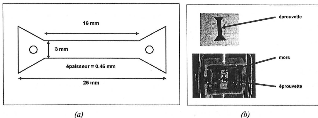
Figure A1.1 : (a) Dimensions de l'éprouvette de la nuance 22Mn0,6C-GG usinée spécifiquement pour être cartographiée dans le MEB FEG (b) Photo de l'éprouvette et du dispositif de traction.
