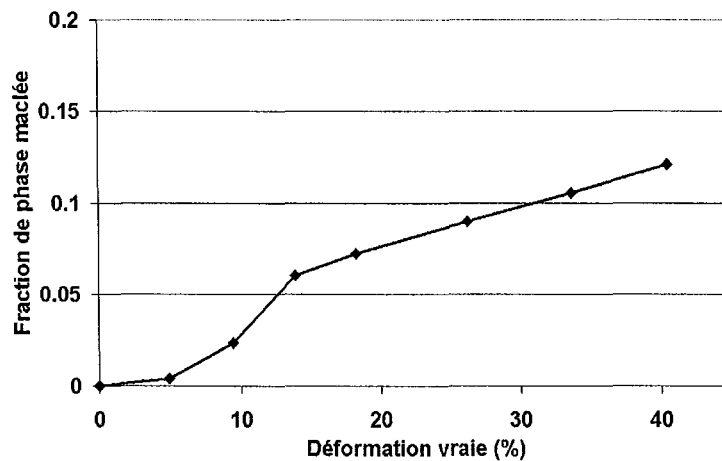
Figure IV.19 : Cinétique de maclage calculée par rapport aux mesures expérimentales du libre parcours moyen de la figure IV.17.
