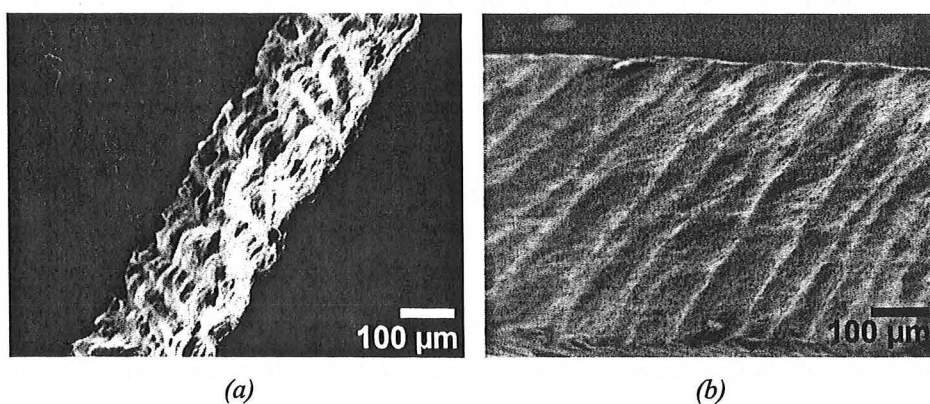
Figure II.4 : Clichés MEB (a) en mode BSE topographique et (b) en mode SE d'une épaisseur d'éprouvette non déformée. Les stries dues à la découpe laser sont visibles mais aucune microfissure n'a pu être détectée.
