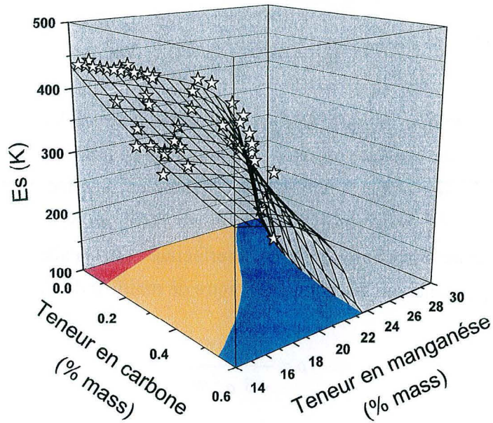
Figure I.17 : Évolution de la température E_s en fonction de la teneur en manganèse et en carbone. La nappe représente les résultats du modèle avec une résistance à la transformation de \Delta G_{E_s}^* = -100 \text{ J.mol}^{-1} . Les étoiles indiquent les résultats expérimentaux issus de la littérature [Ishida & Nishizawa 74][Schumann 72][Rémy 75b][Baik et al. 97][Jun & Choi 98][Lee et al. 96].
