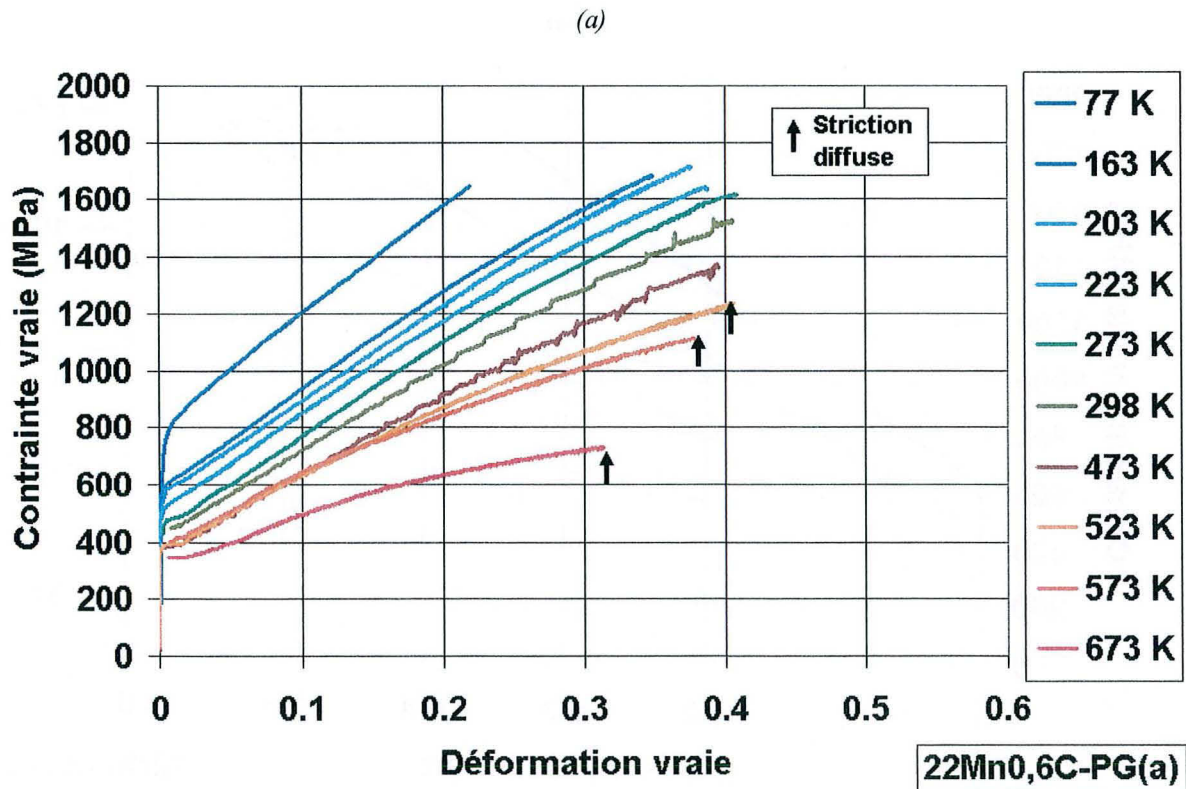
Figure III.1 : Courbes de traction (a) nominales et (b) rationnelles de la nuance 22Mn0,6C-PG(a) ( d_F = 3 \mu m )
