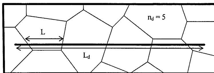
Figure II.5 : Grandeurs caractéristiques utilisées par la méthode des interceptes. Une structure de grains polygonaux ayant été révélée, la droite de longueur totale L_d coupe n_d joints de grains (ici n_d = 5 ).
