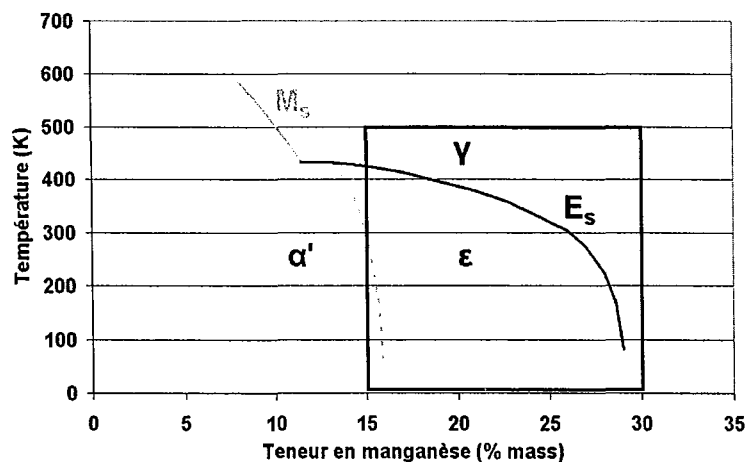
Figure I.2 : Évolution des températures de transformation E_s et M_s en fonction de la teneur massique en manganèse d'après Rémy [Rémy 75a]. La zone encadrée correspond au domaine étudié sur la figure I.3.
