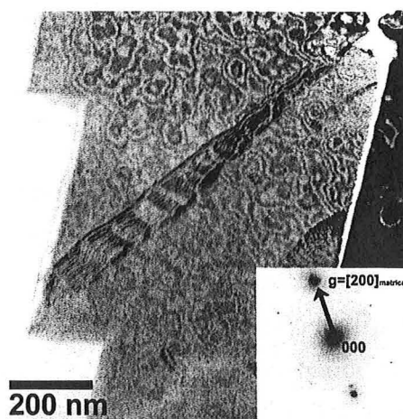
Figure IV.8 : Micrographie DF d'une micromacle émise près d'une microfissure bloquée par un joint de grains en bas à gauche dans un échantillon non déformé. Les franges sont produites par des fautes d'empilement se superposant à différentes hauteurs.
