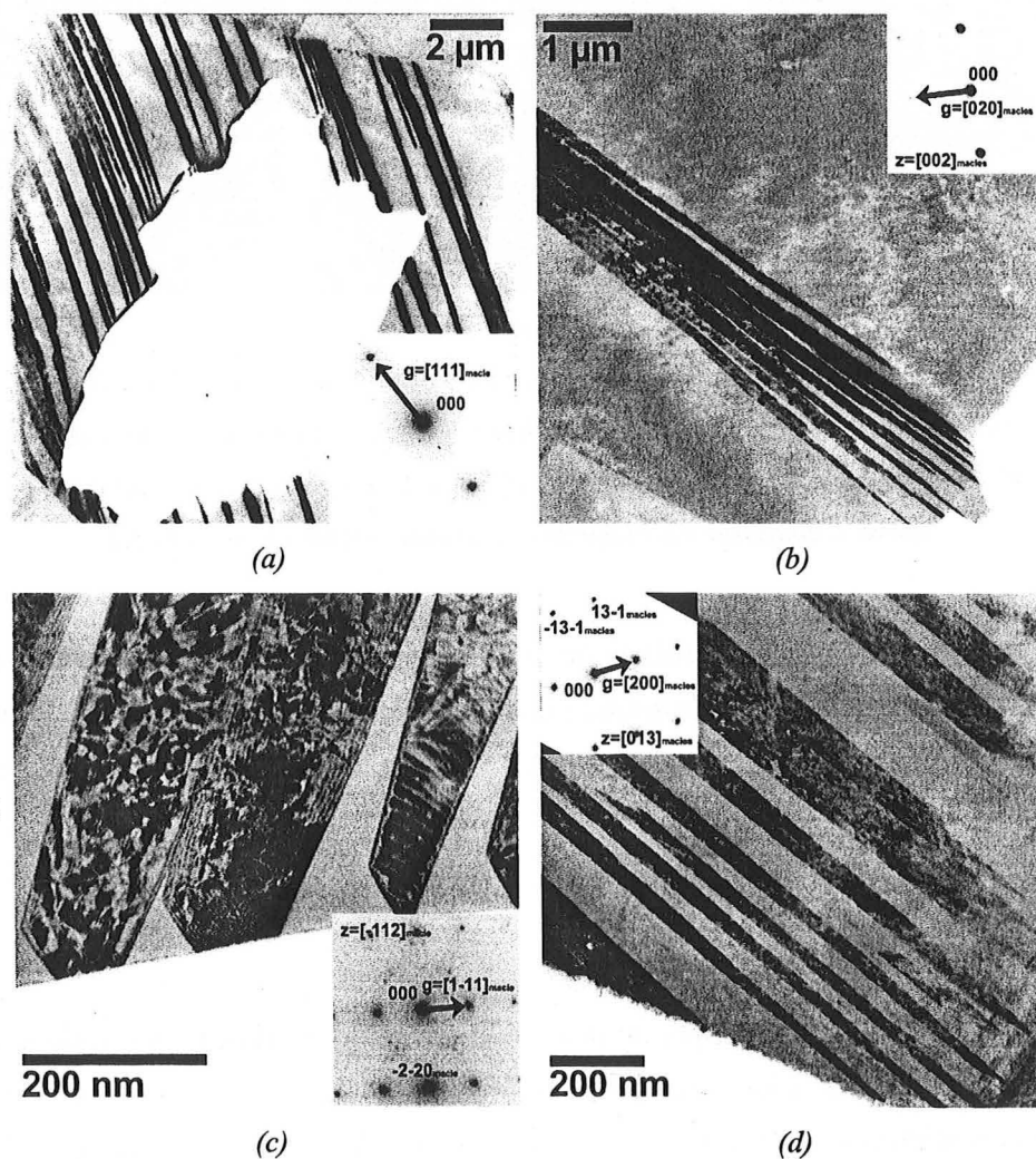
Figure IV.1 : Micrographies MET DF sur des échantillons déformés (a), (b), (c) de 15 % et (d) de 33 %. Quelques micromacles isolées sont présentes dans l'austénite non maclée sur les clichés (a), (c) et (d). La micrographie (c) est prise en condition WB(g,3g).
