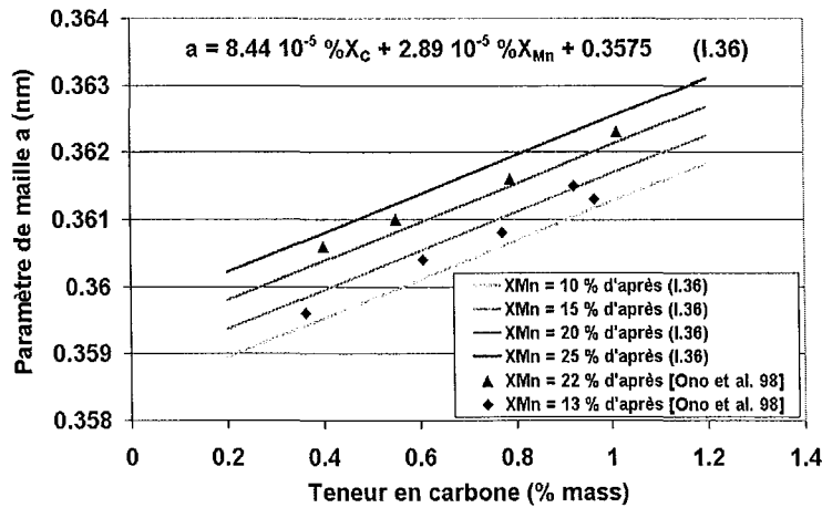
Figure I.18 : Évolution du paramètre de maille avec la teneur massique en carbone à température ambiante pour différentes teneurs en manganèse. Les points représentent les mesures expérimentales de Ono et al. [Ono et al. 98] et les droites les résultats de la modélisation par une loi bilinéaire.
