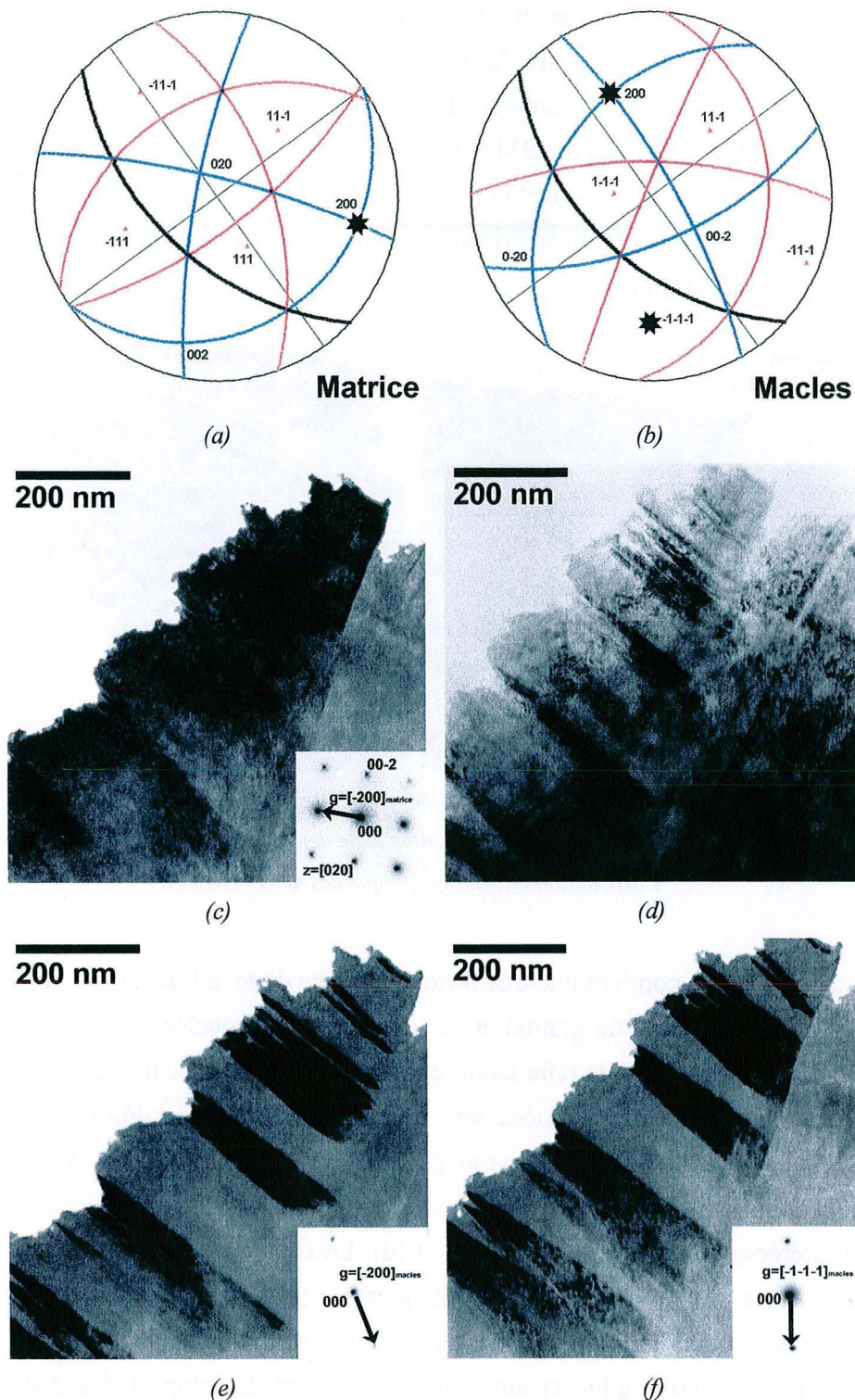
Figure III.12 : (a) et (b) Orientations cristallographiques de l'austénite non maclée et des macles vues en projection stéréographique. Le plan de la lame mince est celui de la projection. Les plans rouges correspondent aux plans \{111\} et les bleus aux plans \{100\} . La convention d'indexation est définie par l'équation (III.8). Le plan de maillage K_1 est représenté en noir. (c) Micrographie DF selon un vecteur de diffraction de la matrice non maclée. (d) Micrographie BF sur laquelle les macles sont en contraste. (e) et (f) Micrographies DF selon des vecteurs de diffraction appartenant à la figure de pôles des macles.
