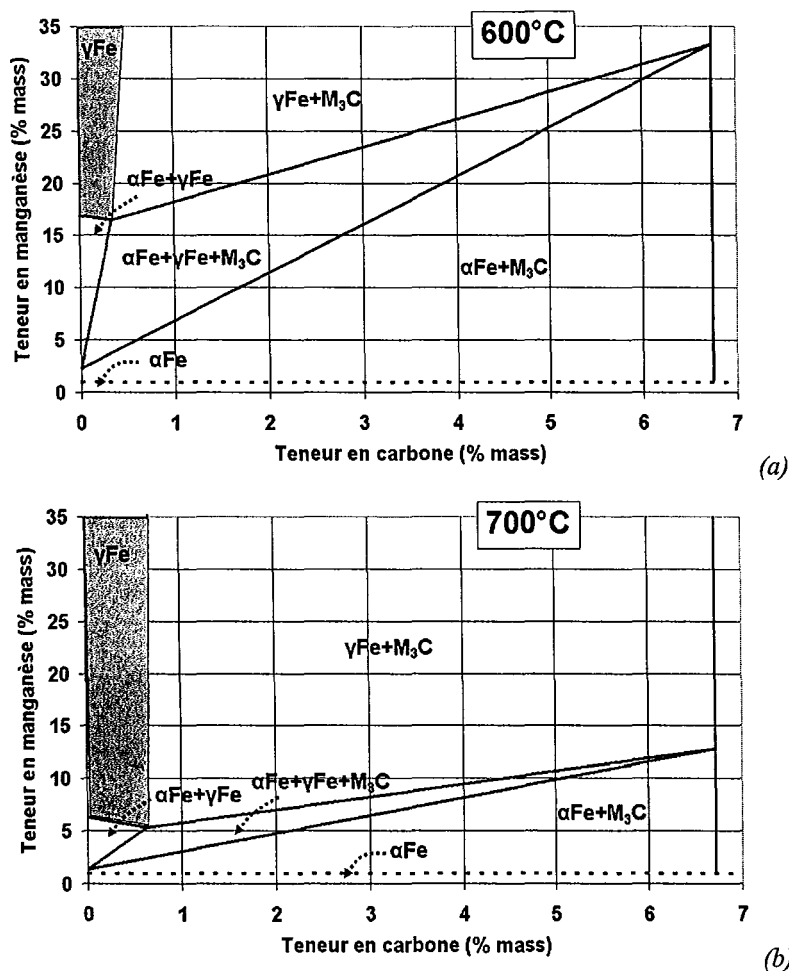
Figure 1.4 : Coupes du diagramme de phases stables des alliages ternaires Fe-Mn-C riches en fer à 600°C et 700°C d'après [Raynor & Rivlin 88]. Les composés M_3C sont des carbures Fe_3C ou Mn_3C .
