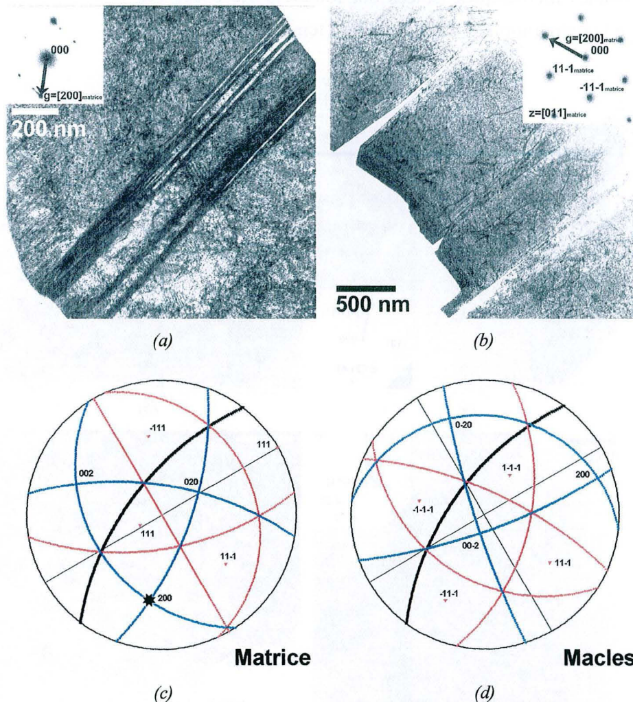
Figure III.13 : Micrographies de la nuance 22Mn0,6C-GG (a) DF, un grain maclé après 14 % de déformation vraie (b) WB( g,3g ) d'un grain maclé après 5 % de déformation. Les vecteurs de diffraction respectifs appartiennent à la matrice pour mettre en contraste une partie des dislocations et des défauts d'empilements. (c) et (d), projections stéréographiques des orientations cristallines respectives de l'austénite non maclée et des macles du grain de la figure (a).
