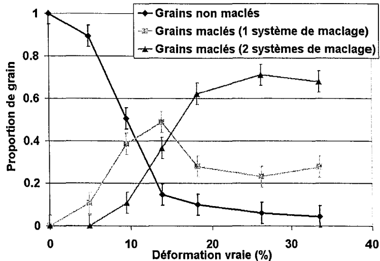
Figure IV.13 : Évolution de la proportion de grains non maclés, ou maclés avec 1 ou 2 systèmes de maclage activés. Cette mesure a été réalisée en microscopie optique sur la nuance 22Mn0,6C-GG après attaque.
