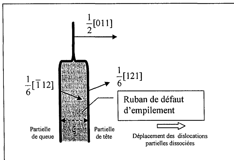
Figure I.8 : Représentation schématique de la dissociation d'une dislocation parfaite de type coin en deux dislocations partielles bordant un défaut d'empilement. Définition de la partielle de tête et de queue.
