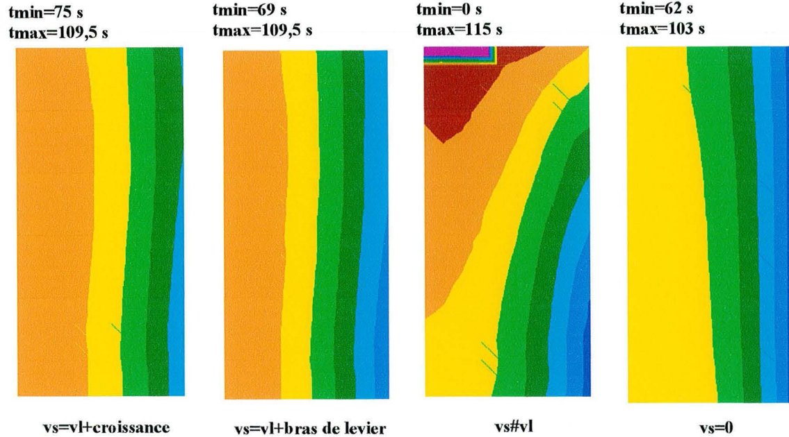
figure V 25 : cartes de distribution du temps local de solidification pour les quatre modèles
