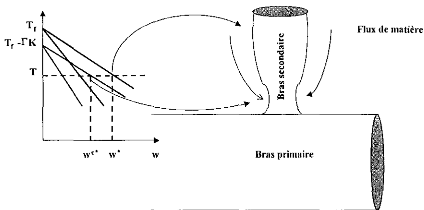
figure 1. 3 : Effets de la courbure interfaciale
