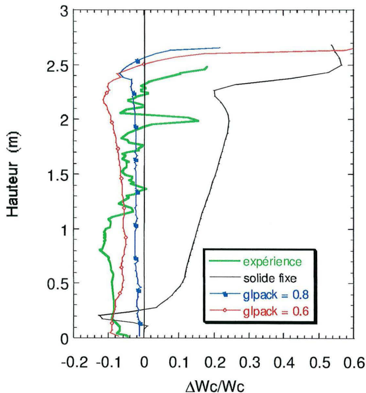
figure V. 37 : Influence de gpack sur la macroségrégation (maillage \Delta x = \Delta y = 3 cm)
