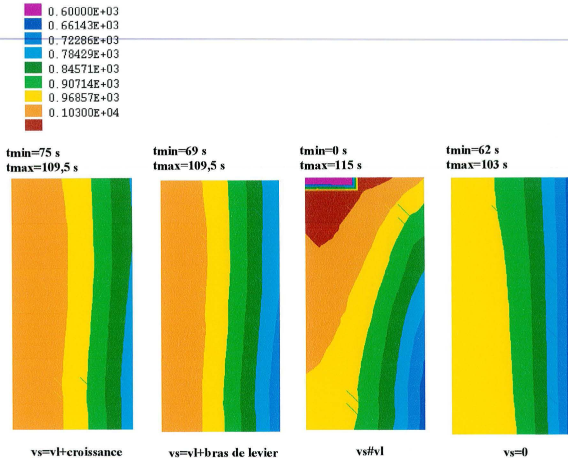
figure V 25 : cartes de distribution du temps local de solidification pour les quatre modèles
