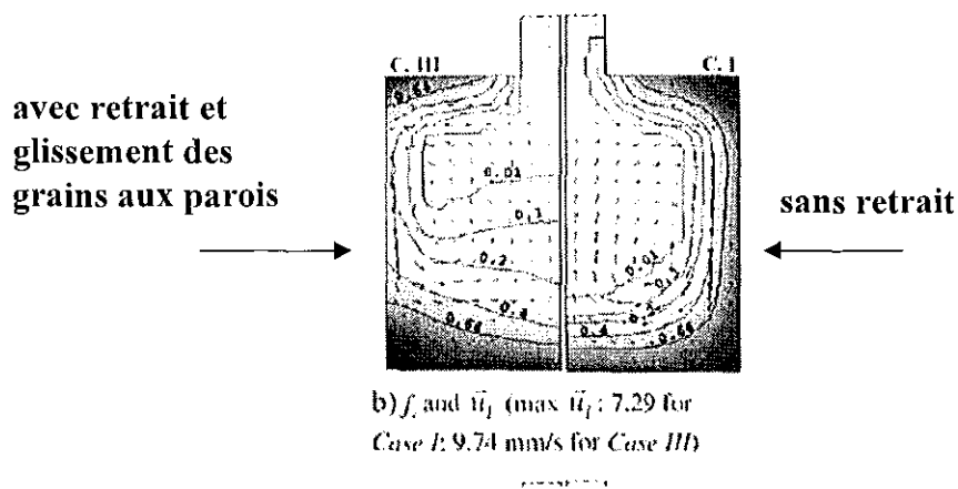
figure II 16 : comparaison des champs de vitesses obtenus après 40 s de calcul [26]
