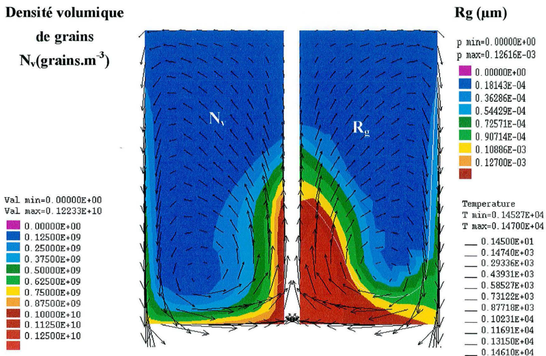
figure V. 5 :cartes de rayon moyen et de la densité volumique de grains (cas : V^s = V^l avec croissance de grains)
