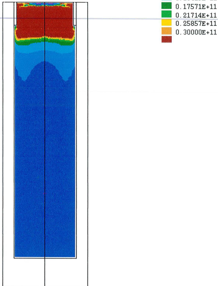
figure V 36 : carte de la densité volumique de grains (maillage \Delta x = \Delta y = 1,5 \text{ cm} )
