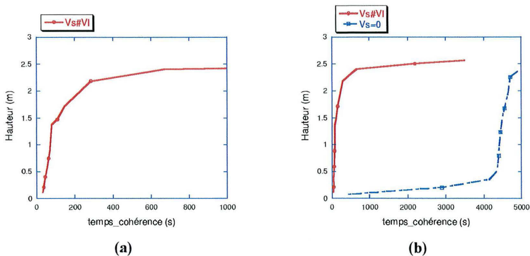
figure V 30 : Montée du front de cohérence au cours du temps
