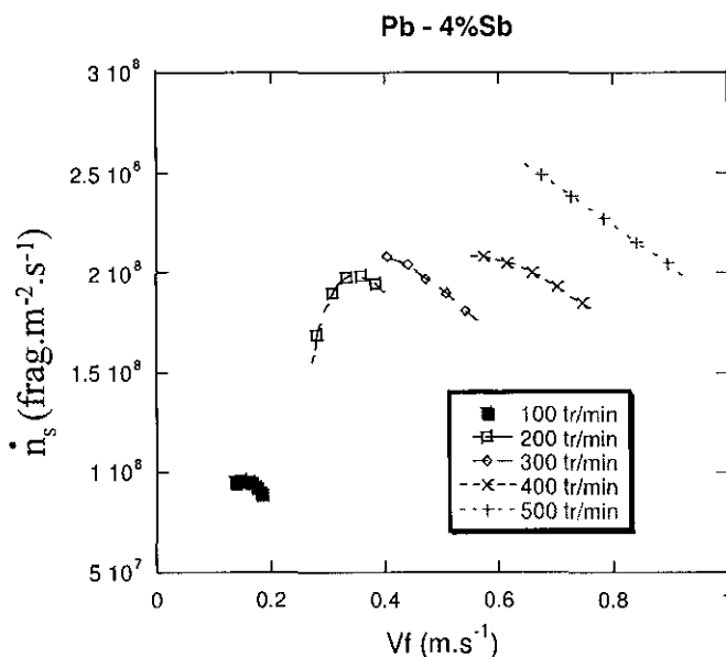
figure III. 13 : Evolution de la densité de flux de fragments détachés du front colonnaire en fonction de la vitesse du fluide devant le front colonnaire
