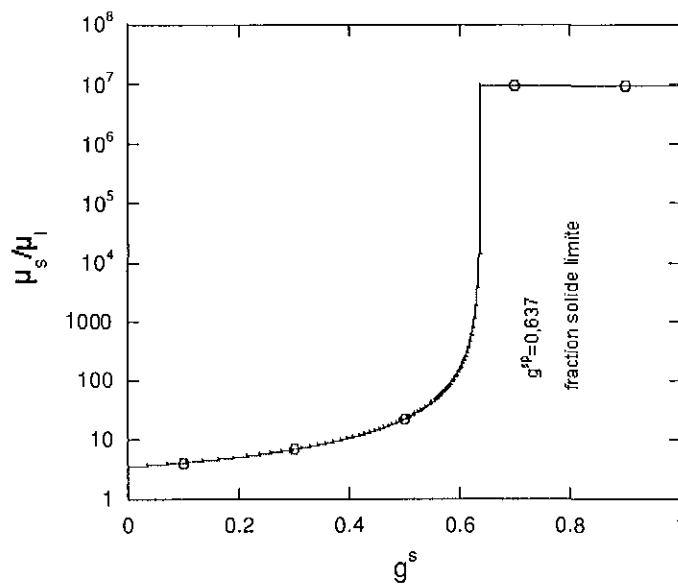
figure II 5 : Evolution en fonction de la fraction solide du rapport de la viscosité de la phase solide à la viscosité du fluide
