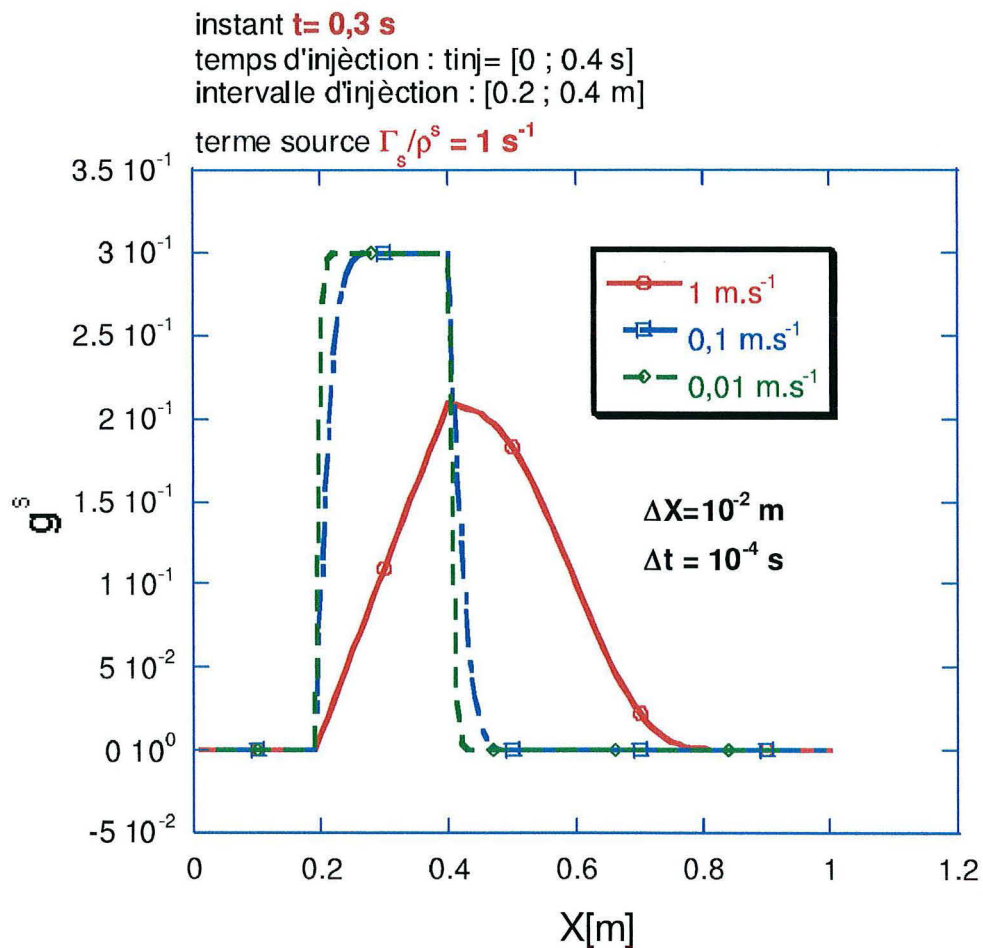
figure IV 11 : Evolution en fonction de la position de la fraction de solide calculée avec la méthode de séparation au temps de calcul t = 0,3 s
