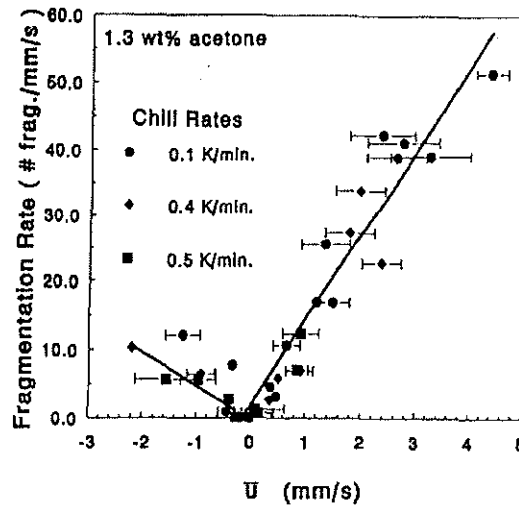
figure I. 10: Evolution de la densité de fragments en fonction de la vitesse estimée du fluide devant le front colonnaire (Paradies et Glicksmann [11])
