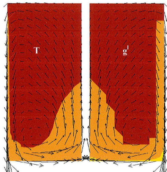
figure V. 3 : cartes de température et de fraction liquide (cas: V^s=V^l , bras de levier)
