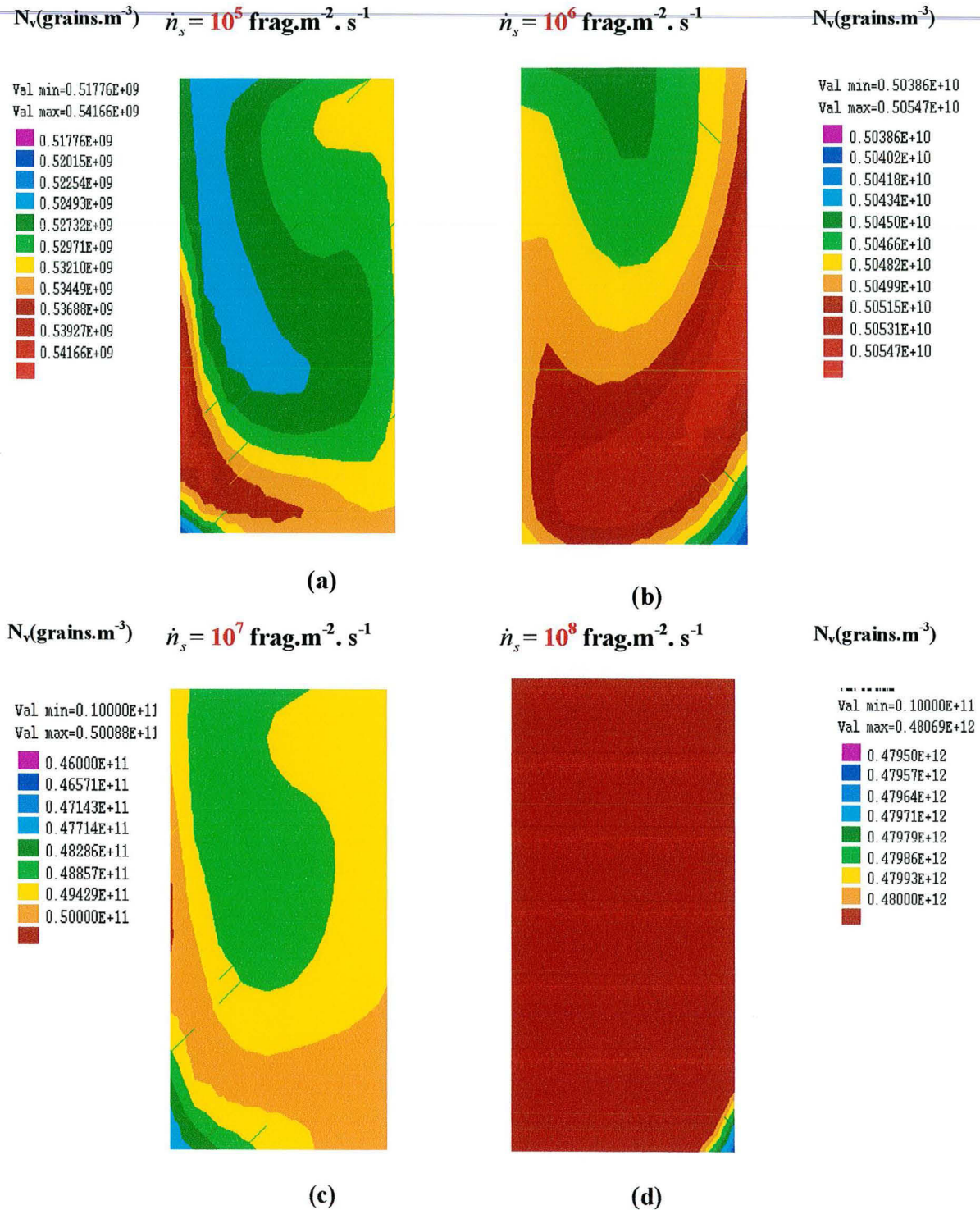
figure V 14 : cartes de densité volumique de grains à la fin de la solidification
