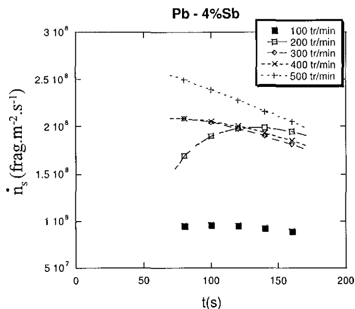
figure III. 12 : Evolution au cours du temps de la densité de flux de fragments détachés du front colonnaire
