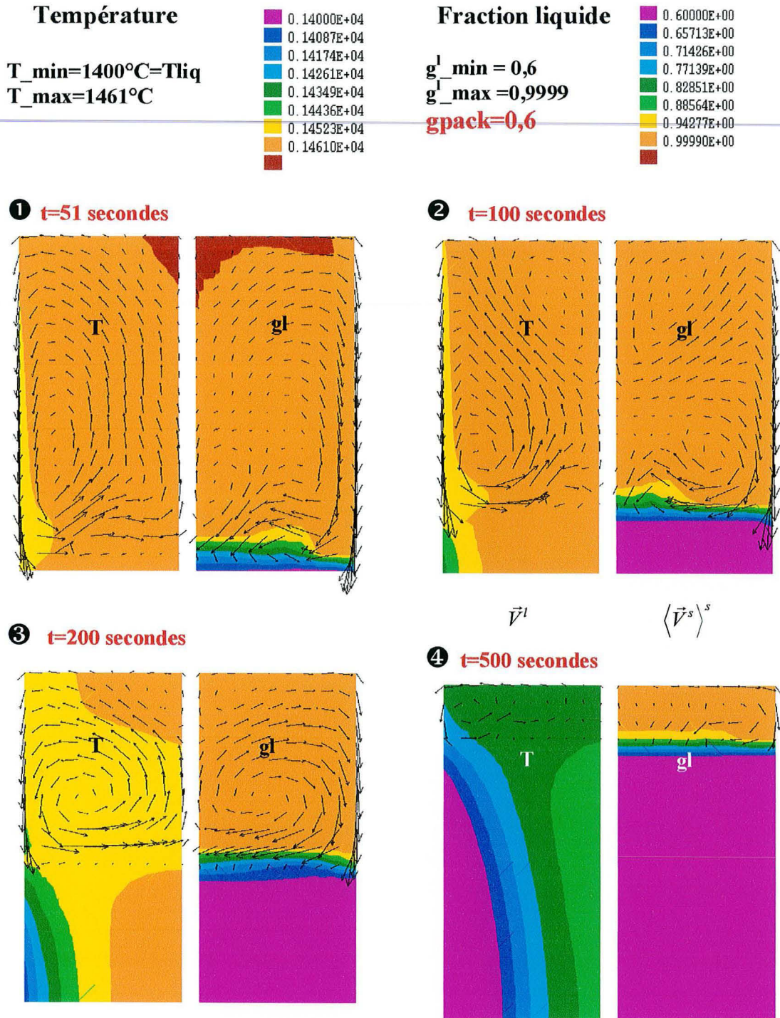
figure V. 20 : Cartes de température et de fraction de liquide pendant la solidification. Les champs de vitesse correspondent à la vitesse intrinsèque de la phase solide sur la partie droite du domaine et à la vitesse moyenne débitante de la phase liquide sur la partie gauche.
