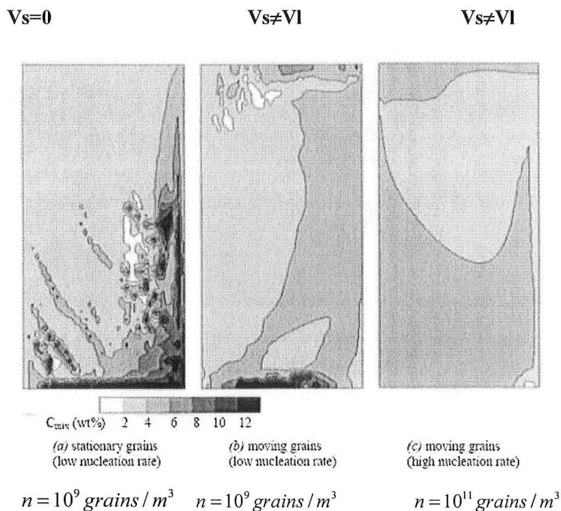
figure II. 9 : cartes finales de la macroségrégation [25]
