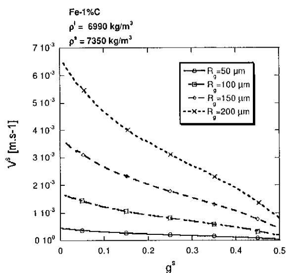
figure IV 3 : Evolution de la vitesse de chute de grains sphériques de taille donnée en fonction de la fraction de solide
