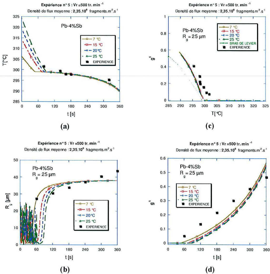
figure III. 23 :Influence de la surchauffe sur l'évolution de population de cristallites dans le liquide
