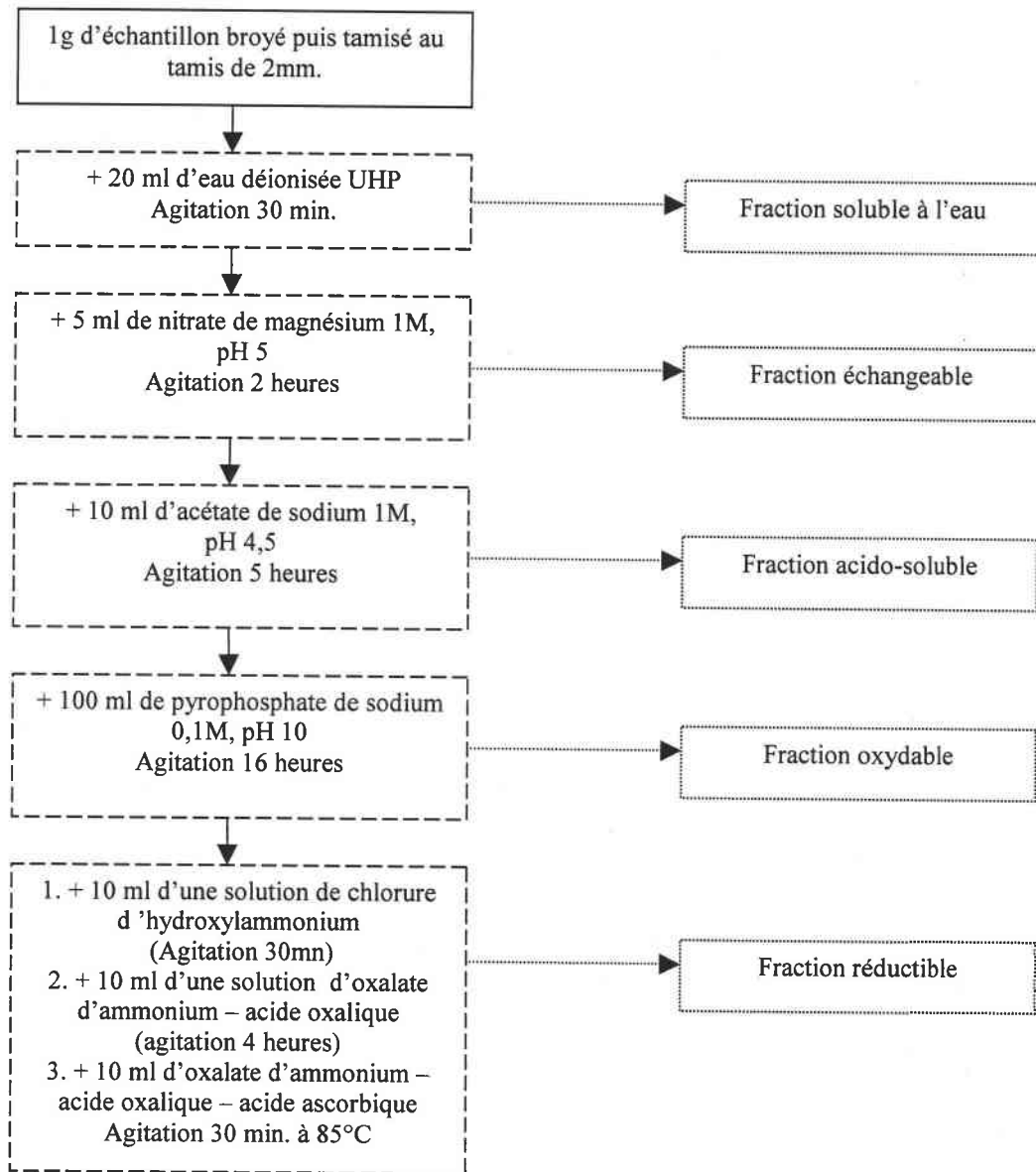
Figure II-34: Principe de l'extraction séquentielle en cascade. Après chaque extraction, le résidu de sédiments est récupéré, puis séché à l'étuve à 60°C jusqu'à masse constante
