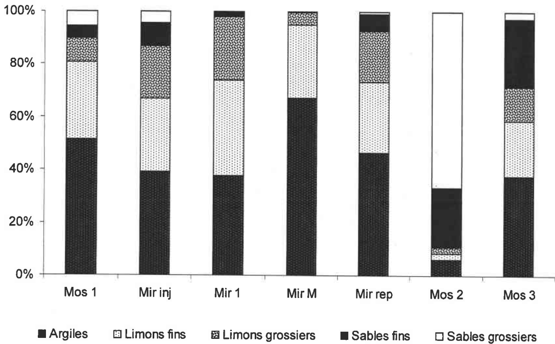
Figure III-38 : Composition granulométrique des différents échantillons de sédiments analysés. Argiles (0 – 2 µm), limons fins (2 – 20 µm), limons grossiers (20 – 50 µm), sables fins (50 -200 µm), sables grossiers (200 – 2000µm).
