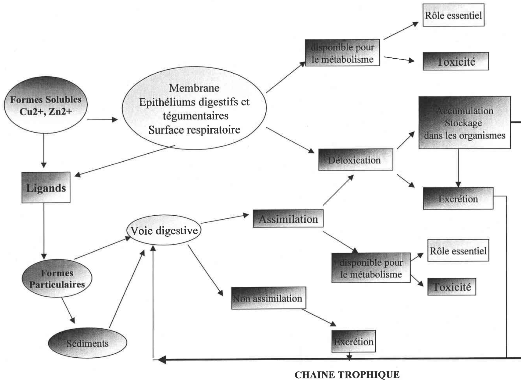
Figure I-14 : Schéma simplifié de la circulation des métaux dans les compartiments biotiques.
