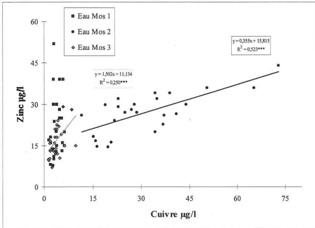
Figure III-13 : Comparaison de la relation linéaire (coefficient de corrélation r de Pearson) des concentrations en cuivre et en zinc dans l'eau brute ( \mu\text{g/l} ) aux stations Moselle (Mos1, Mos2 et Mos3).
