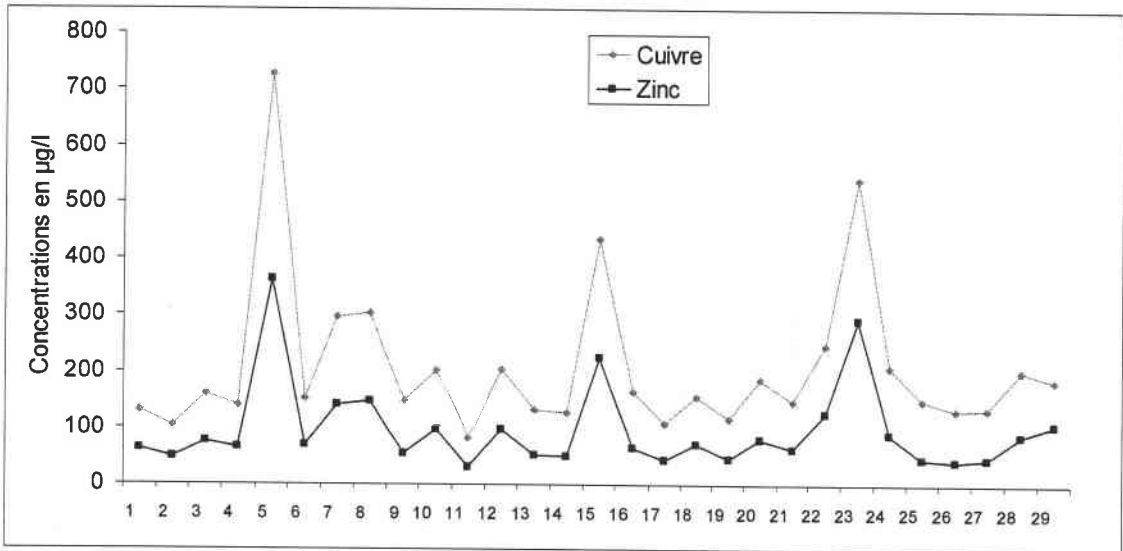
Figure III-5 : Evolution journalière des concentrations moyennes (n=59) en cuivre et en zinc en \mu\text{g/l} dans l'eau brute de la station C2 en juin 2001
