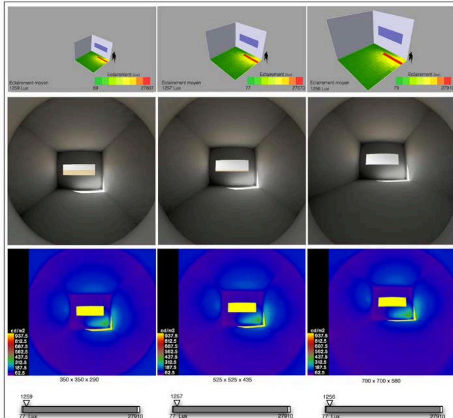
Fig 33. Influence de l'échelle de l'espace architectural sur comportement lumineux
