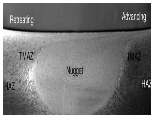
FIGURE 1.9 – Coupe d'une soudure sur un alliage d'aluminium 7075Al-T651 (Référence : [82])
