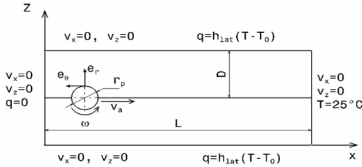
FIGURE 3.1 – Dimensions du domaine d'étude et conditions aux limites
