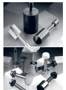
Quelques géométries utilisées sur un rhéomètre.
