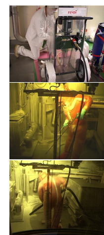
Quelques images d'un essai de décontamination de cellule blindée par gels.
