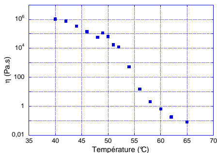
FIGURE 4.23 – Viscosité en fonction de la température pour un gel ι carraghénane 2% dans l'eau.
