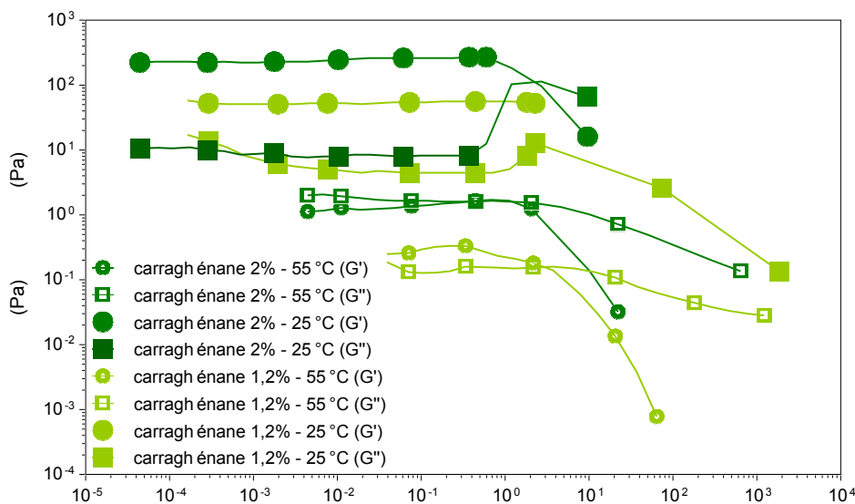
FIGURE 4.25 – Évolution des modules viscoélastiques en fonction de la déformation ( \omega = 1 \text{ rad.s}^{-1} ) pour des gels ι carraghénane 2% wt. (vert sombre) et 1,2% wt. (vert clair) dans l'eau, à 25°C (symboles pleins) et 55°C (symboles creux).
