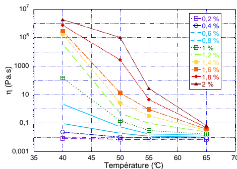
FIGURE 4.24 – Viscosité en fonction de la température pour différents gels ι carraghénane dans l'eau.
