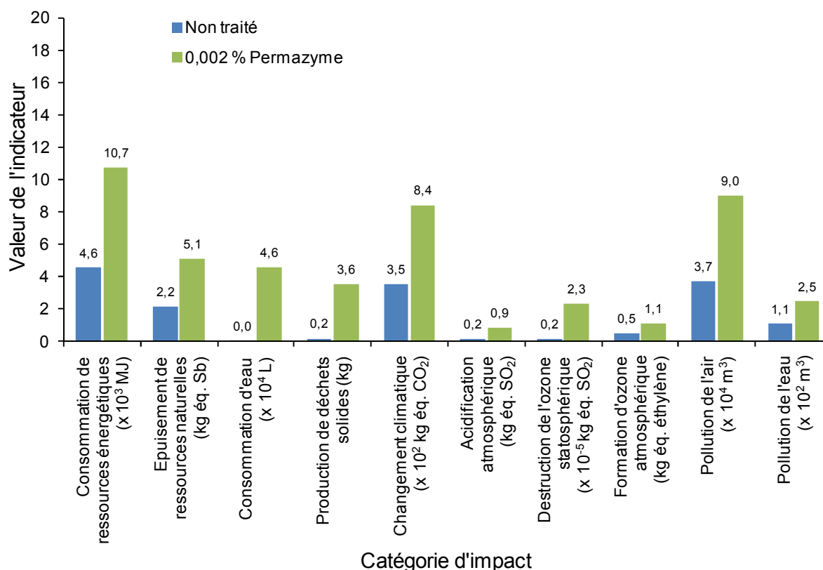
Figure IV.5 : Comparaison des impacts environnementaux pour le traitement à 0,002 % de Permazyme et le compactage du sol non traité à l'énergie Proctor modifiée.
