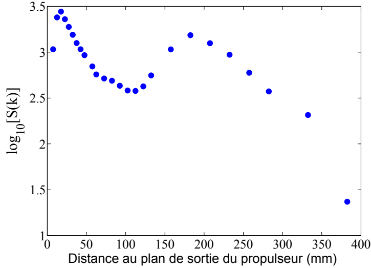
Figure 1.6: Variation du logarithme en base 10 du facteur de forme dans la direction \alpha = 0^\circ avec la distance axiale par rapport au plan de sortie du propulseur. Le nombre d'onde k est fixe et vaut 6200 rad/m. Figure reproduite à partir de [71].
