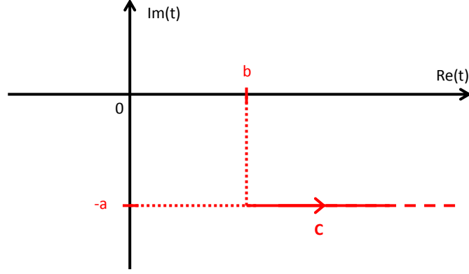
Figure C.2: Contour d'intégration dans le plan complexe de la fonction \operatorname{erfc}(-iz) définie par l'Eq. C.5 pour z = a + ib avec (a, b) \in \mathbb{R}^+ \times \mathbb{R}^+ .
