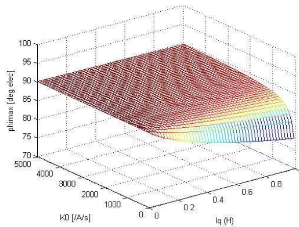
Figure IV-4 : Erreur d'estimation initiale maximale pour l_q variant de 0,01 mH à 1H K_0 allant de 1 à 5000 \text{s}^{-1} \text{A}^{-1} avec : T = 0,1 \text{ ms} , V_{\delta s} = 100 \text{ V} , \tilde{l}_s = 0,1 l_q et \tau = 1 \text{ s} .
