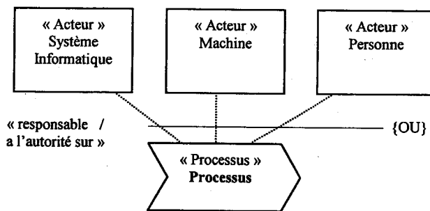
Figure IV.3-10- Notion d'Acteur
