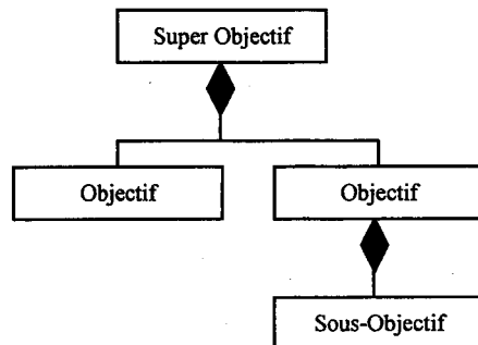
Figure IV.3-4- Décomposition d'objectifs
