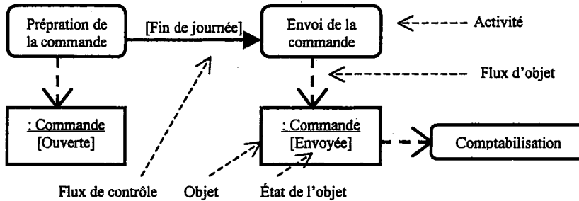
Figure 32 – Diagramme d'activités
