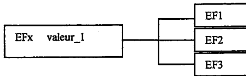
Figure 3 – Déclenchement parallèle
