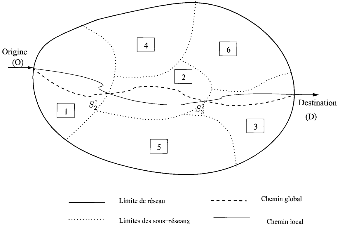
FIG. 3.1 – Représentation de la méthode.
