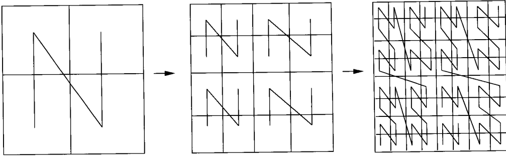
FIG. 3.3 – Une courbe-Z
