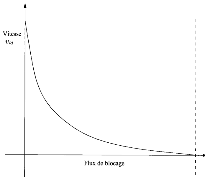
FIG. 4.1 – Vitesse fonction du flux
