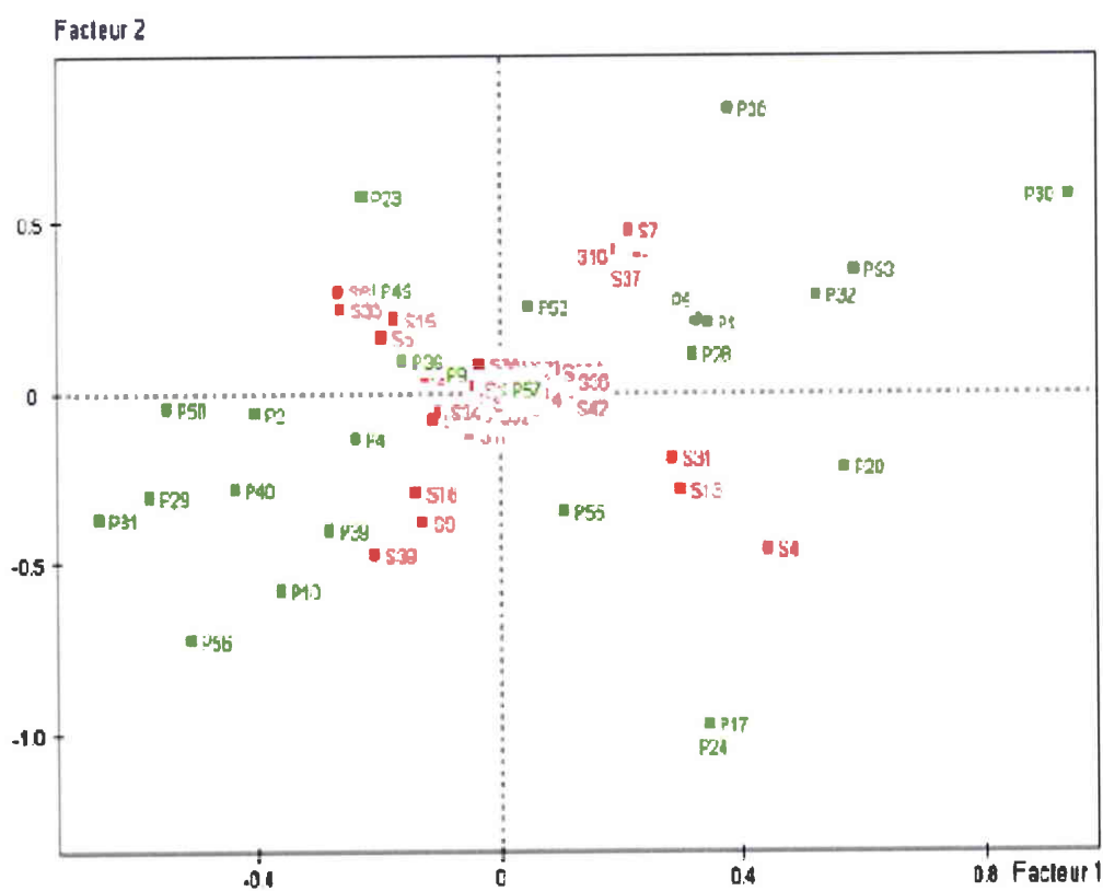
FIG. 5.5 – Un résultat de l'analyse des correspondances multiples
