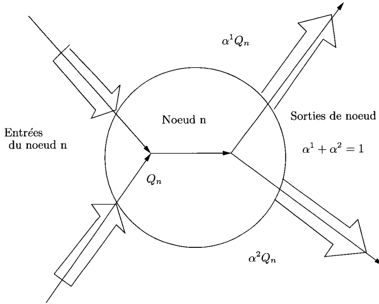
FIG. 4.4 – Modélisation d’un noeud autoroutier
