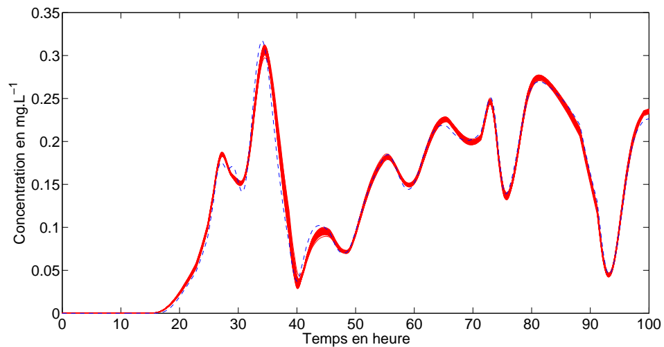
FIGURE 3.7 – Concentration prédite pour une simulation de Monte Carlo de 100 jeux de données (méthode SRIVC-EDP-LPV) pour x = 1, 2 km, les courbes rouges représentent les concentrations prédites, la courbe bleue représente la concentration déterministe
