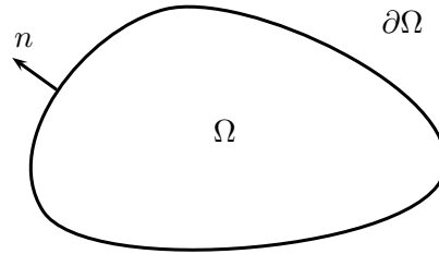
FIGURE 1.2 – Vecteur normal unité orienté vers l'extérieur
