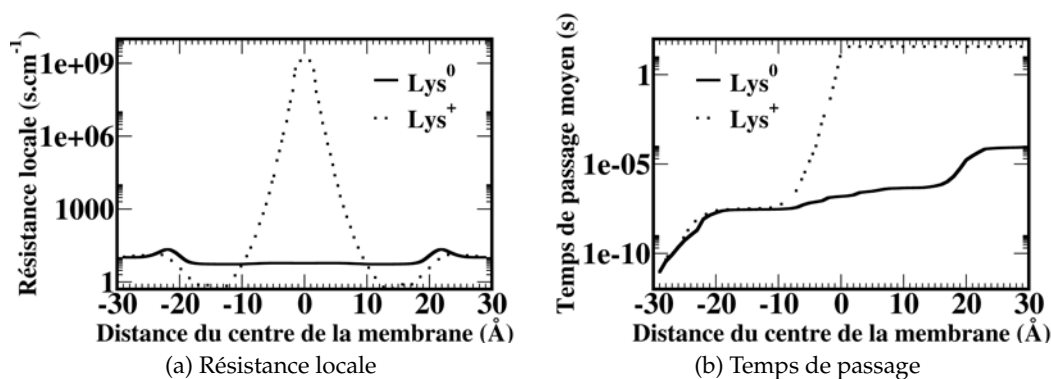
FIGURE 3.8 – Gauche : Résistance locale, correspondant à l'intégrante dans l'équation de la perméation pour le transfert de l'analogue de la lysine depuis un côté de la membrane à l'autre pour la forme protonée (noir – tirets) et déprotonée (noir – plein). Droite : Temps de passage moyen en fonction de la distance pour la forme protonée (noir – tirets) et déprotonée (noir – plein)
