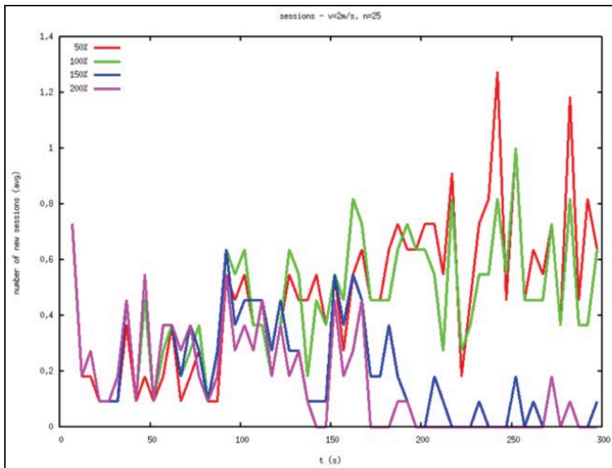
Figure 4-31 : Nombre des nouvelles sessions pour n = 25 nœuds ; V = 2m/s et \xi \in \{50\%, 100\%, 150\%, 200\%\}
