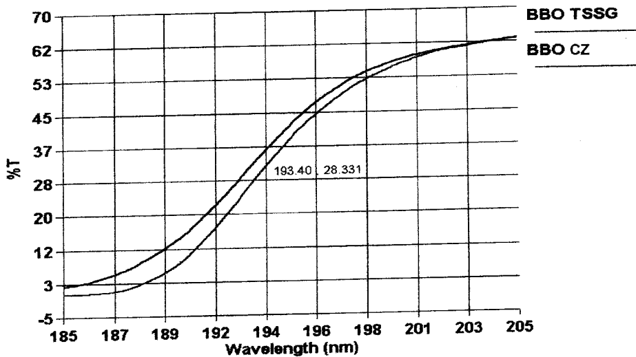
Figure IV.8.a- Spectres de transmission de Cz-BBO synthétisés à Metz et TSSG-BBO synthétisés à Budapest
