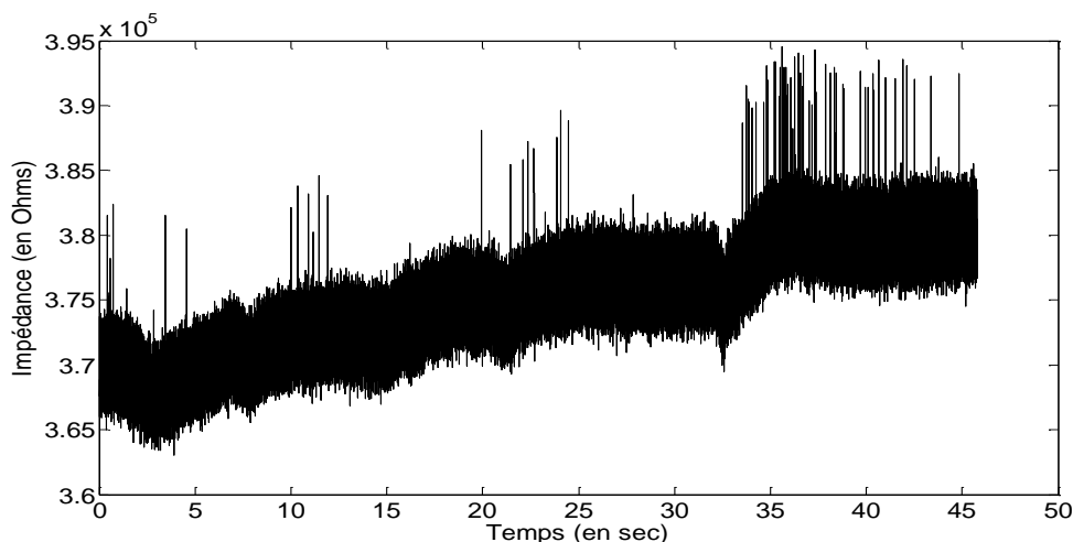
Figure 5-10 Impédance mesurée au cours du temps lors du passage de particules à 100kHz. billes de 6 \mu m dans une solution à 0,5S/m
