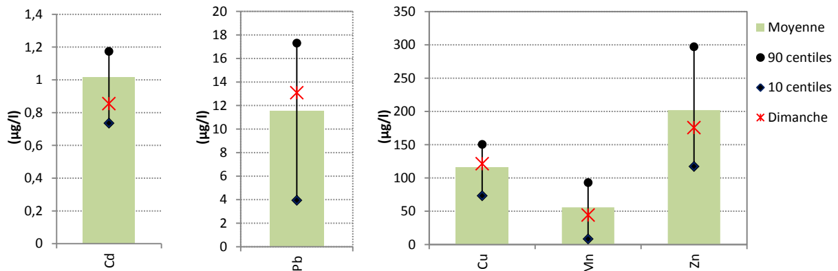
Figure 4.20 : Variabilité des concentrations métalliques journalières d'une journée à l'autre à Clairlieu
