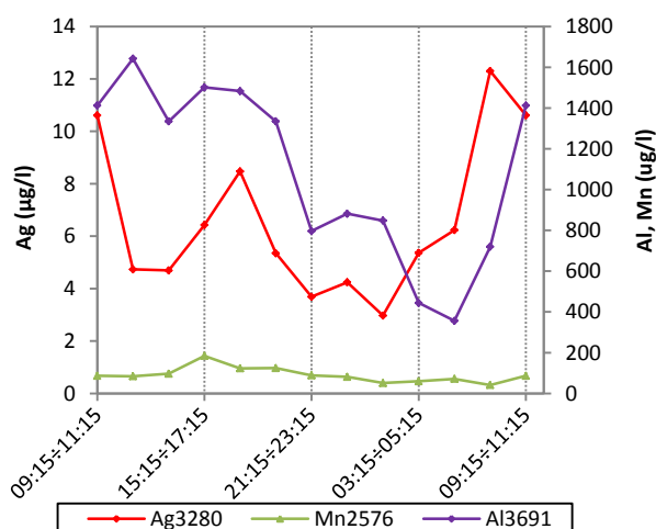
Figure 4.8 : Variations des concentrations des échantillons bruts en métaux lourds pour les sites étudiés.
