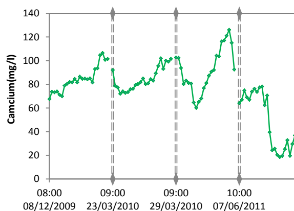
Figures 4.10 (a, b, c et d) : Variations au cours du temps de la concentration en calcium dans les eaux usées de Brabois (a), Clairlieu (b), Fléville-village (c) et STEP de Nancy (d)
