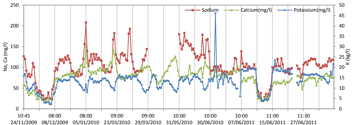
Annexe 10 : Evolutions au cours du temps de différents paramètres mesurés sur des échantillons prélevés à STEP de Nancy
