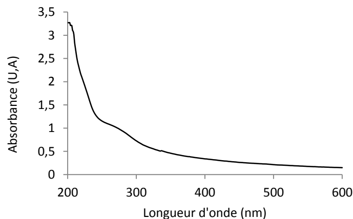
Figure 2.11 : Spectre d'absorption UV-visible de l'eau usée à la STEP Maxéville 24/10/2011
