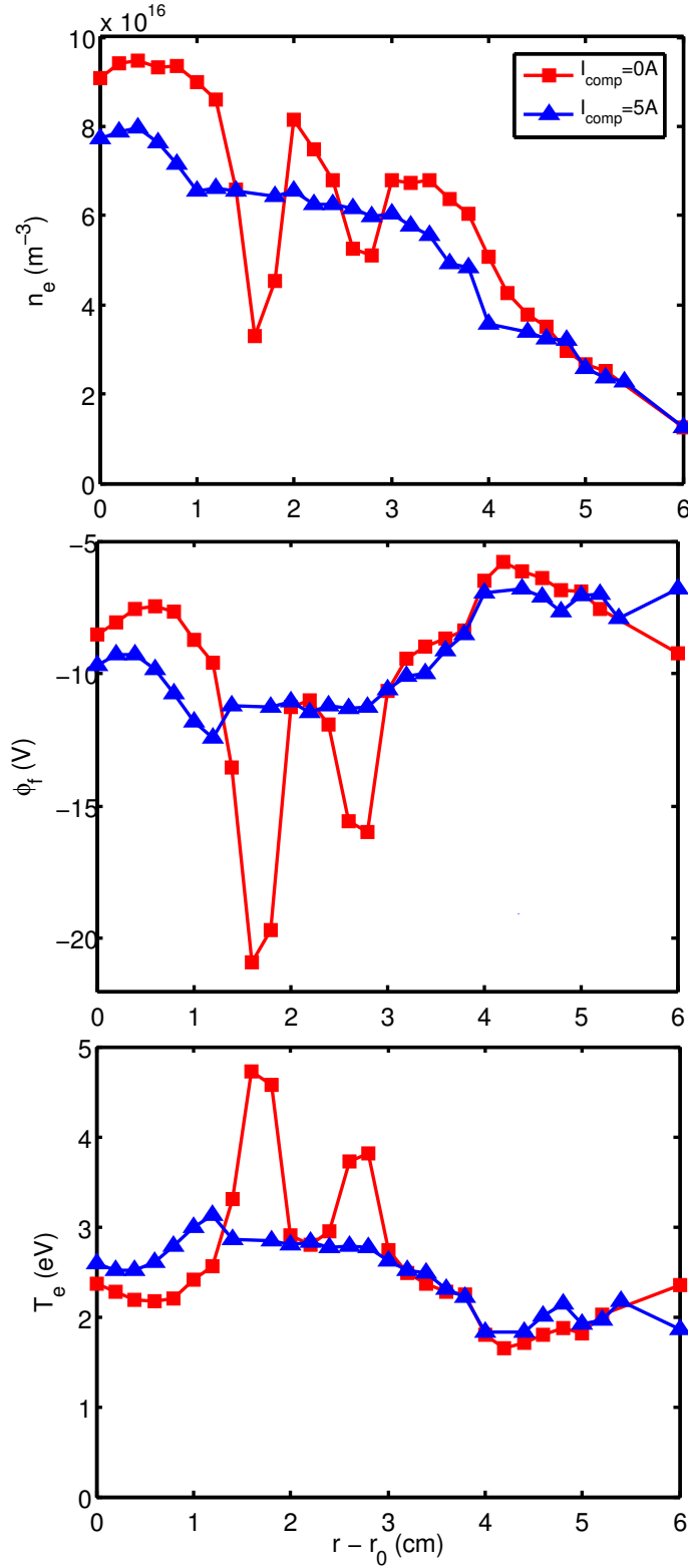
Figure 2.13: Profils de densité, potentiel flottant et température électronique pour deux intensités de courant de compensation I_{\text{comp}} . Les paramètres expérimentaux sont : B = 57 \text{ mT} , P_{\text{argon}} = 4 \times 10^{-4} \text{ mbar} , V_{\text{ac}} = 25 \text{ V} , V_{\text{fil}} = 18 \text{ V} , d_{\text{limiteur}} = 15 \text{ cm} , absence de grille à l'entrée de la colonne.
