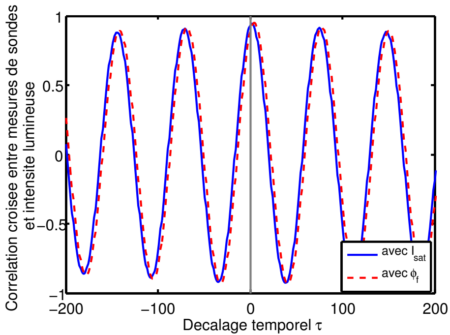
Figure 5.9: Corrélation croisée entre intensité lumineuse enregistrée sur le pixel situé au niveau de la sonde et le courant de saturation ionique(bleu), respectivement le potentiel flottant(tirets rouges).
