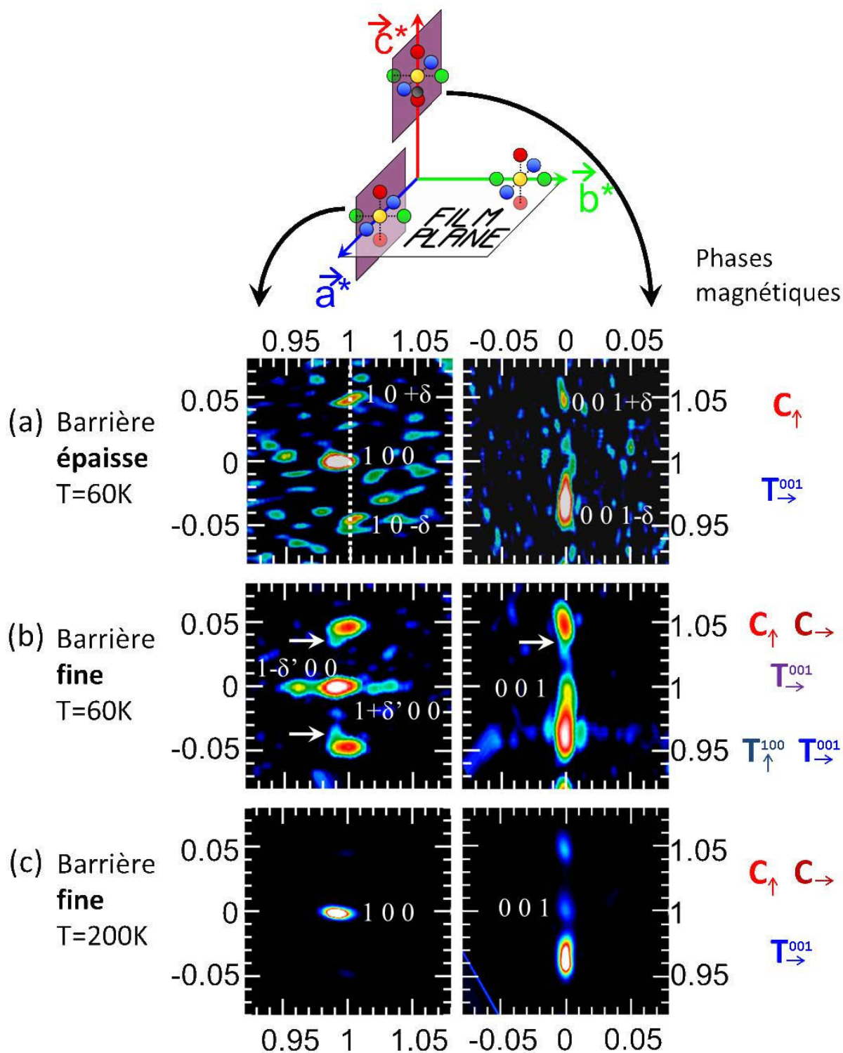
FIGURE 18.4 – Cartographies obtenues par diffraction de neutrons sur une tricouche à barrière épaisse à 60 K (Figures a et b) et à barrière fine (Figures b et c) à 60 K et 200 K, coupes (101) autour du noeud 100 et coupes (010) autour du noeud 001 du réseau réciproque du Cr. Les coordonnées sont données en unités de réseau réciproque. Les traits pointillés blancs soulignent le décalage du pic commensurable par rapport aux pics satellites et les flèches indiquent les pics satellites 10 \pm \delta'' et 001 + \delta'' .
