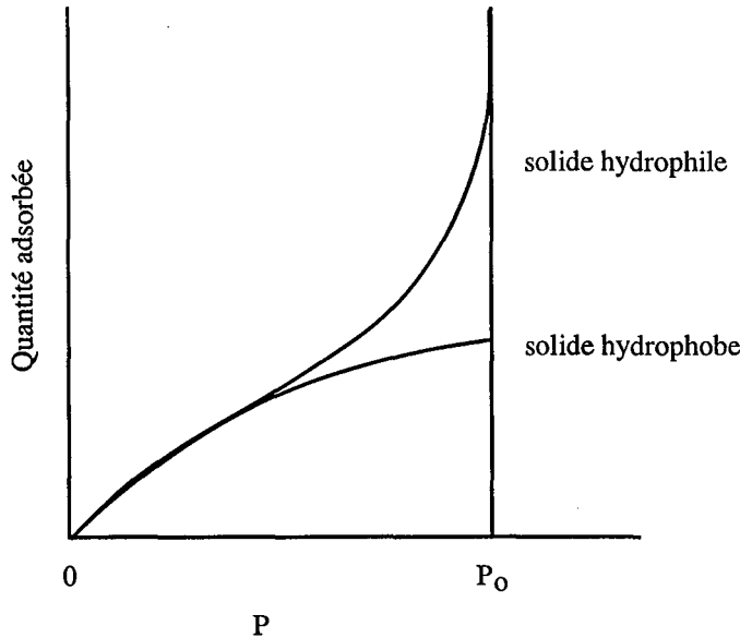
Figure V.8 : Adsorption schématique d'eau et mouillabilité des solides
