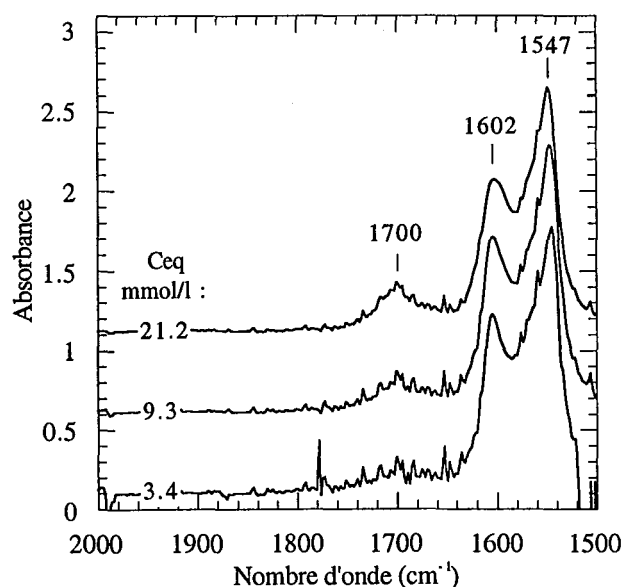
Figure IV.63 : Vibrations des carbonyles normées à la concentration de trisiloxane. Système Hydrates cimentaires / Anhydride
