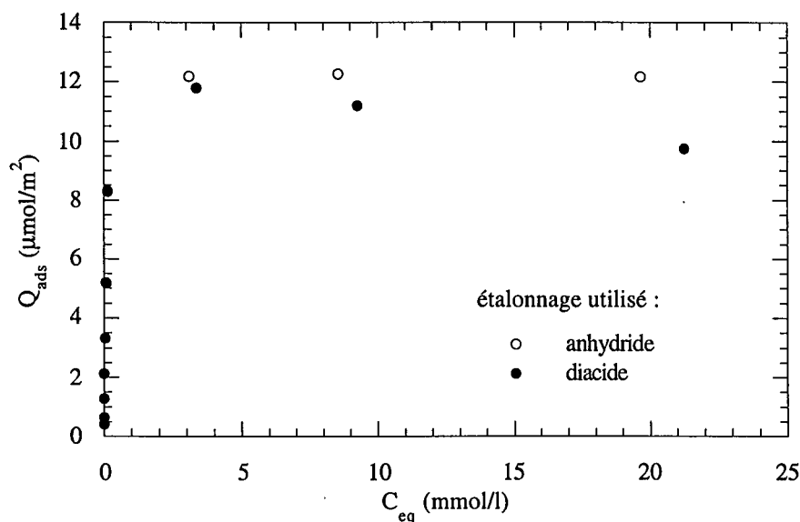
Figure IV.49 : Corrections de l'isotherme d'adsorption de l'anhydride sur les hydrates cimentaires
