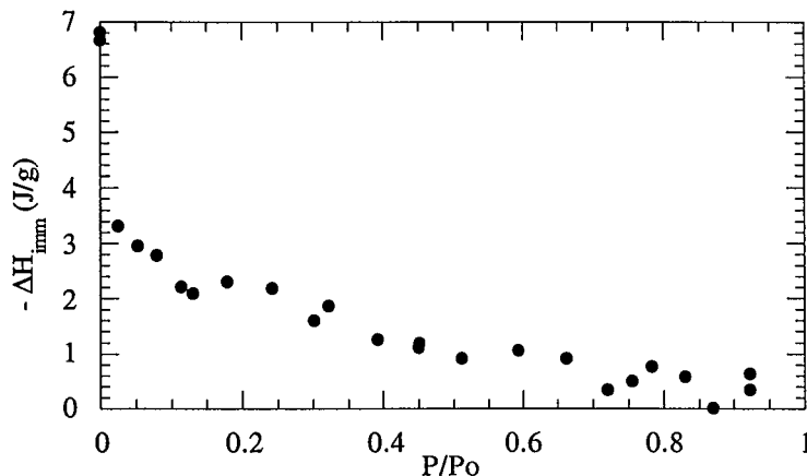
Figure V.50 : Évolution de la chaleur d'immersion dans l'eau en fonction de la pression relative de précouvreurment en vapeur d'eau sur le carbonate hydrofugé.
