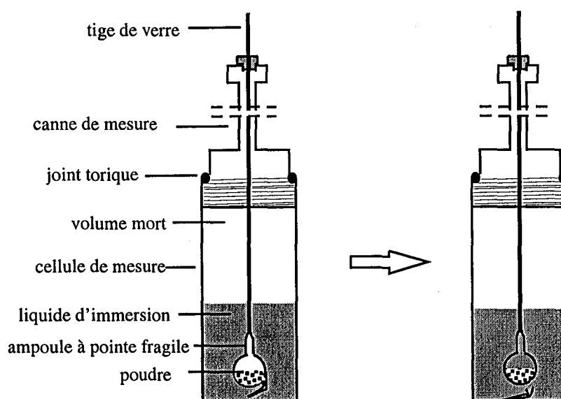
Figure II.5 : Principe de l'immersion
