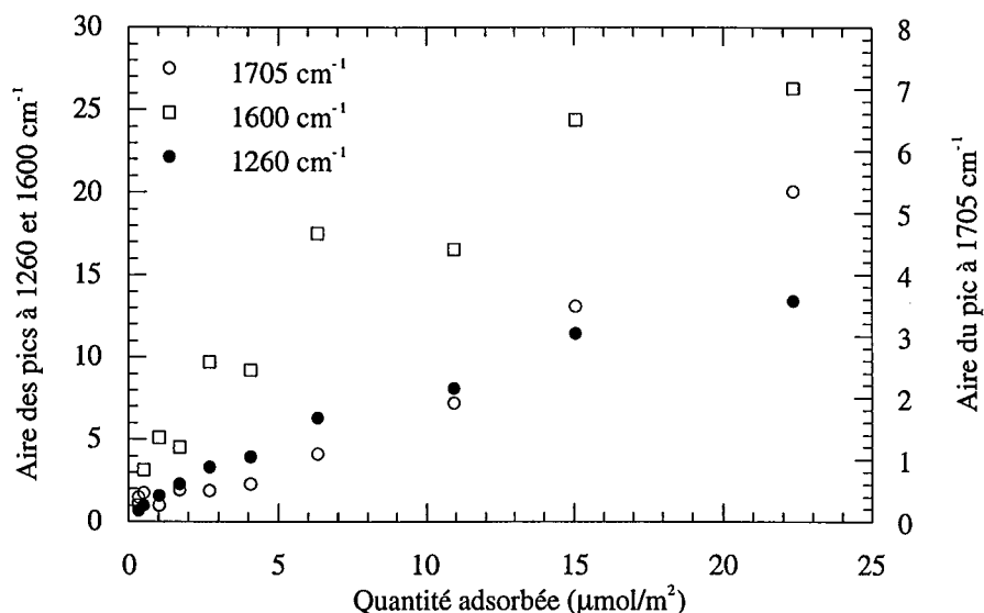
Figure IV.62 : Aire des pics à 1705, 1600 et 1260 \text{cm}^{-1} des spectres en réflexion diffuse en fonction de la quantité de trisiloxane adsorbée. Système carbonate / diacide.
