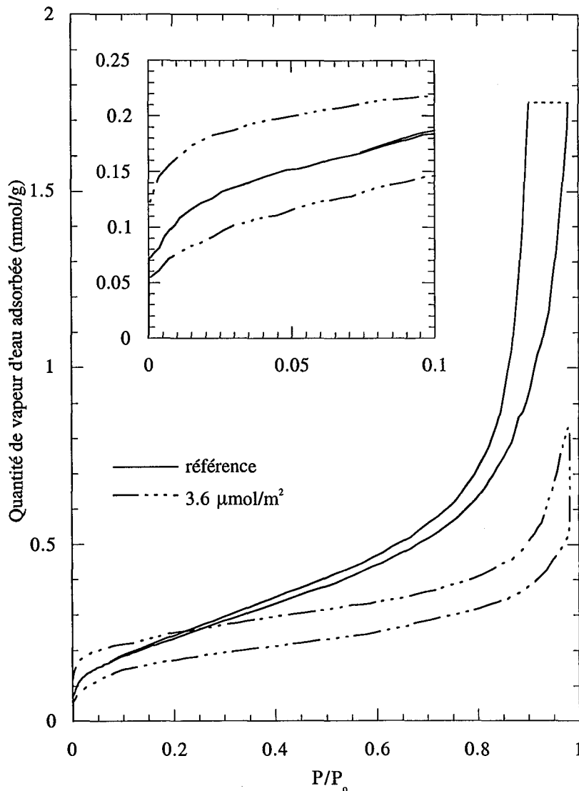
Figure V.22 : Comparaison des isothermes d'adsorption-désorption de l'échantillon de référence et du carbonate recouvert de 3.6 \mu\text{mol}/\text{m}^2 .
