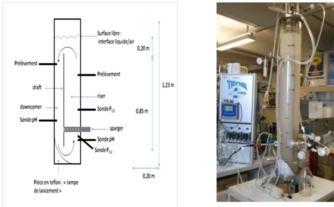
Figure II-4. Coupe longitudinale et photographie du réacteur de type airlift utilisé au cours de ce travail.
