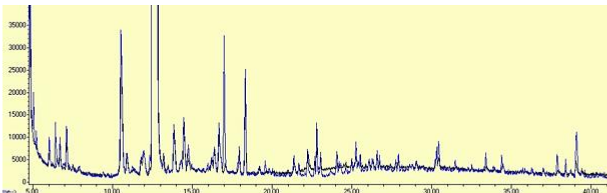
Figure III-8. Chromatogramme (0-40 minutes) GC-FID d'huiles de pyrolyse d'épicéa produites au four à image. Trait bleu T(\text{gazéifieur}) = 850^\circ\text{C} ; trait noir T(\text{gazéifieur}) = 700^\circ\text{C} .
