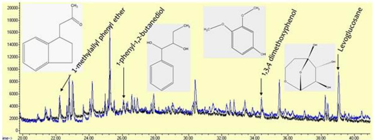
Figure III-10. Chromatogramme (20-40 minutes) GC-FID d'huiles de pyrolyse de hêtre produites au four à image. Trait bleu T(\text{gazéifieur}) = 850^{\circ}\text{C} ; trait noir T(\text{gazéifieur}) = 700^{\circ}\text{C} .
