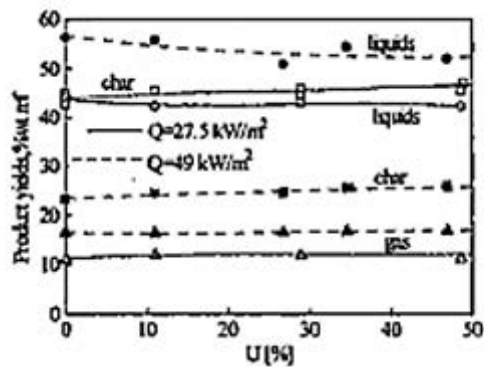
Figure I-34. Rendements massiques (par rapport à la masse sèche) en charbon, gaz et liquides de pyrolyse en fonction du pourcentage d'humidité du bois de hêtre pour des flux radiatifs de 27,5 et 49 kW/m 2 [Di Blasi et al, 2000].
