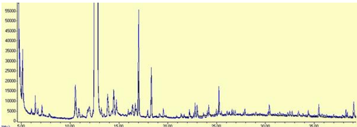
Figure III- 7. Chromatogramme (0-40 minutes) GC-FID d'huiles de pyrolyse de hêtre produites au four à image. Trait bleu T(\text{gazéifieur}) = 850^\circ\text{C} ; trait noir T(\text{gazéifieur}) = 700^\circ\text{C} .
