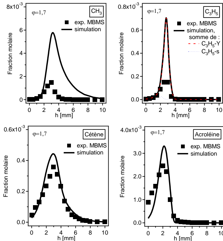
Figure 4.24. Comparaison entre la simulation et l'expérience avec la MBMS (au PC1-Bielefeld) pour quelques espèces réactives mesurées dans la flamme de furane \phi=1,7 .
