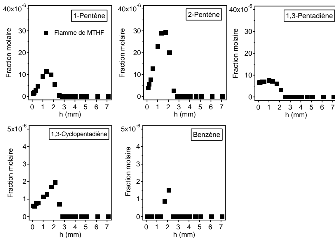
Figure I-5. Profils de fraction molaire des intermédiaires non oxygénés en C 5 -C 6 ( \phi=0,7 ).
