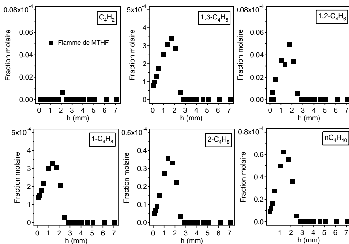
Figure I-4. Profils de fraction molaire des intermédiaires non oxygénés en C 4 ( \phi=0,7 ).
