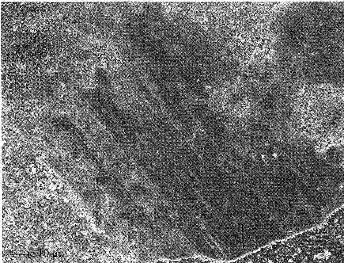
Figure 37 : Image MEB du revêtement \{111\} après frottement contre le disque HSS, sous vapeur d'eau à faible charge (0.2 N)
