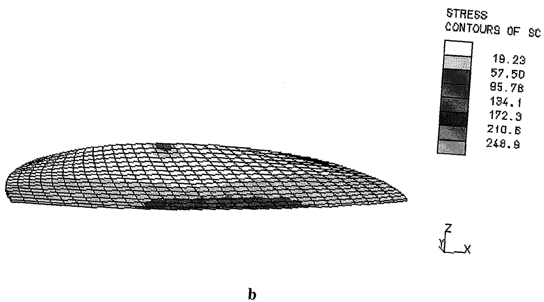
Figure d : Distributions des contraintes (a) normales, (b) de cisaillement après un déplacement de trois pas (30 \mu\text{m} )
