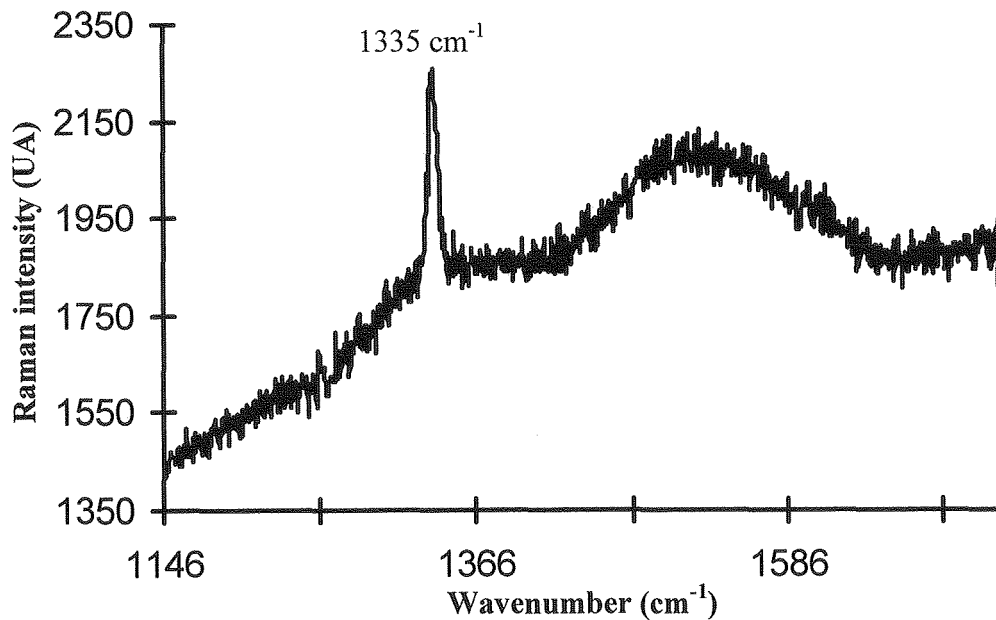
Figure 42 : Spectre Raman du revêtement {100} après frottement sous vapeur d'eau à faible charge (0.2 N)
