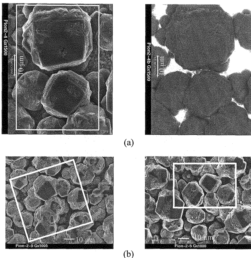
Figure 64 : (a) Images MEB et secondaire des grains éloignés de la zone de travail (b) Images MEB des deux cristaux traités au voisinage de la lunule
