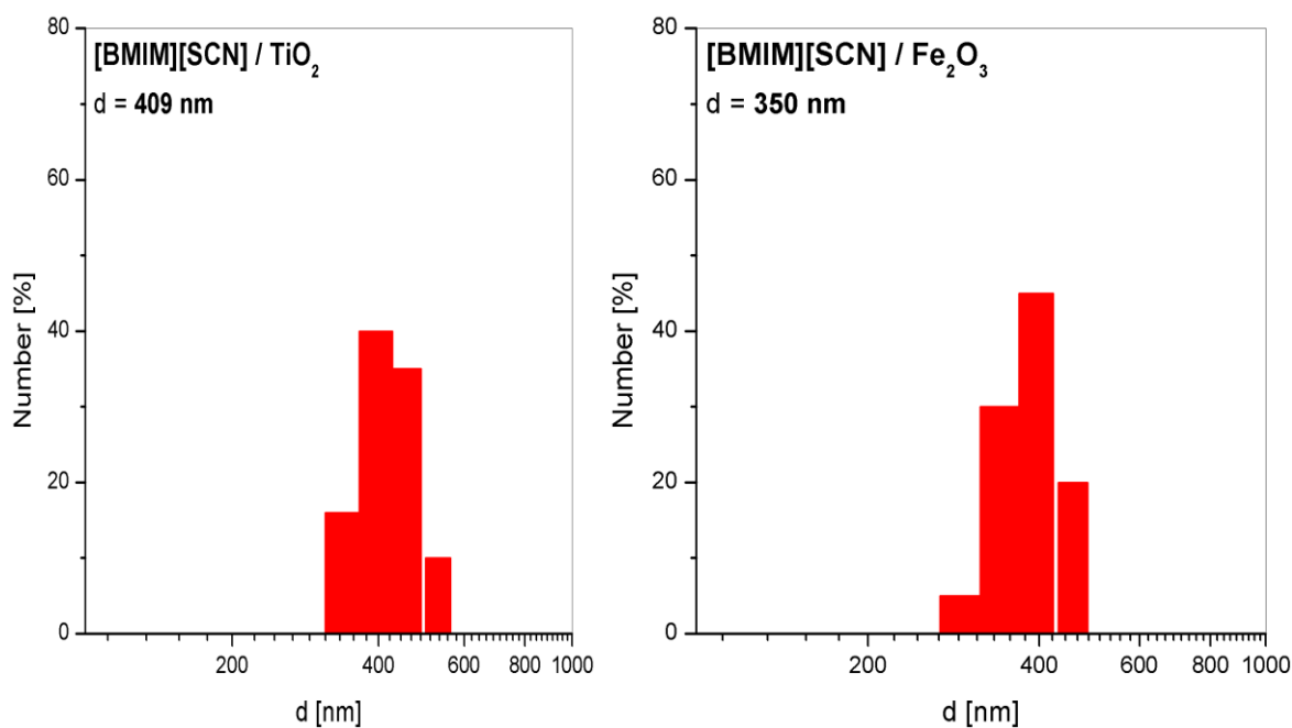
Figure 38- Histogramme de tailles d'agrégats dans [\text{BMIM}][\text{SCN}] de : NPs de \text{TiO}_2 et \text{Fe}_2\text{O}_3
