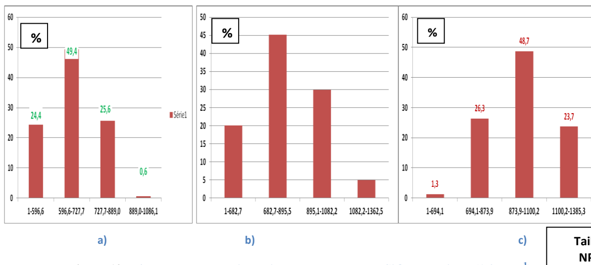
Figure 19- Histogramme de tailles d'agrégats de NPs de SiO 2 dans l'eau (1,0 g L -1 ) :
