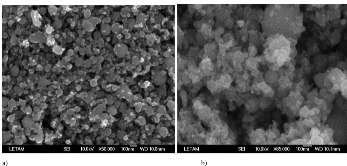
Figure 33- Images MEB de NPs de TiO 2 .
