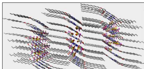
Figure 3- Organisation de C_4C_1 -imPF 6 à sa température de fusion [87].
