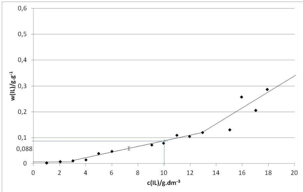
Figure 31- L'isotherme de sorption de [BMIM][Br] par des agrégats de NPs de TiO 2 NPs, w_{LI} (g·g -1 ), en fonction de la concentration de LI ( c_{LI} /g·L -1 ) à T = 298,15 K. Ligne droite entre 2 g·L -1 et 12 g·L -1 représente les données expérimentales avec une déviation standard de +/-0,003 g·L -1 . A la concentration de c_{LI} = 10 g·L -1 , w_{LI} = 0,094 g·g -1 .
