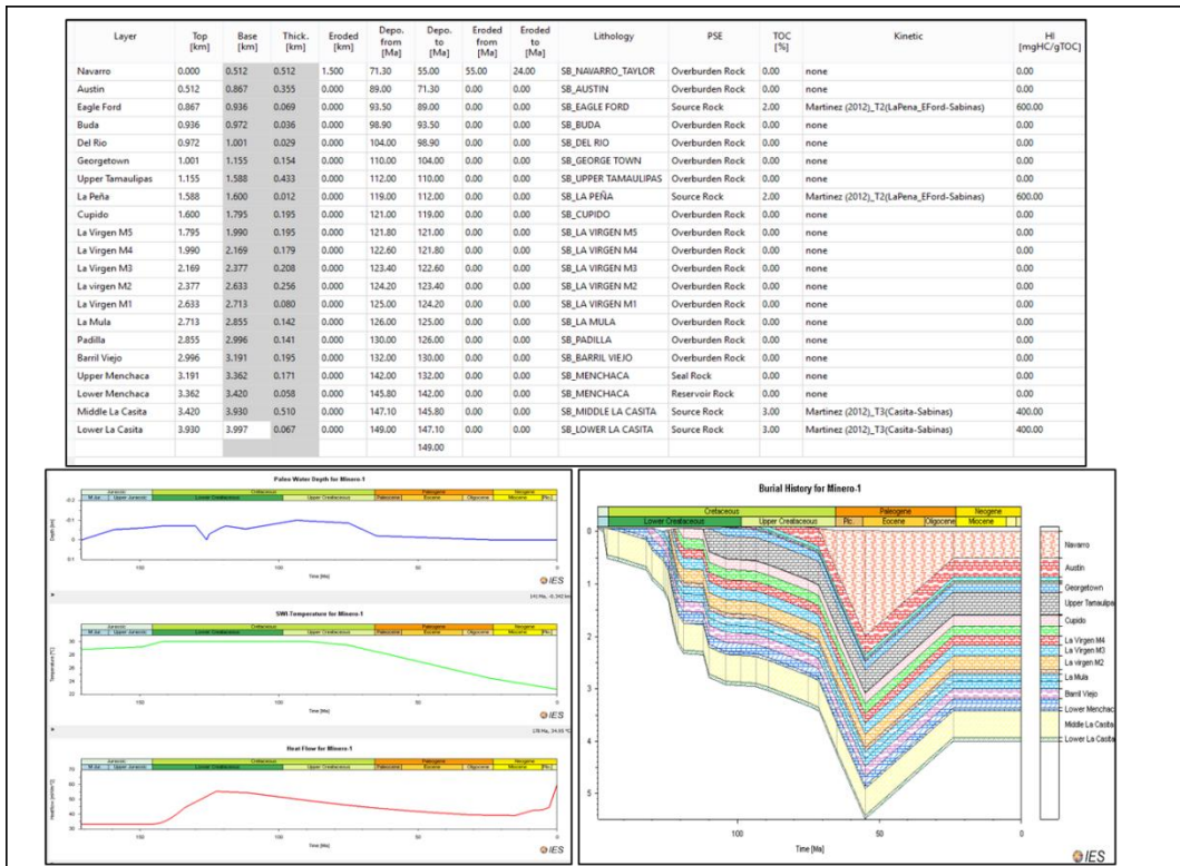
Figura 107. Parámetros de entrada para la calibración térmica del pozo Minero-1.
