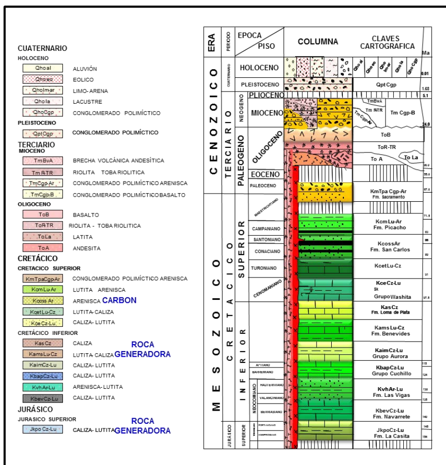
Figura 49. Columna geológica, del área de Ojinaga-Manuel Benavides, con las formaciones del sistema Jurásico superior-Mesozoico, Tomado de Hernández, et al., 2002 (SGM), modificada en este trabajo.
