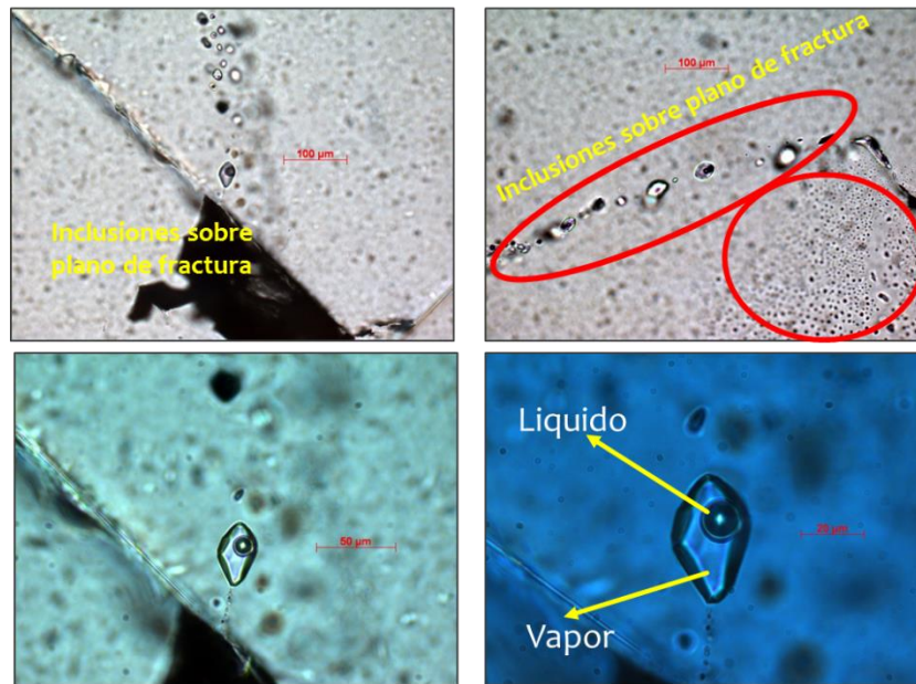
Figura 88. Muestra 1A, inclusiones en un cristal de fluorita, de la zona de la Cuenca de Sabinas, inclusiones de dos fases, agua-vapor sin aceites ni gas.
