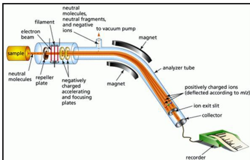
Figura 11. Esquematación del paso de una muestra por los principales componentes de un instrumento de espectroscopia de masas.
