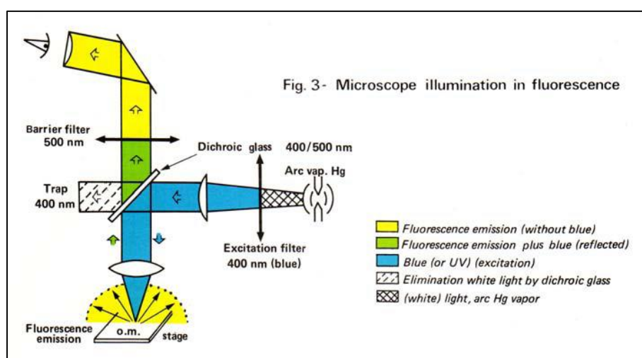
Figura 16. Esquema de un microscopio petrográfico de iluminación en fluorescencia. Tomado de Robert (1983).
