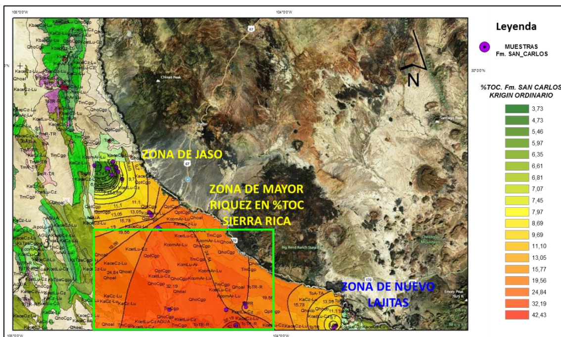
Figura 133. Distribución espacial de valores de carbón orgánico total (%TOC), para la Formación San Carlos en la Cuenca de Chihuahua.
