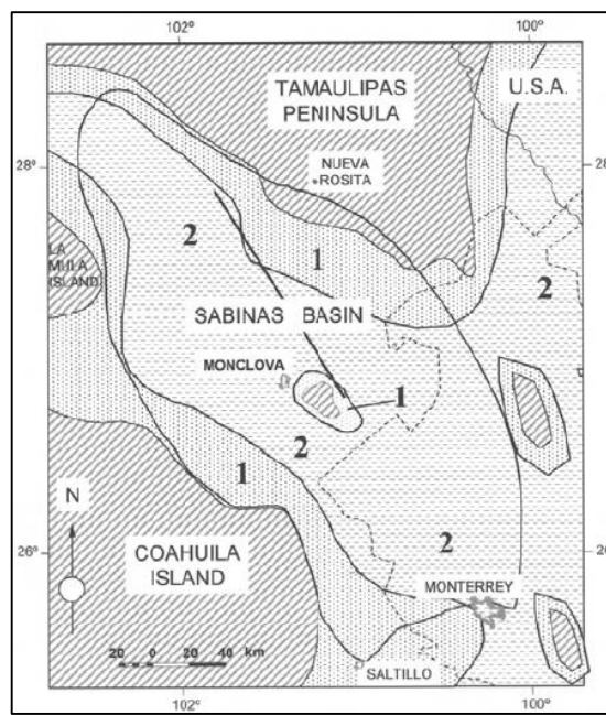
Figura 34. Paleogeografía del Títoniano de la Cuenca de Sabinas. Zonas rayadas indican tierras emergidas. (1) Frente de costa arenosas y (2) facies de lutitas marinas profundas de la formación La Casita, (Eguiluz de Antuñano, 2001).
