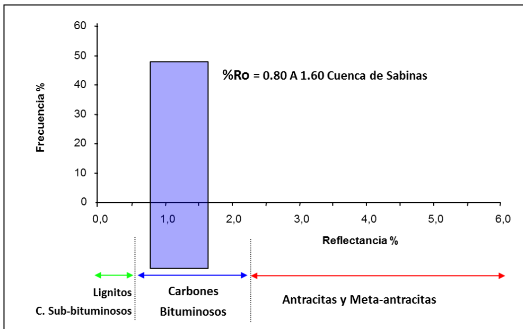
Figura 84. Clasificación de los carbones de la cuenca de Sabinas, únicamente en base a la reflectancia de las muestras analizadas.
