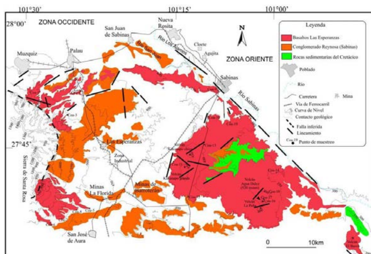
Figura 28. Mapa geológico simplificado del campo volcánico Las Esperanzas. En él solo se resaltan las rocas y depósitos del Terciario tardío y del Cuaternario. En la región occidental la distribución de los derrames de lava sugiere que fueron extravasados por fisuras ubicadas en el borde de la Sierra de Santa Rosa. Los volcanes de la región oriental tienen la morfología de escudos de lava; los puntos de emisión están marcados por conos cineríticos pequeños que aún son fácilmente reconocibles. Nótese que los bordes nororientales de los derrames parecen haberse desviado a lo largo de un alineamiento paralelo al curso actual de los ríos Sabinas y Los Álamos. Tomado de Valdez-Moreno (2001).
