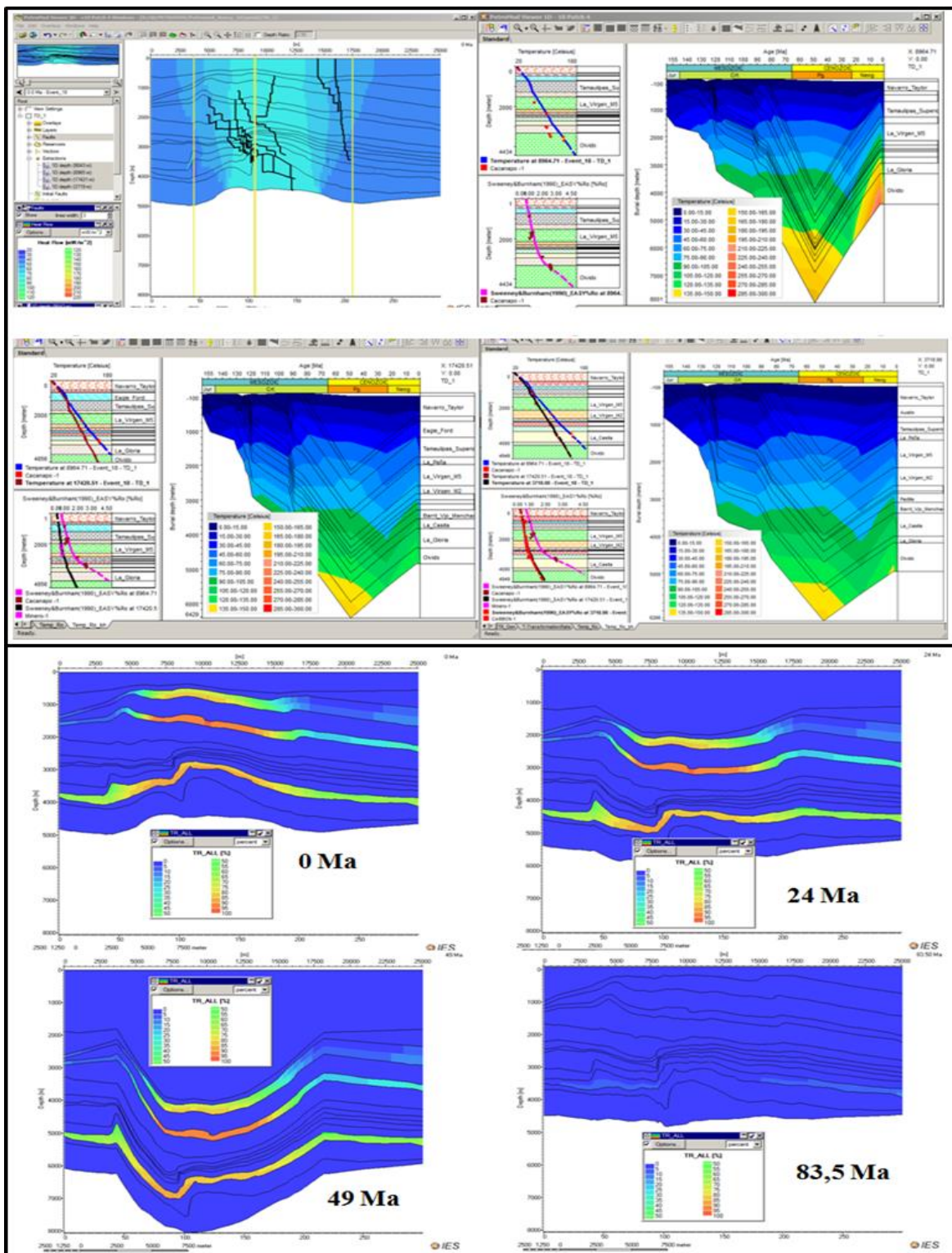
Figura 114. Evolución de la tasa de transformación de las rocas madres con los flujos de calor calibrados en la línea sísmica L-2.
