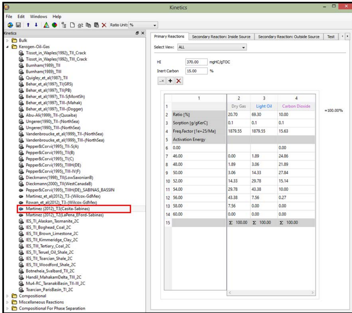
Figura 103. Cinética para la Formación La Casita, utilizada para el modelado de la Cuenca de Sabinas.
