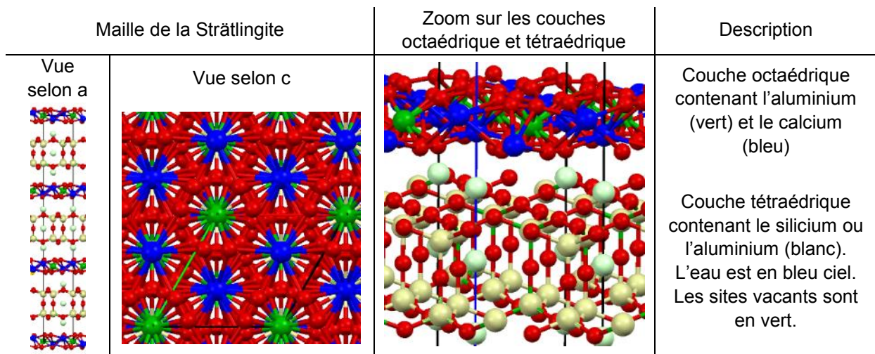
Figures 16. Structure de la strätlingite (Rinaldi et al. , 1990)
