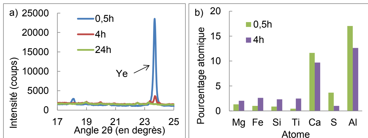
Figures 20. Diffraction (a) et analyse chimique (b) des insolubles
