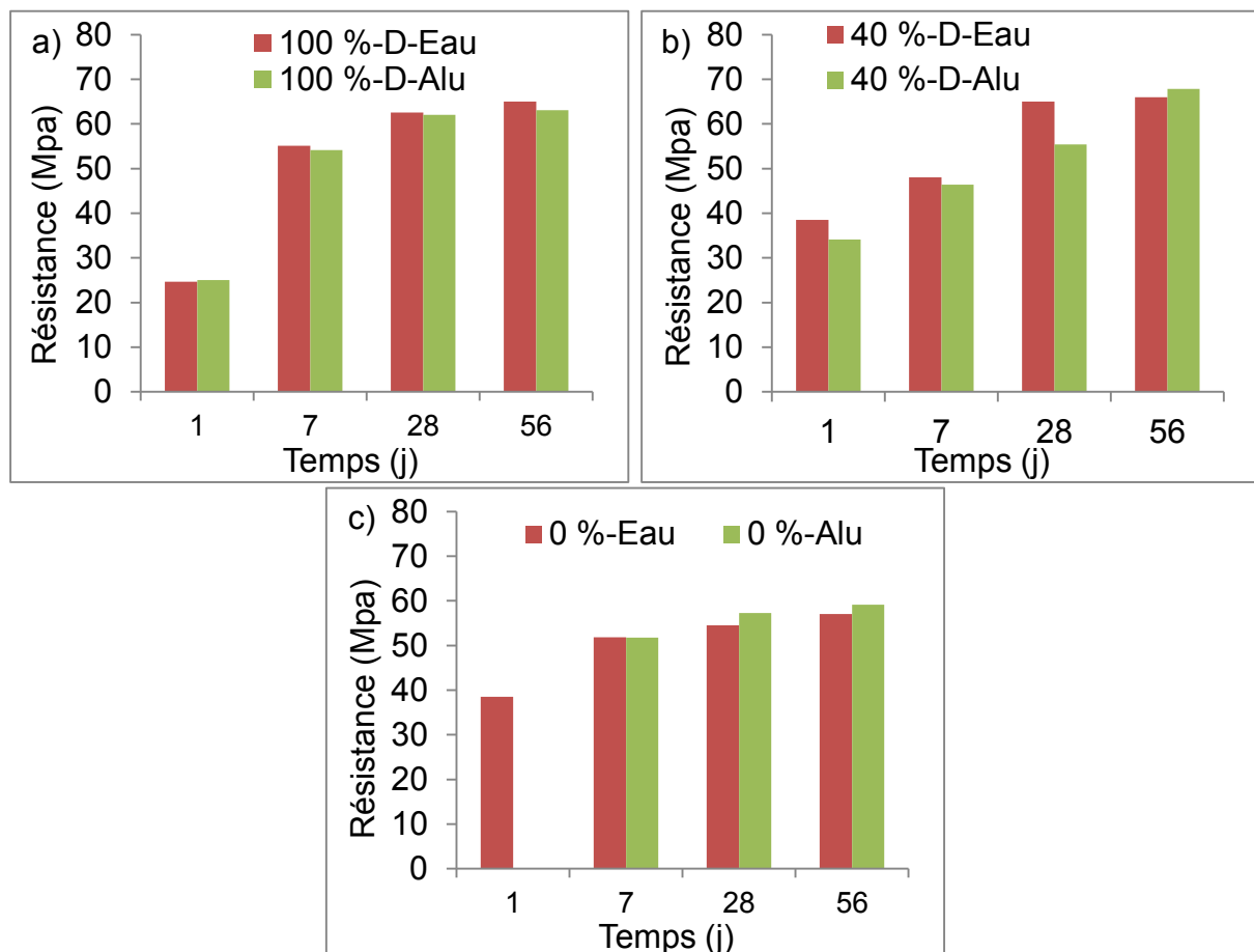
Figures 24. Résistance à la compression à 1, 7, 28 et 56 jours d'hydratation pour le ciment D (a), le mélange (b) des deux ciments (40 % de CEM I) et le ciment sulfoalumineux (c)
