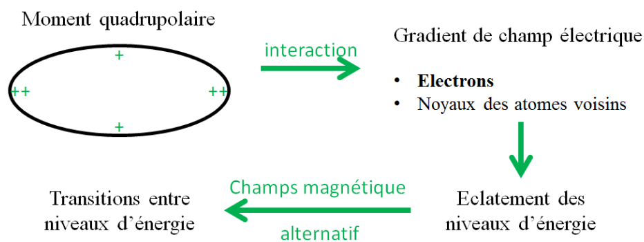
Figure 17: Principe de la RQN (extrait de [Ferrari, 2008])
