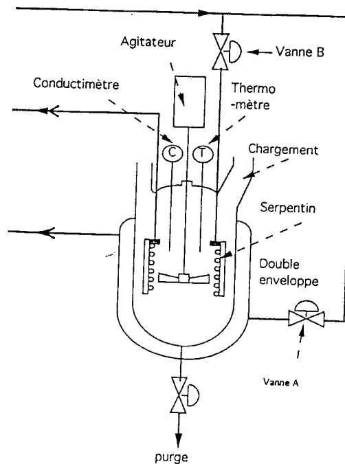
Figure II-1 : Cristalliseur détaillé.
