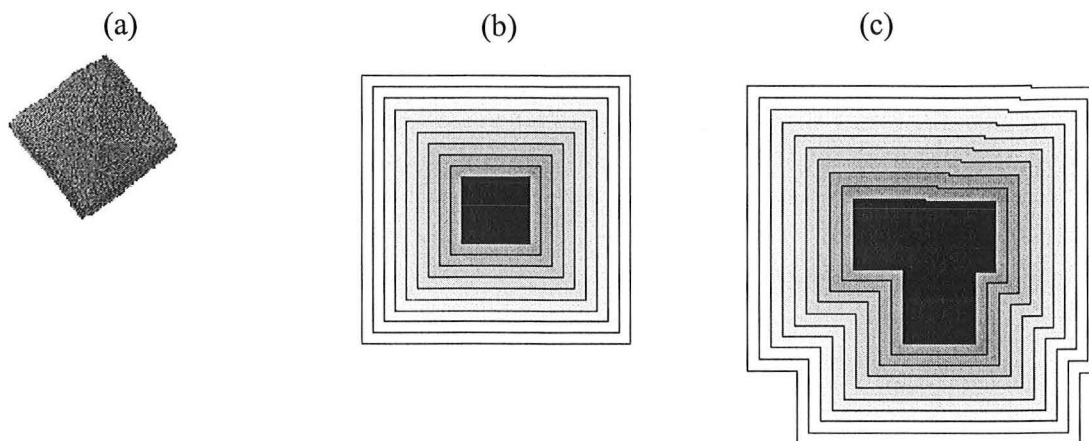
Figure I-13 : Croissance moléculaire par des dilations successives, (a) Monocrystal d'oxalate de calcium dihydrate, (b) croissance moléculaire du monocrystal, (c) croissance de l'agglomérat.
