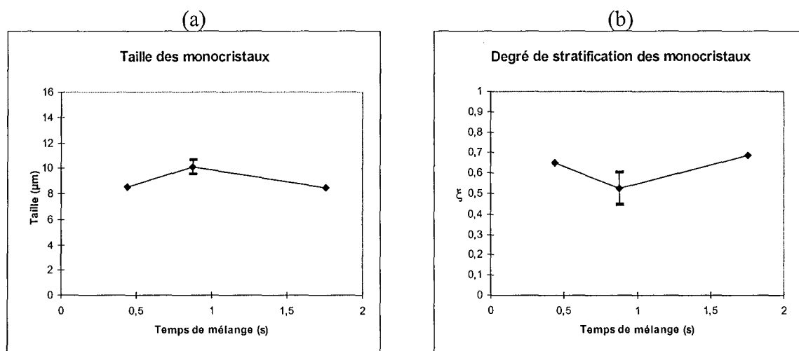
Figure II-21 : (a) Taille moyenne des monocristaux, (b) Stratification des monocristaux.
