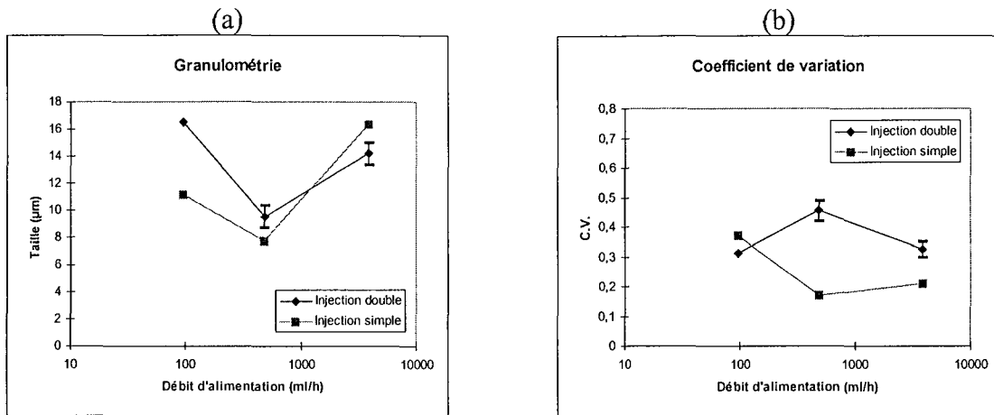
Figure II-15 : (a) Taille moyenne en nombre, (b) Coefficient de variation C.V.
