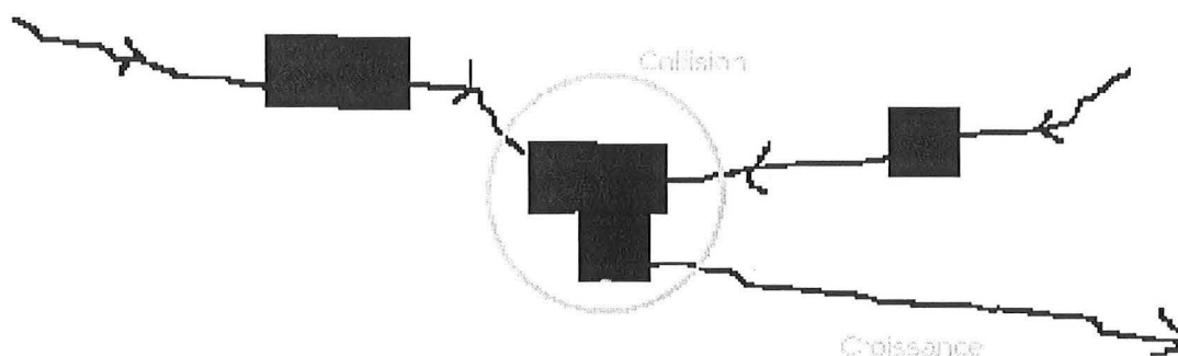
Figure I-14 : Collision d'un monocrystal et d'un agglomérat.
