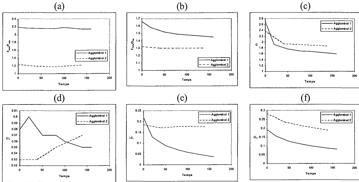
Figure I-19 : Evolution de la morphologie des deux agglomérats, (a) F_{\max}/F_{\min} , (b) F_{\max}/D_{eq} , (c) Circularité, (d) \Omega_1 , (e) I.C., (f) \Omega_2 .
