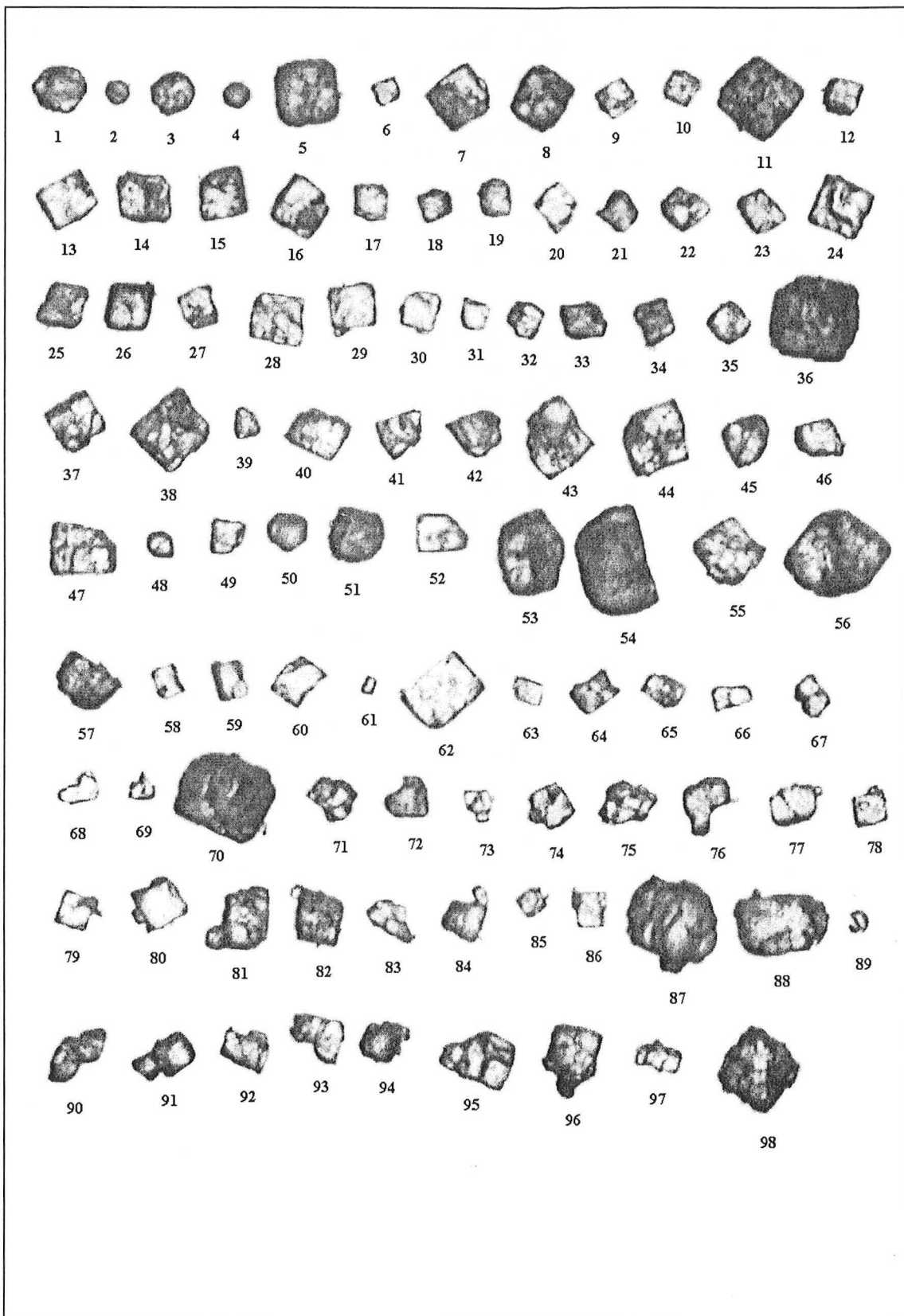
Figure III-5 : Population totale de 98 cristaux de KCl analysés par les deux méthodes d'analyses d'images.
