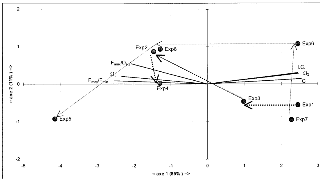
Figure III-4 : Morphologie moyenne en masse par ACP, (a) expériences du Tableau III-1, \rightarrow Q_a=5,7 l/h, \dots\rightarrow Q_a=10 l/h, (b) position des paramètres morphologiques.
