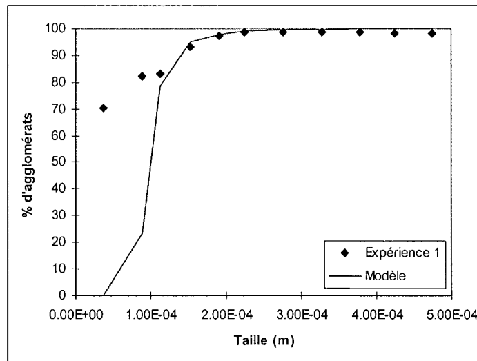
Figure III-16 : Confrontation du modèle mixte avec les résultats expérimentaux au niveau de l'évolution du pourcentage d'agglomérats pour l'expérience 1.
