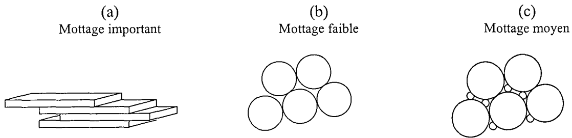
Figure I-2 : Exemples de surfaces de contact (a) plaques de même taille, (b) sphères de même tailles, (c) distribution bimodale de sphères.
