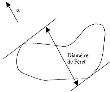
Figure I-16 : D efinition du diam etre de F eret
