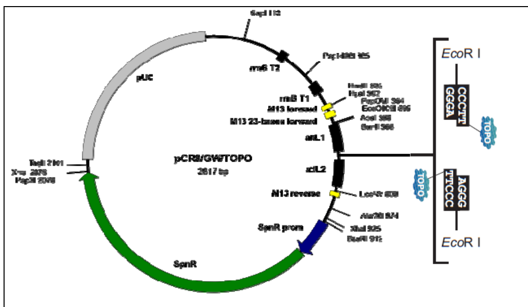
Figure 34 : Carte physique du plasmide pCR8 ® /GW/TOPO ®
