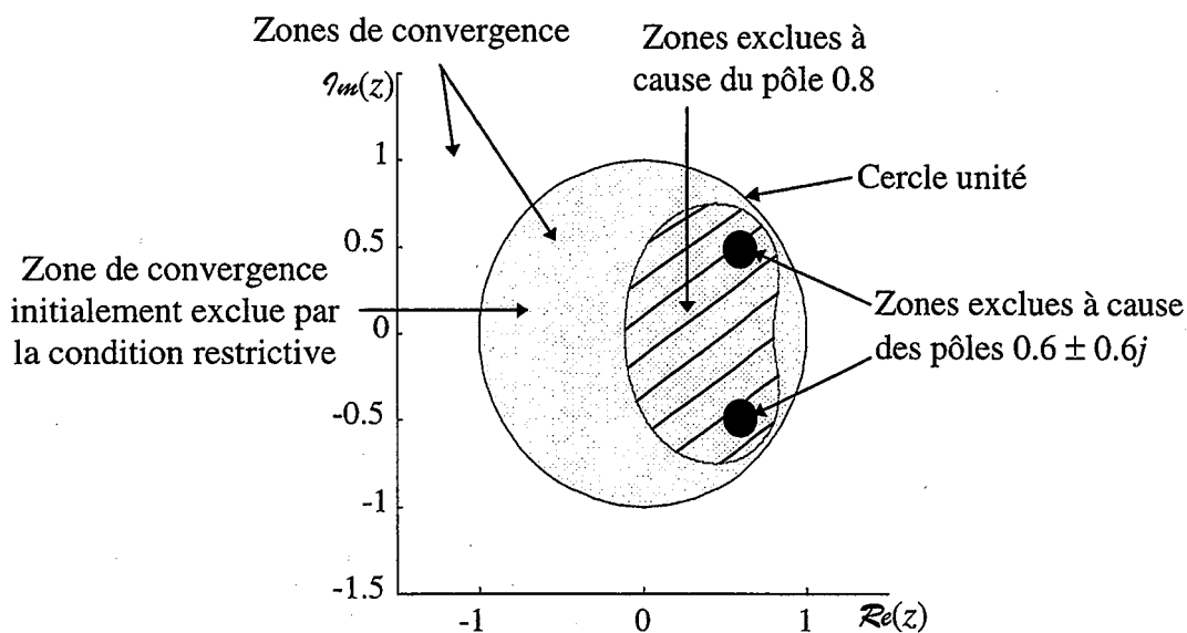
Figure II. 6 - Domaine de convergence de la série de Kautz sur le plan de la transformée en z
