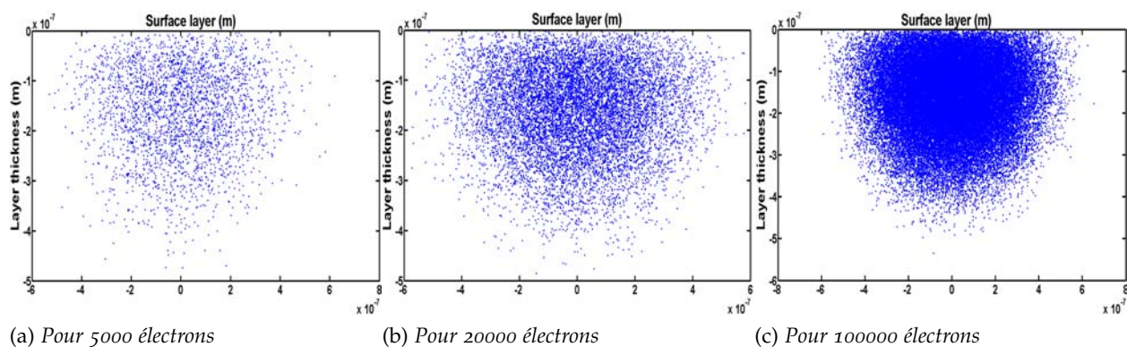
FIGURE 2.41 – Simulations de Monte-Carlo des positions de fins de parcours des électrons dans le matériau GaN, obtenues pour une tension d'accélération de E = 10\text{keV} (les électrons rétrodiffusés ne sont pas représentés) et un nombre d'électrons pris en compte différent.
