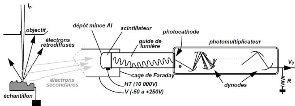
FIGURE 2.12 – Schéma de principe du détecteur d'Everhart-Thornley
