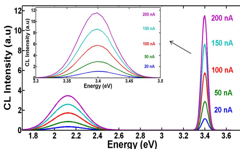
FIGURE 2.35 – Spectres de CL simulés d'un substrat GaN épais pour différents courants du faisceau électronique
