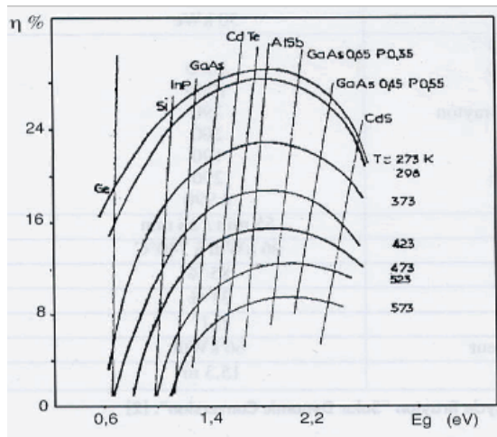
FIGURE A.4 – Rendement de conversion en fonction de l'énergie de gap E_g et de la température pour différents semi-conducteurs.
